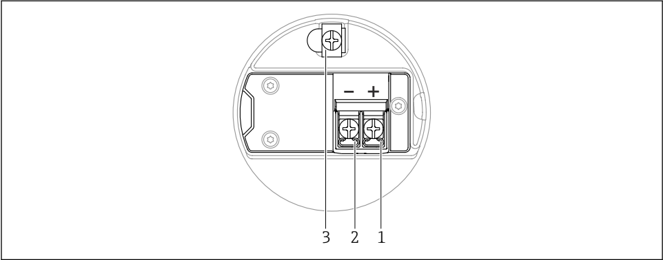
图 7 接线腔中的接线端子和接地端
