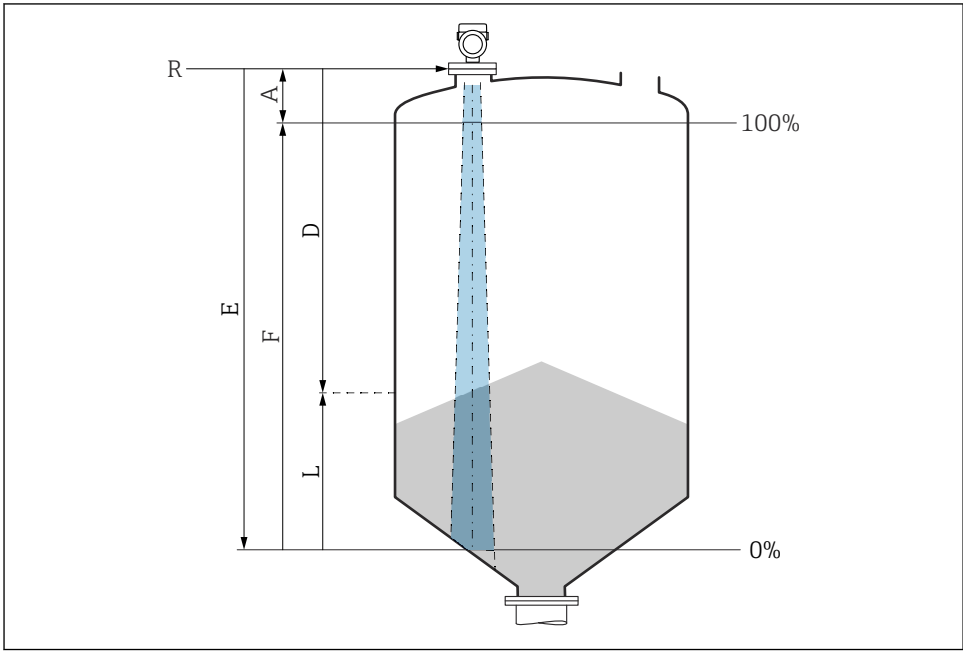
图 16 固体散料料位测量的设置参数
