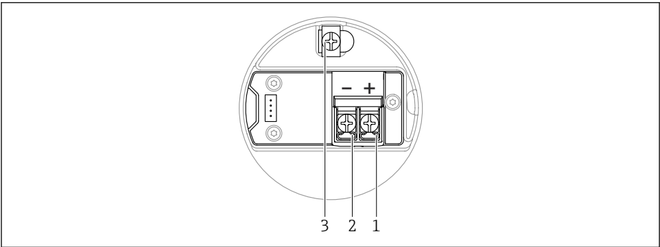
图 8 接线腔中的接线端子和接地端
