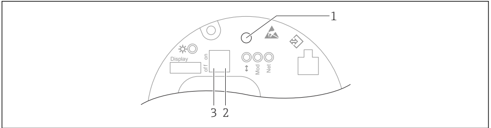
图 9 Ethernet-APL 电子插件上的操作按键和 DIP 开关
