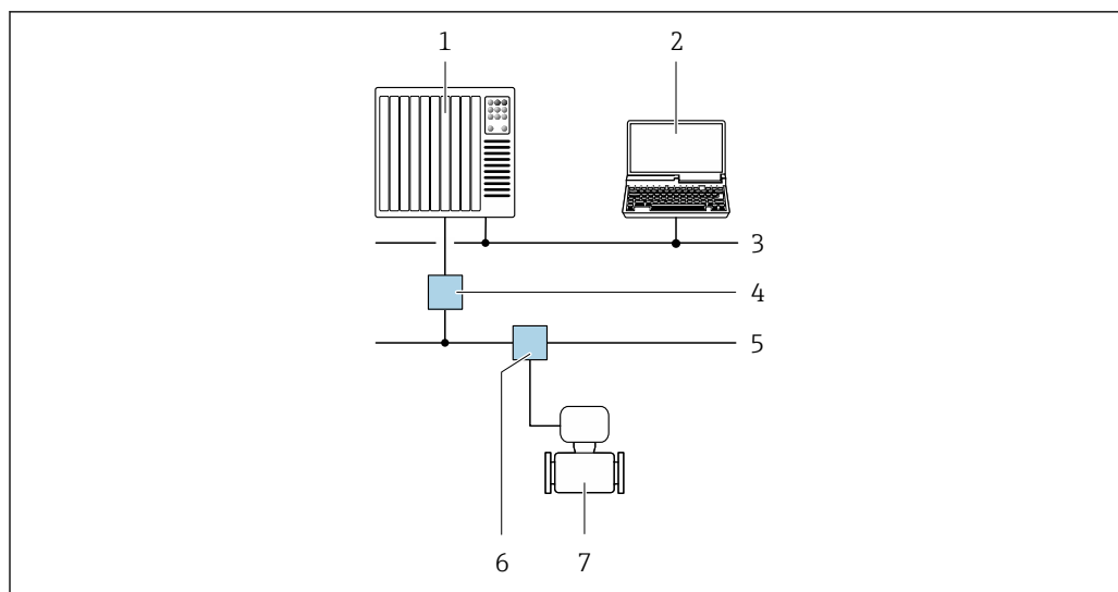
24 Варианты дистанционного управления по сети PROFIBUS PA
