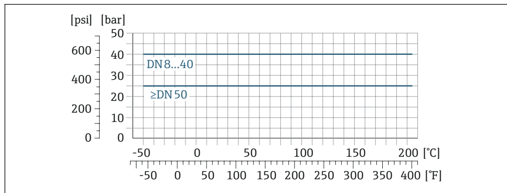
图 21 法兰材质: 1.4435 (316L)
