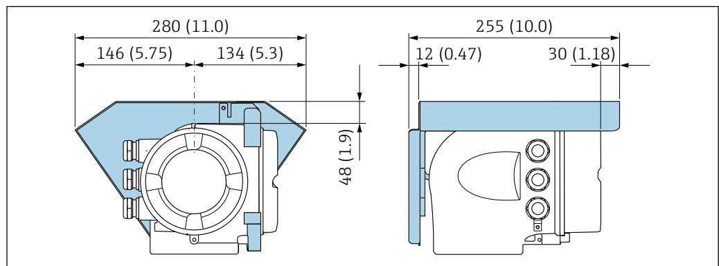
15 单位: mm (in)
