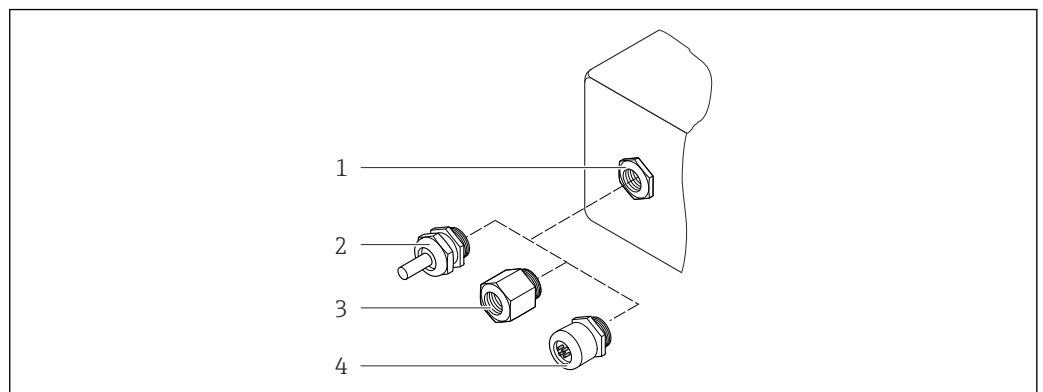
图 39 允许的电缆入口/缆塞
