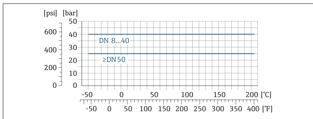
图 22 连接部件材质: 1.4435 (316L)
