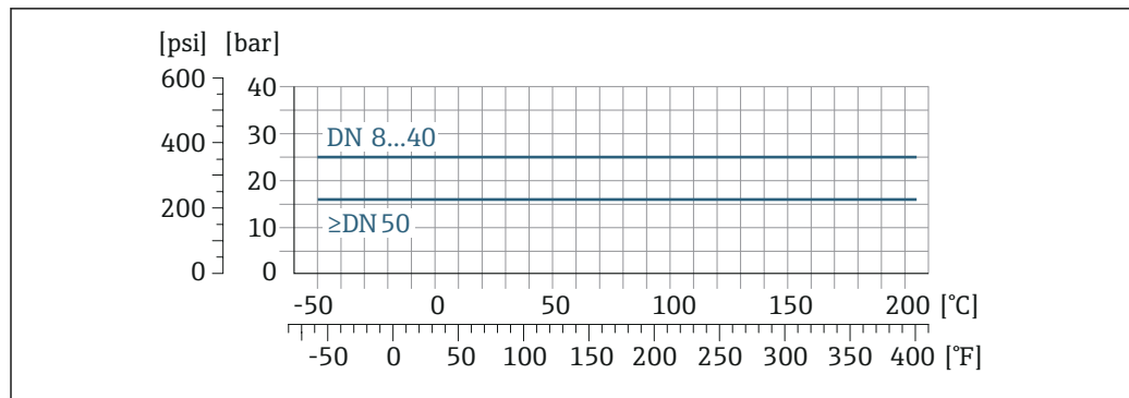
图 20 法兰材质: 1.4435 (316L)
