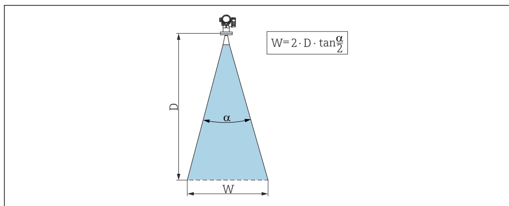
19 Zależność między kątem wiązki \alpha , odległością D a średnicą wiązki W
