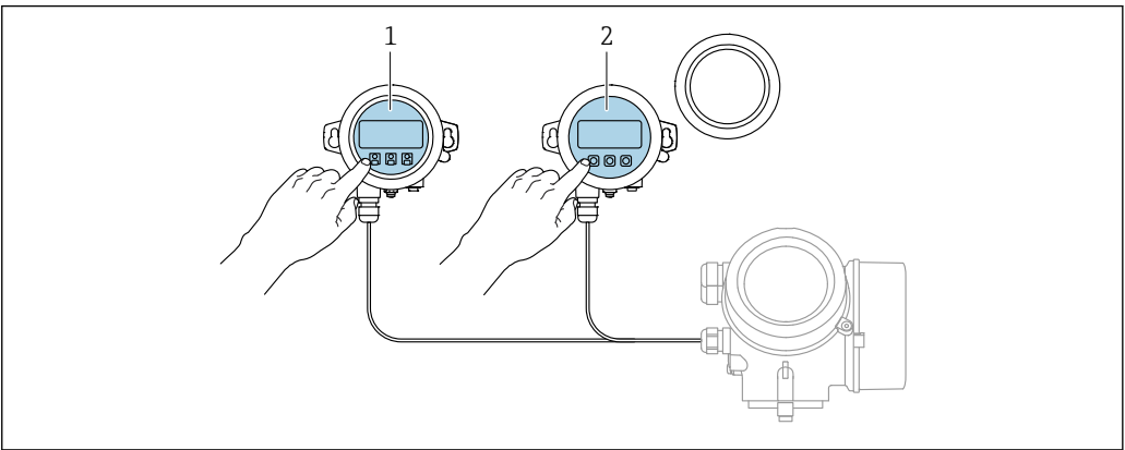
39 Warianty obsługi za pomocą zewnętrznego wskaźnika FHX50
