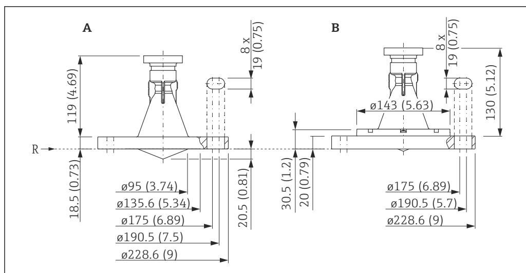
34 Wymiary FMR56 z kołnierzem przesuwным 4"/DN100. Jednostka miary mm (in)
