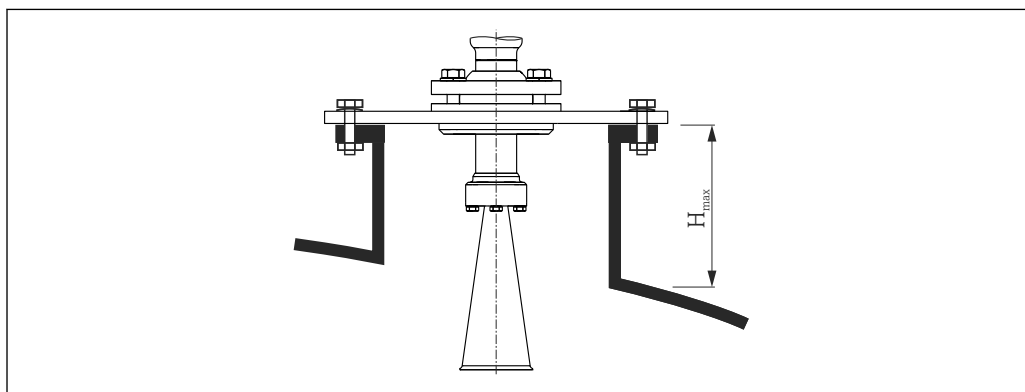
22 Wysokość króćca montażowego dla anteny stożkowej (FMR57)
