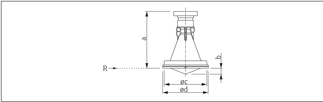
31 Wymiary FMR56 bez przyłącza procesowego. Jednostka miary mm (in)
