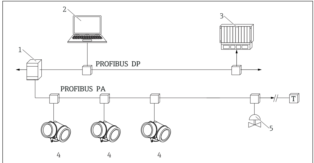
43 Opcje obsługi zdalnej z wykorzystaniem protokołu PROFIBUS PA
