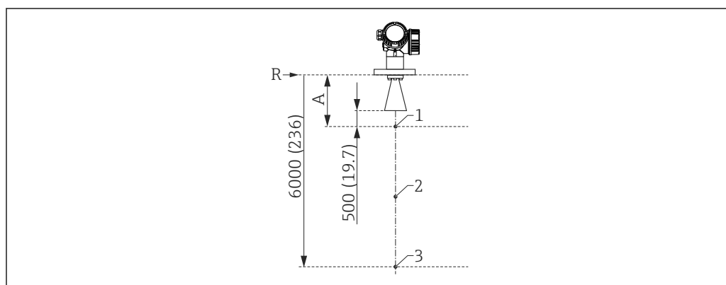
48 Punkty 3-punktowego protokołu linearyzacji; wymiary w mm (calach)
