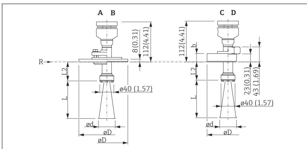
36 Wymiary FMR57 z anteną stożkową - wersja standardowa. Jednostka miary mm (in)
