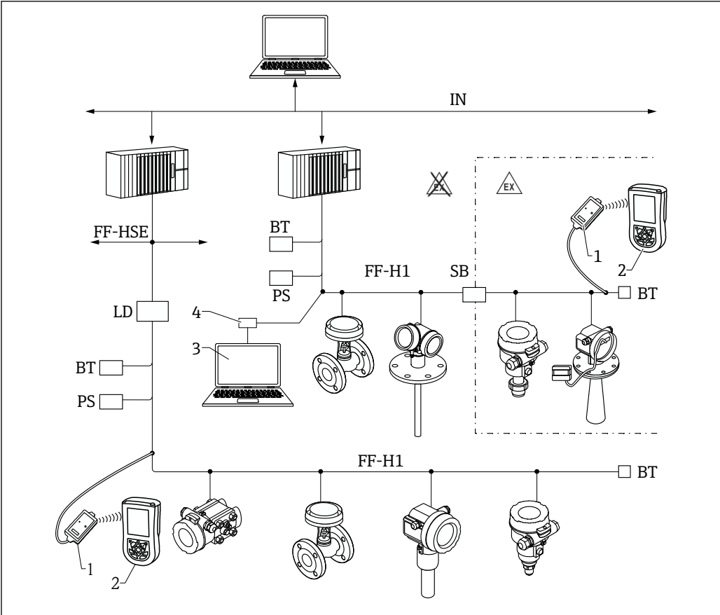
44 Architektura systemu FOUNDATION Fieldbus i elementy składowe
