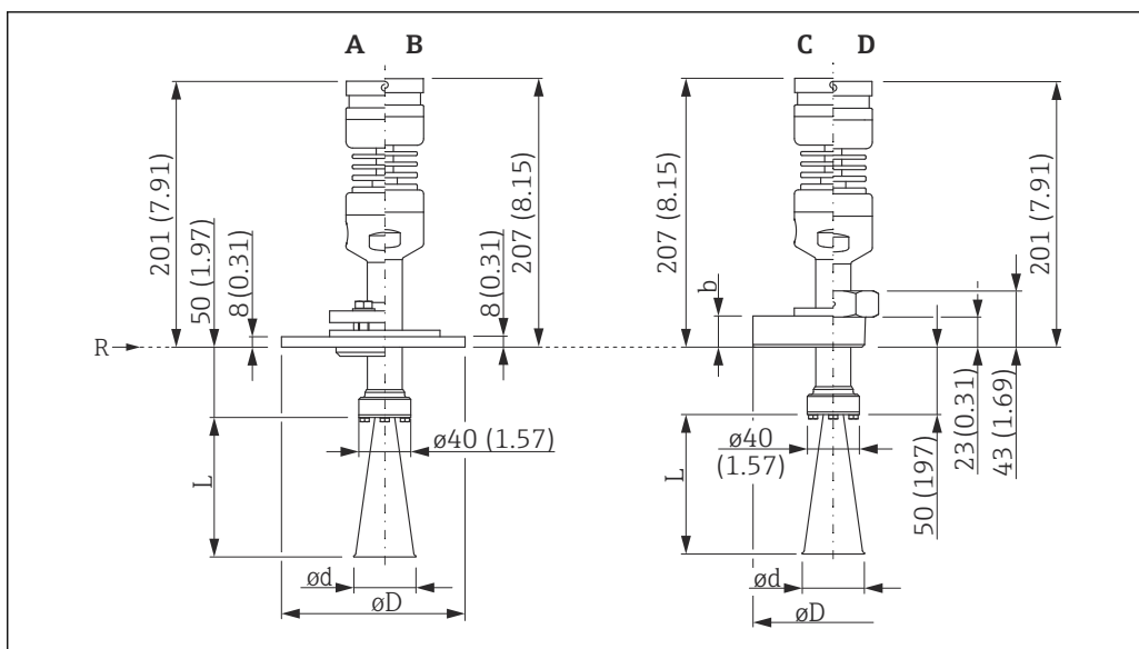
37 Wymiary FMR57 z anteną stożkową - wersja wysokotemperaturowa; wymiary w mm(calach)
