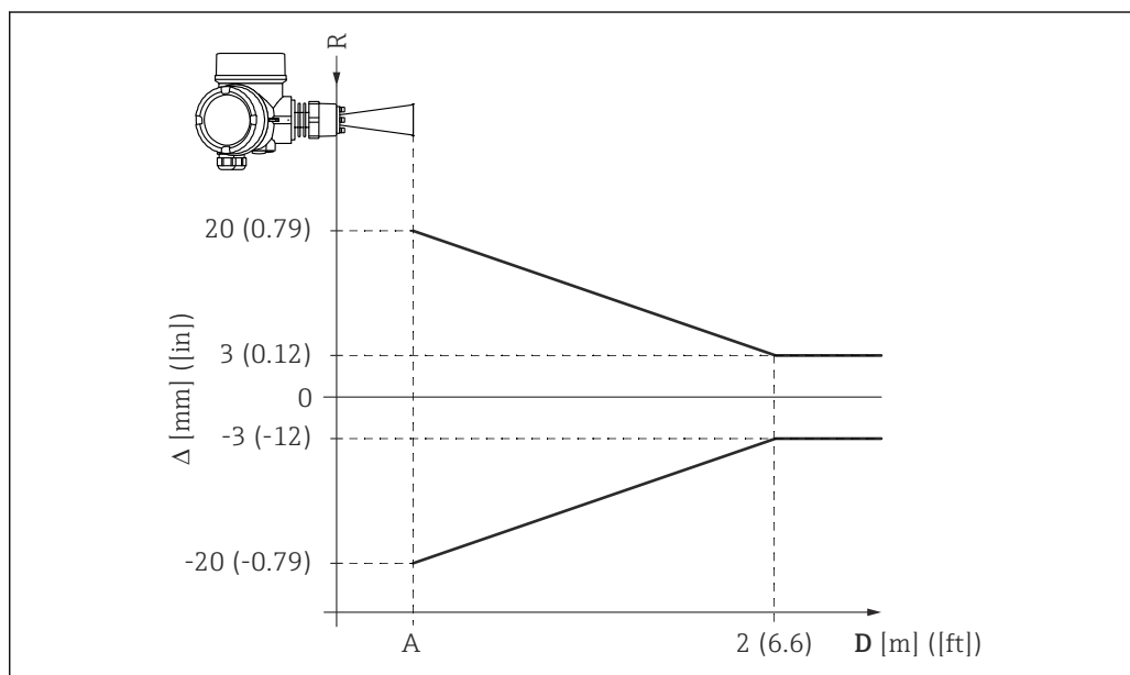
18 Maksymalny błąd pomiaru dla małej rozpiętości zakresu pomiarowego
