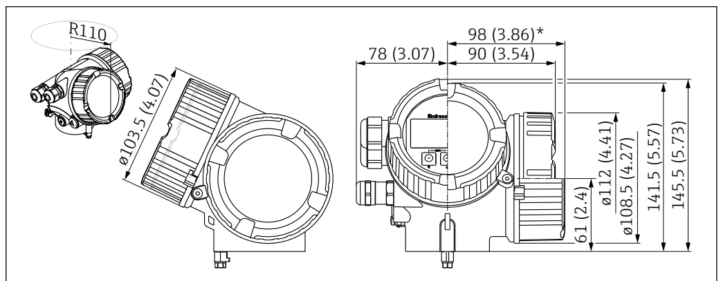
■ 30 Obudowa GT20 (aluminium malowane proszkowo). Jednostka miary mm (in)
