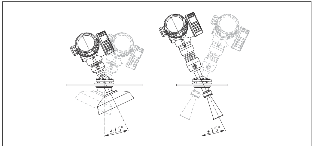
24 Micropilot FMR57 z pozycjonerem anteny
