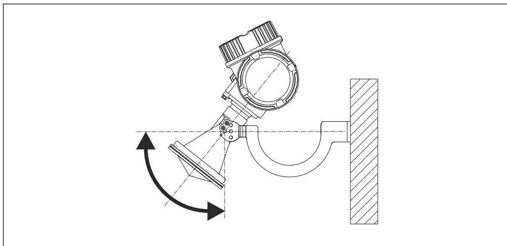
21 Montaż anteny stożkowej z uchwytem montażowym
