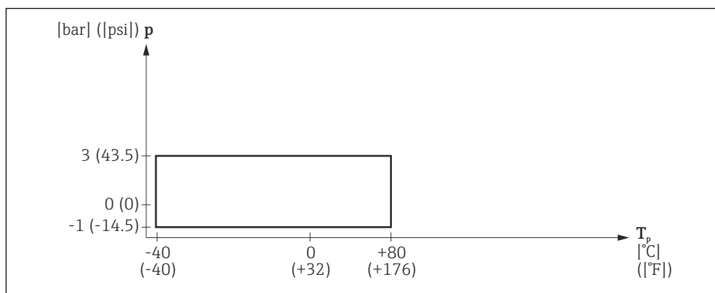
26 FMR56: Dopuszczalny zakres temperatury i ciśnienia medium
