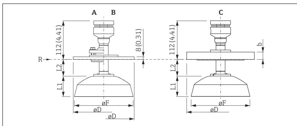
38 Wymiary FMR57 z anteną paraboliczną; wymiary w mm (calach)
