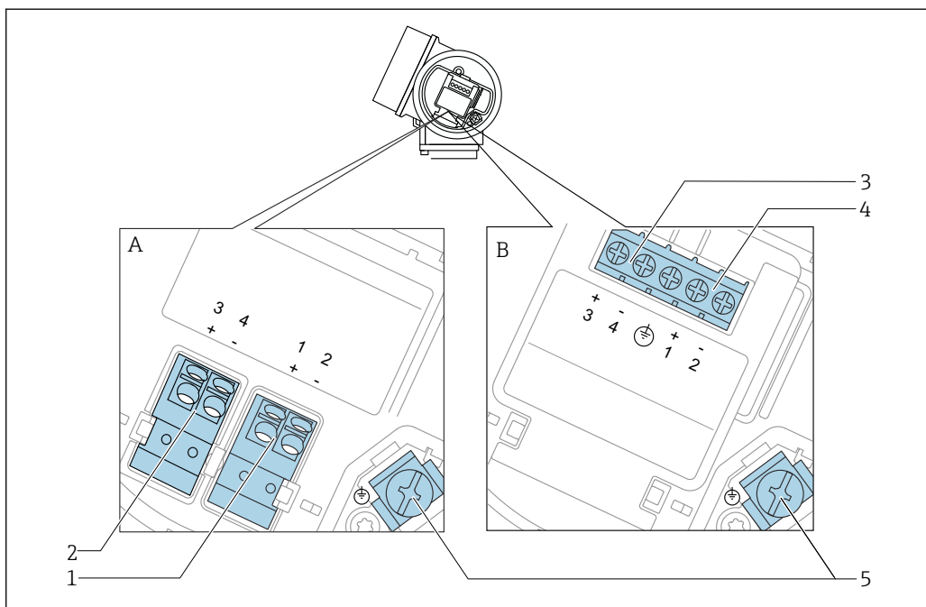
12 Przyporządkowanie zacisków dla wersji PROFIBUS PA / FOUNDATION Fieldbus
