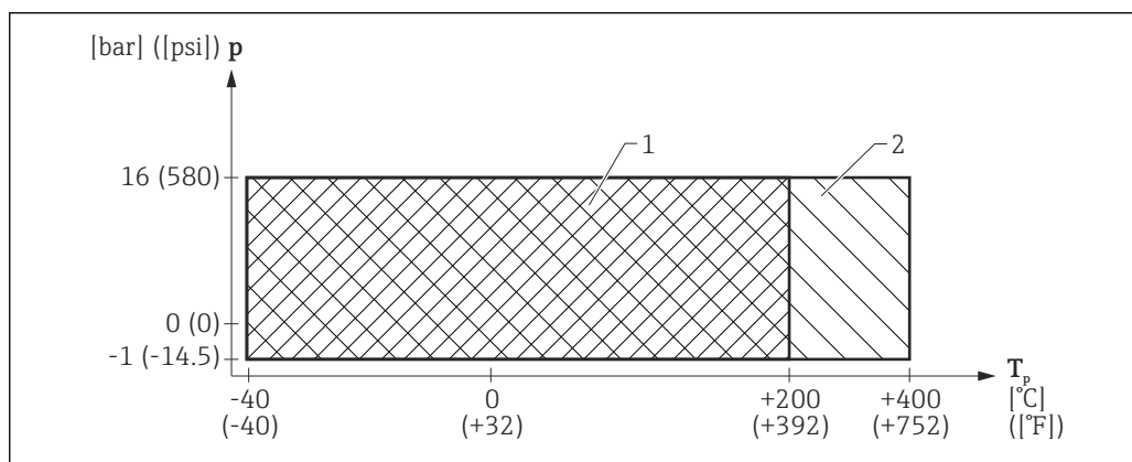
27 FMR57: Dopuszczalny zakres temperatury i ciśnienia medium
