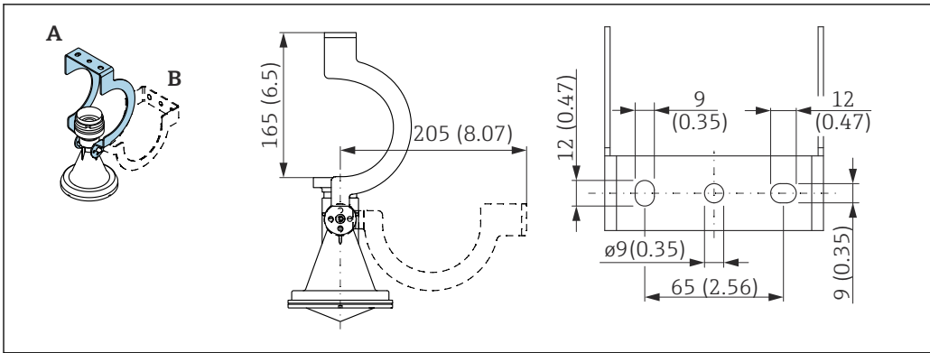
32 Wymiary uchwyty montażowego. Jednostka miary mm (in)
