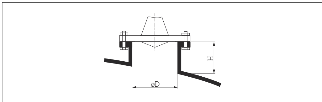
20 Wysokość króćca i średnica anteny stożkowej z kołnierzem przesuwным
