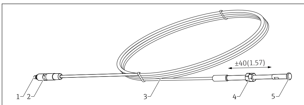
11 Extension de câble
