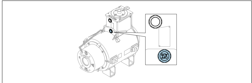
39 Fenêtres du mécanisme de fermeture
