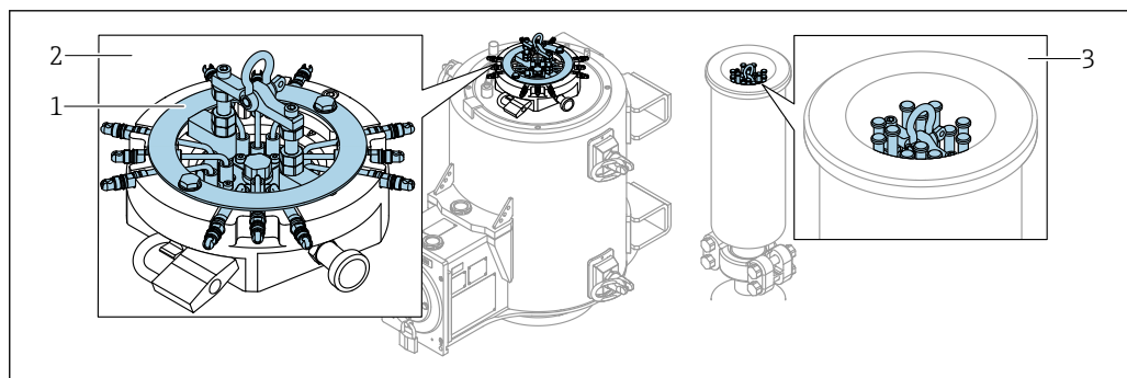
36 Magasin de sources et porte-source
