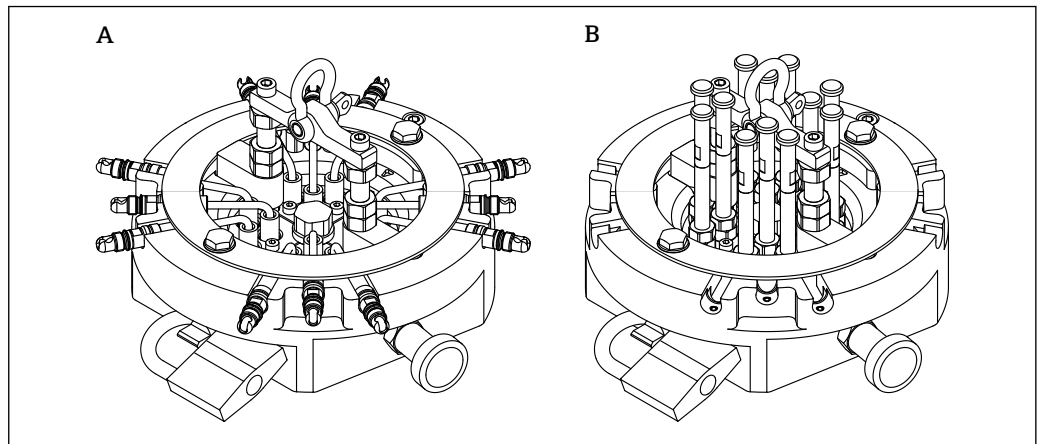
7 Anneau de fixation avec 12 sources radioactives abaissables (magasin de sources pas encore abaissé)
