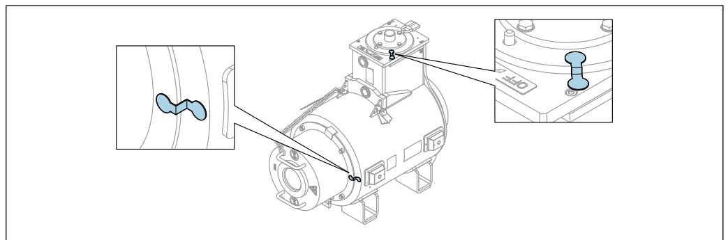
42 Scellés de sécurité sur le conteneur de source
