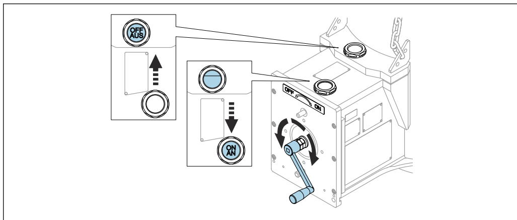
37 Contrôle du fonctionnement du mécanisme de fermeture
