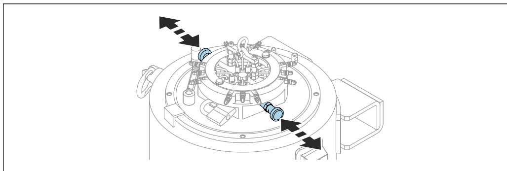
38 Contrôle du fonctionnement des boulons de verrouillage
