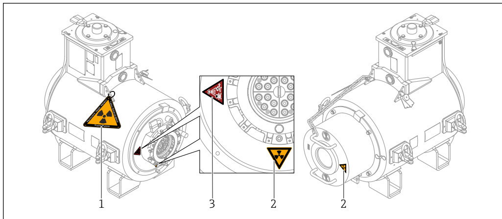
10 Position des panneaux d'avertissement contre le rayonnement
