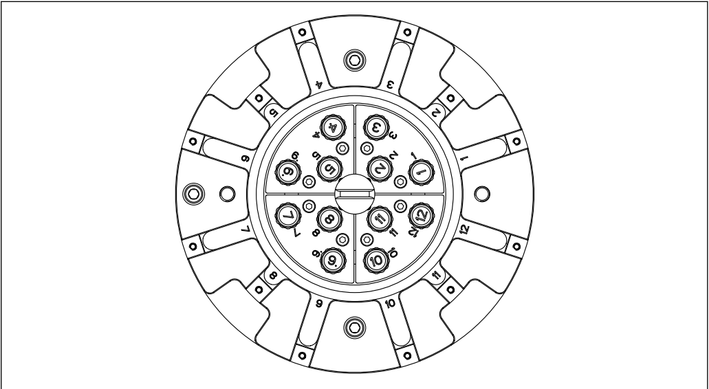
29 Aperçu du chargement, magasin de sources (12 positions)
