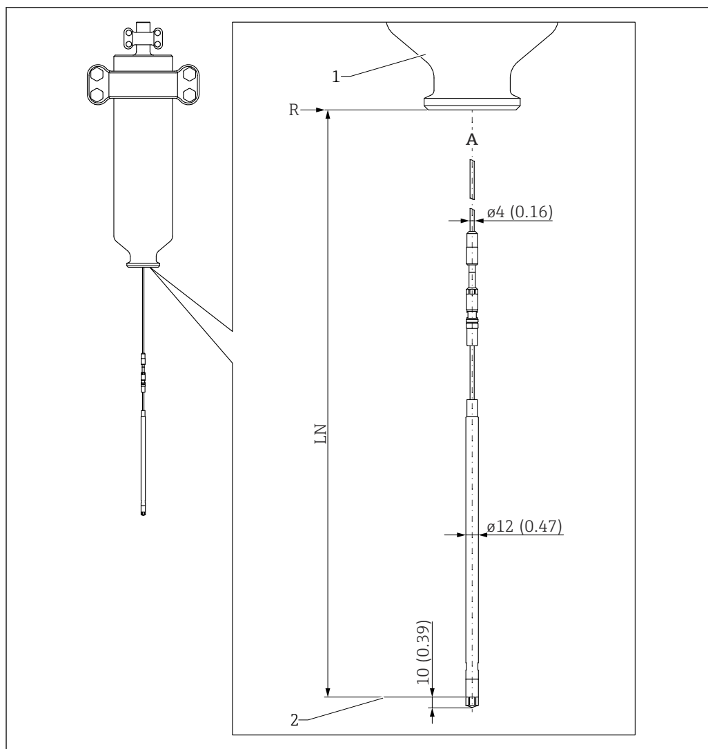
8 Version rigide, conçue pour les tubes de protection droits
