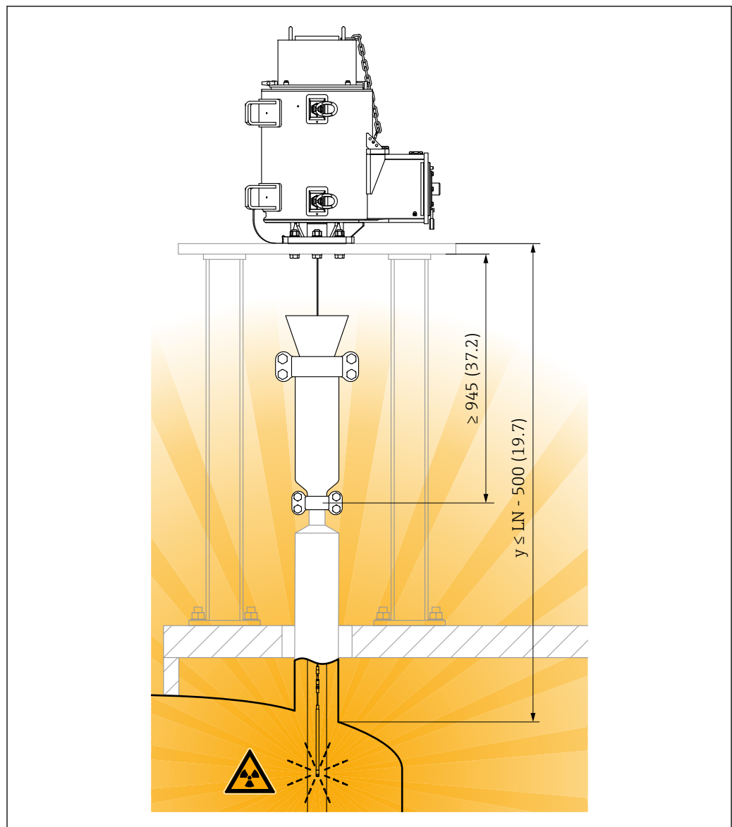
26 Dimensions de montage
