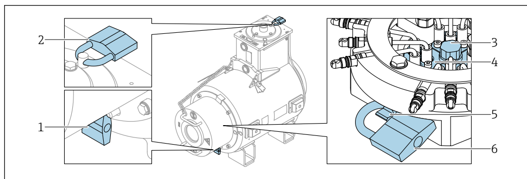
35 Composants de la protection antivol
