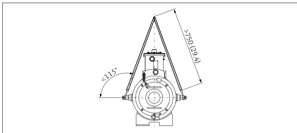
24 Angle de câble (< 115°) et longueur de câble (> 1500 mm (59 in)). Unité de mesure mm (in)
