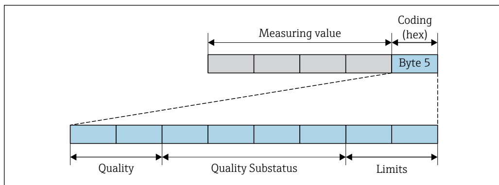
37 Estrutura do byte de codificação
