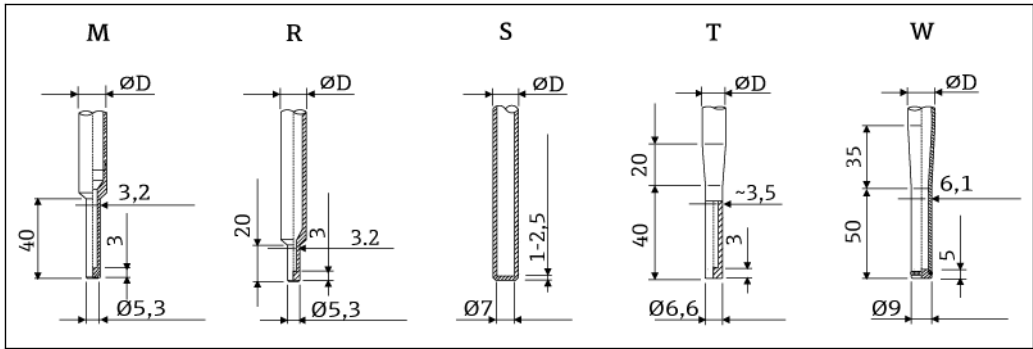
5 Доступные варианты наконечников термогильзы (усеченный, прямой и суженный) Максимальная шероховатость поверхности Ra ≤ 0,8 мкм
