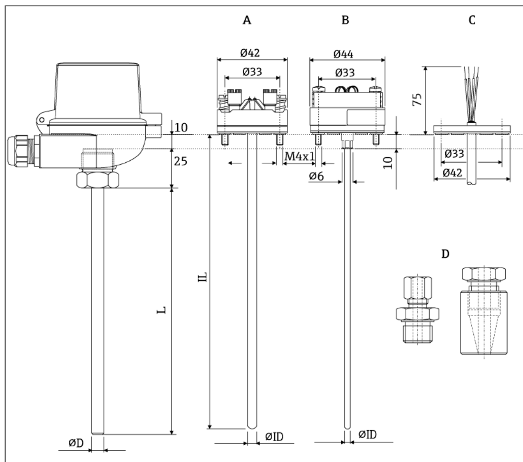
4 Размеры TR12 и TC12
