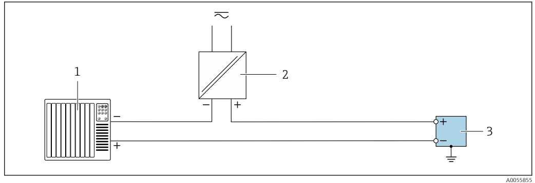
25 Exemple de raccordement pour sortie impulsion / sortie fréquence / sortie tout ou rien (passive)
