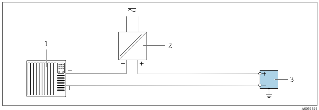
26 Exemple de raccordement pour sortie relais
