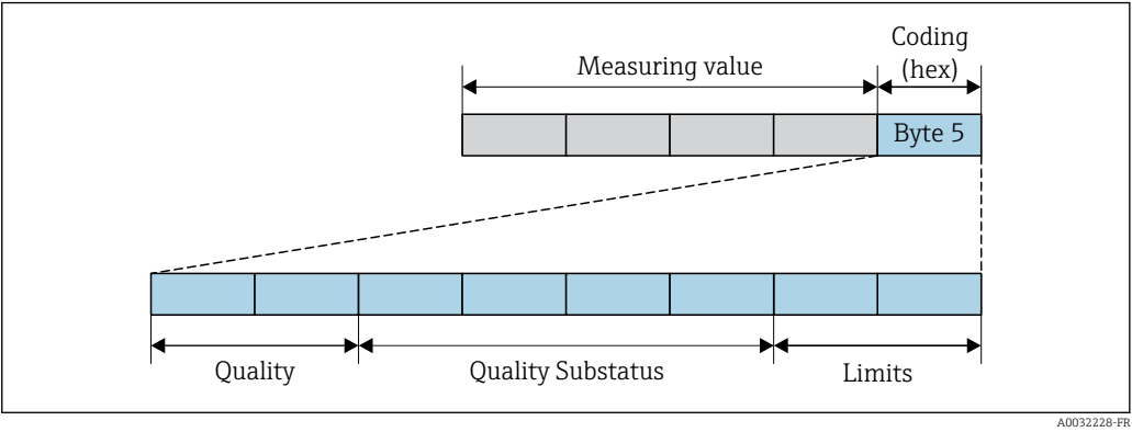
41 Structure de l'octet de codage
