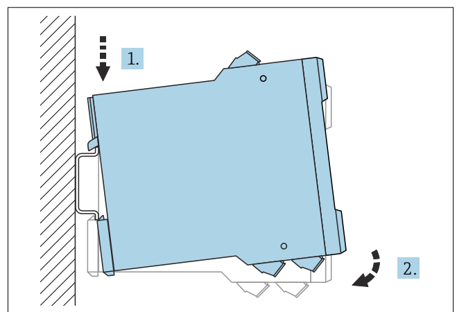
1 Montieren; Hutschiene gemäß EN 60715 TH35-7.5/EN 60715 TH35-15
