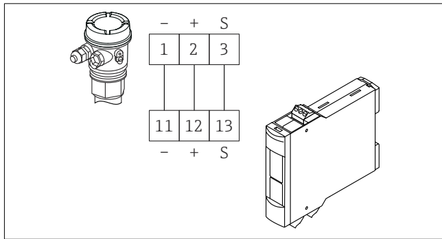
2 Anschluss der Spannungsversorgung und Signalleitung S mit beliebigem Messaufnehmer
