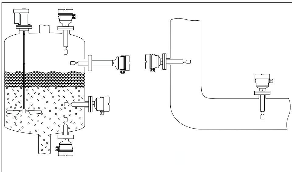
2 Примеры монтажа в резервуаре, баке или трубопроводе
