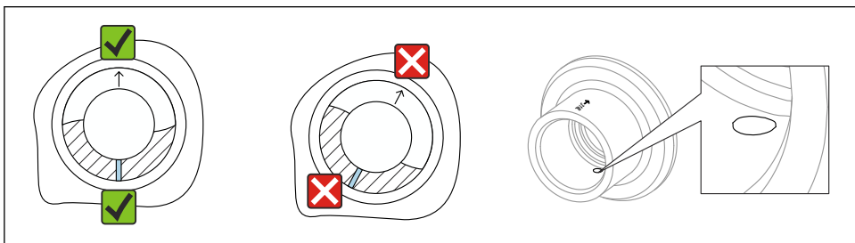
10 Сварной переходник с отверстием для утечек
