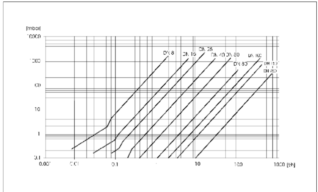
水的系统压损
