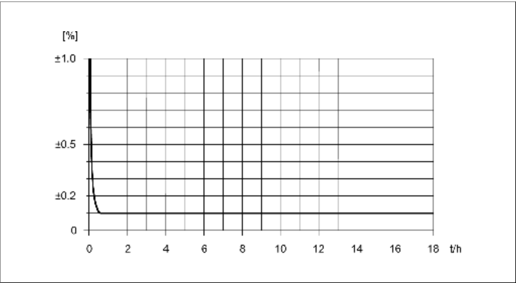
仪表的最大测量误差(%读数值)(以Promass 83F/DN25为例)
