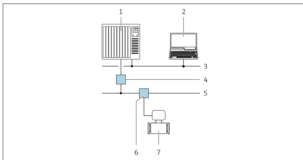
14 Варианты дистанционного управления по сети PROFIBUS PA
