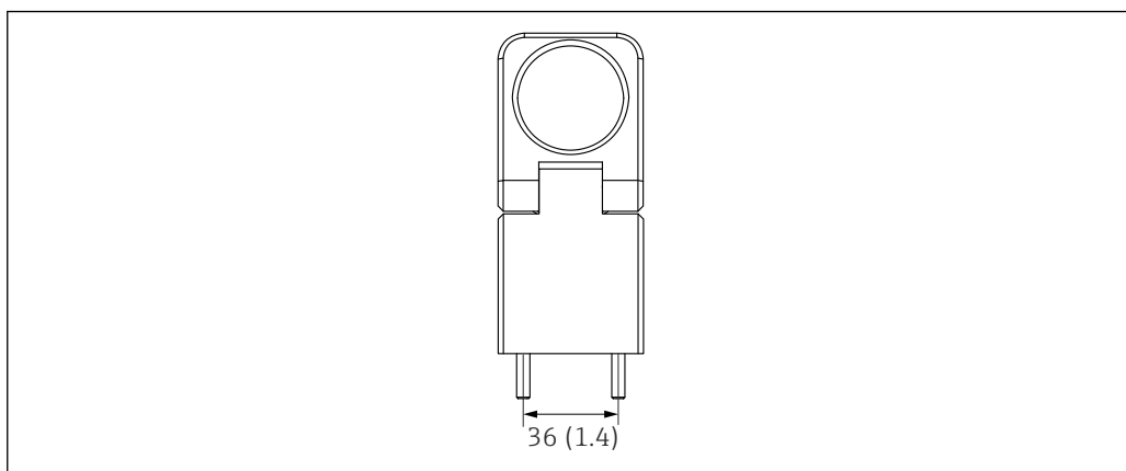
6 Mål for ringklemme med mellemstykke. Teknisk enhed: mm (")
