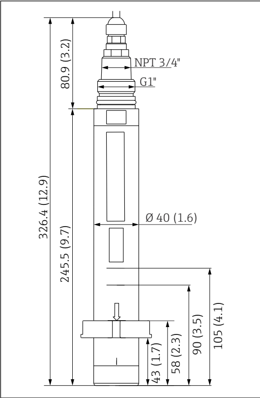
3 Sensorens mål inklusive fastgørelsesring. Enhed: mm (tommer)
