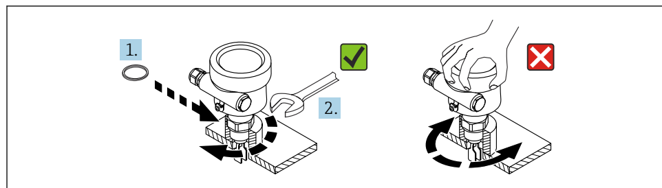
図 13 機器のネジ止め
