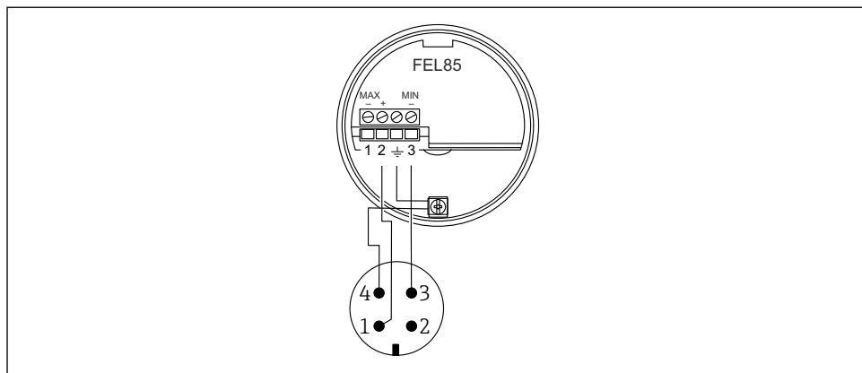
図 16 M12 コネクタを使用した端子の割当て、MIN 動作モード
