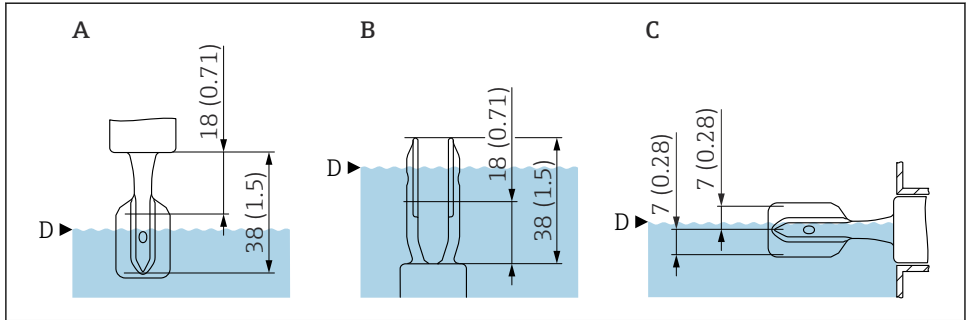
4 標準的なスイッチポイント
