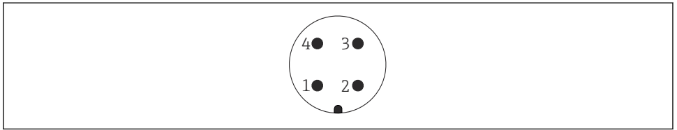
図 14 M12 プラグ、ピンの割当て
