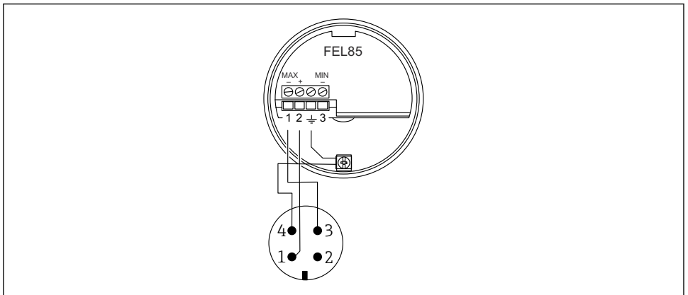
図 15 M12 コネクタを使用した端子の割当て、MAX 動作モード
