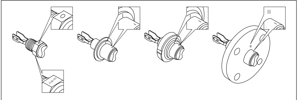
図 11 マークを使用して容器に水平に取り付ける場合の音叉部の位置
