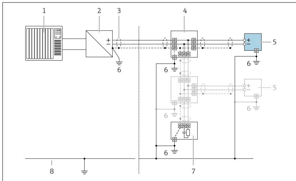
25 Ejemplo de conexión de FOUNDATION Fieldbus
