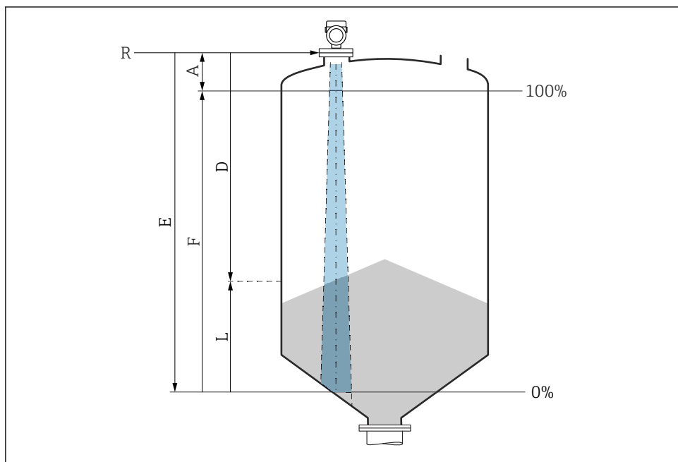
11 Configuratieparameters voor niveaumeting in stortgoederen
