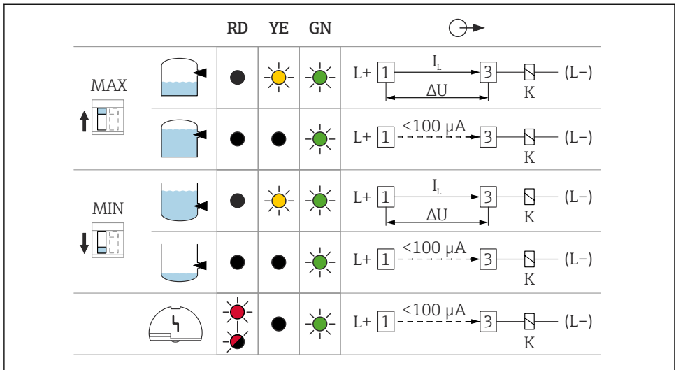
18 Azione dell'uscita di commutazione e segnalazione, inserto elettronico FEL62
