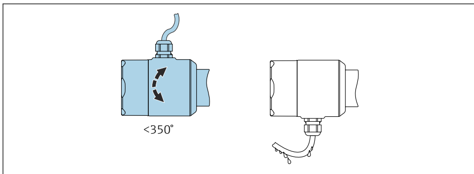
11 Custodia senza vite di fermo; formare un anello salvagoccia sul cavo.
