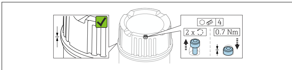
13 Coperchio con vite di fissaggio
