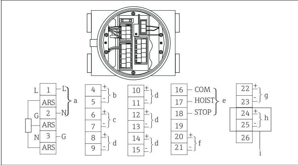
37 Bornes du NMS5
