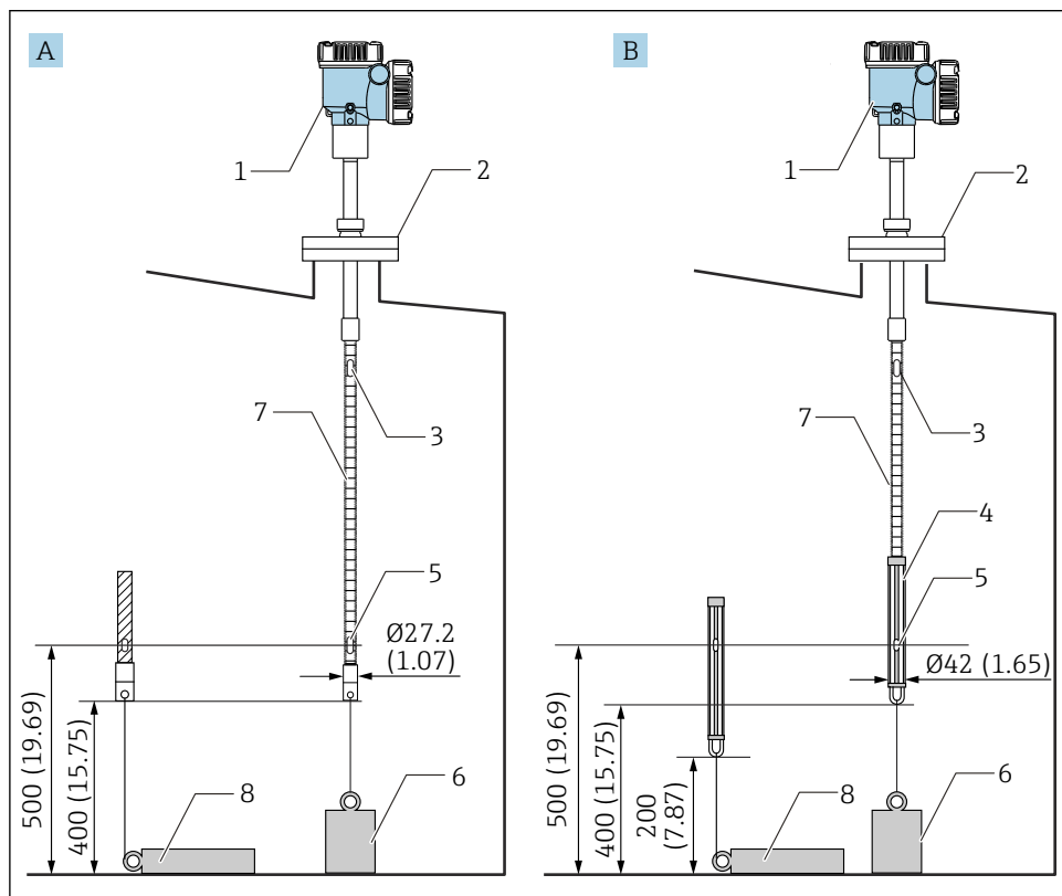
28 Méthode du poids d'ancrage. Unité de mesure mm (in)
