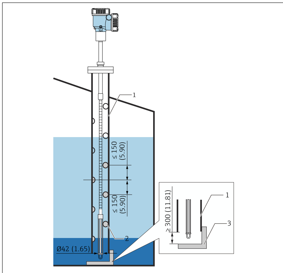
☛ 27 Tube de mesure. Unité de mesure mm (in)
