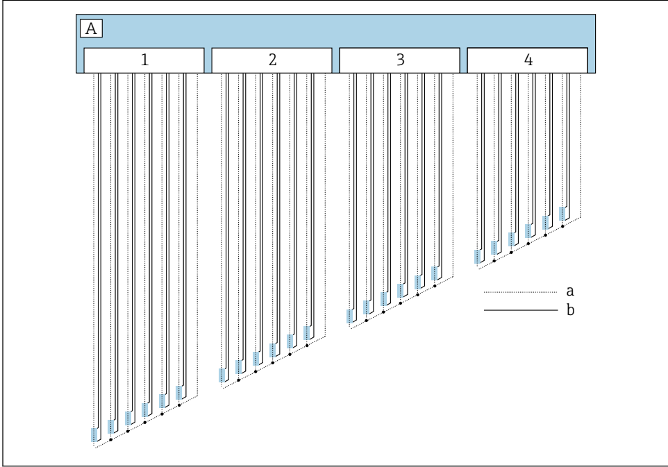
35 Schéma de raccordement à 4 fils
