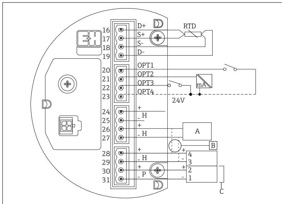
38 Bornes (à sécurité intrinsèque) du NRF590
