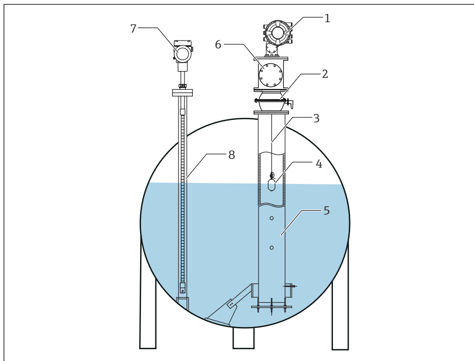
32 Protecteur pour une cuve sous pression
