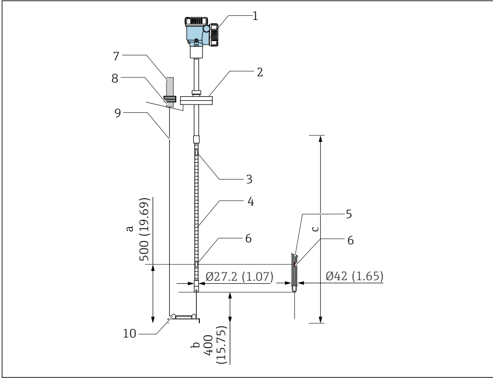
24 Méthode de l'ancrage supérieur. Unité de mesure mm (in)
