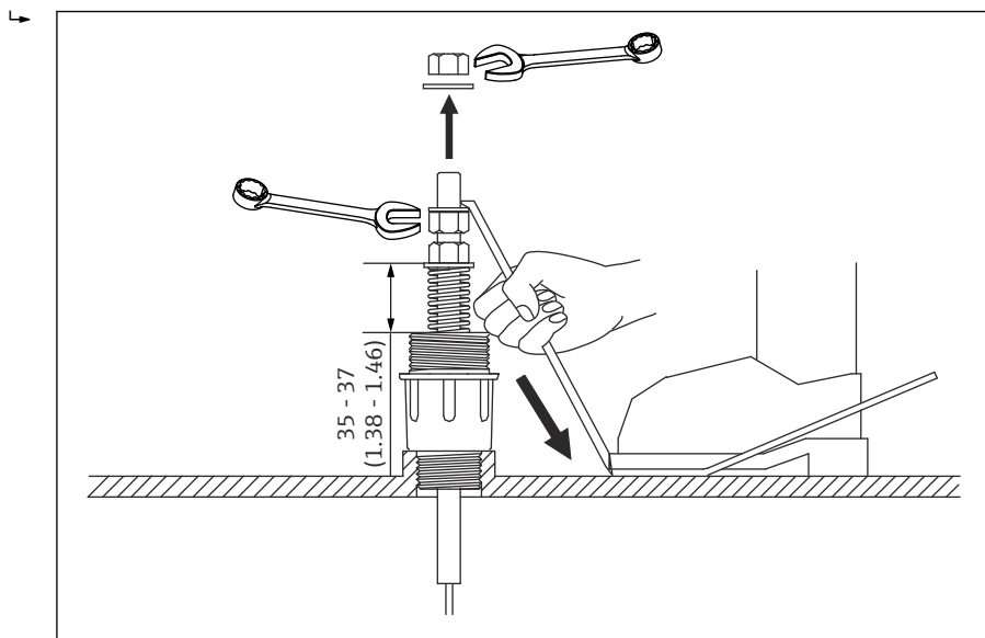
26 Montage d'un ancrage supérieur 2. Unité de mesure mm (in)
