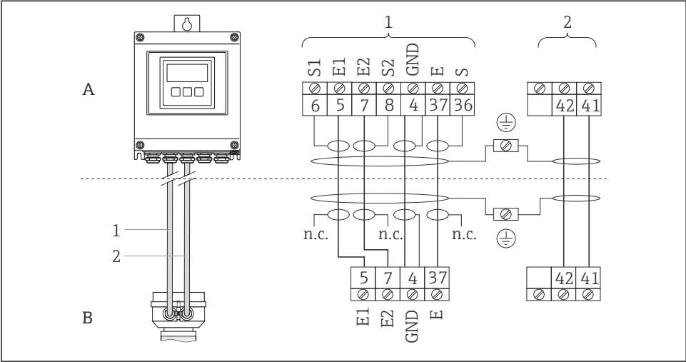
5 Asignación de terminales en la versión separada
