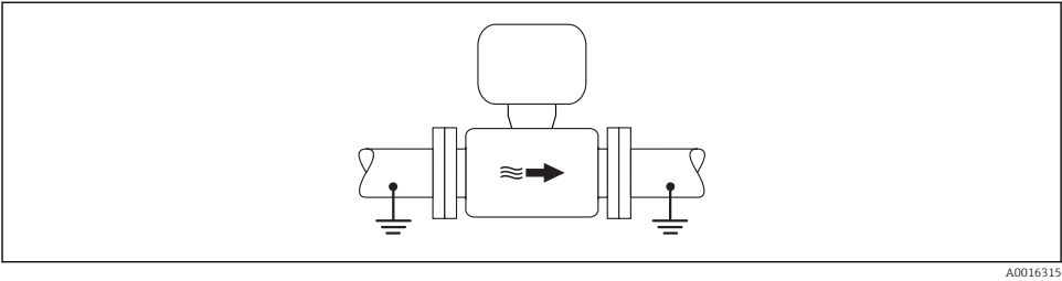
10 Igualación de potencial a través del tubo de medición
