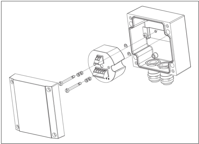
图 1 安装
