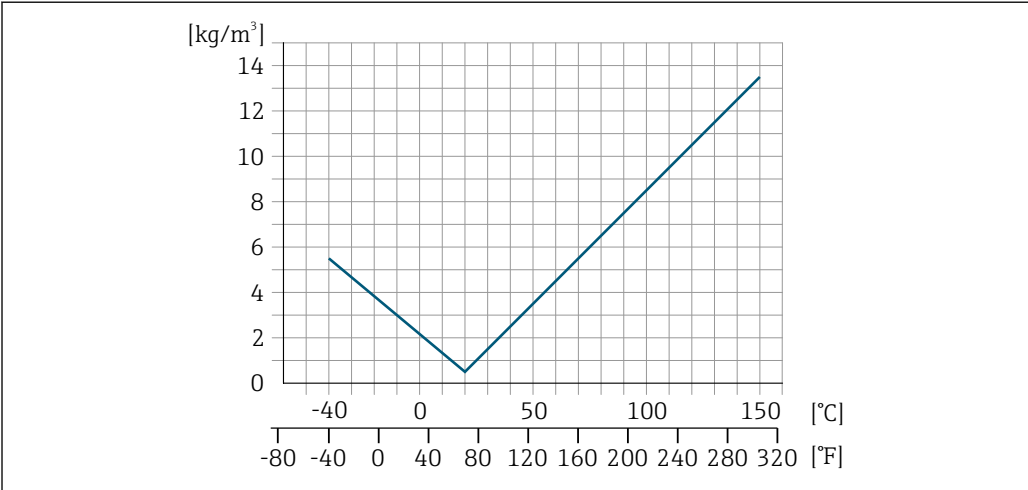
図 45 現場密度調整、例：+20 °C (+68 °F) 時
