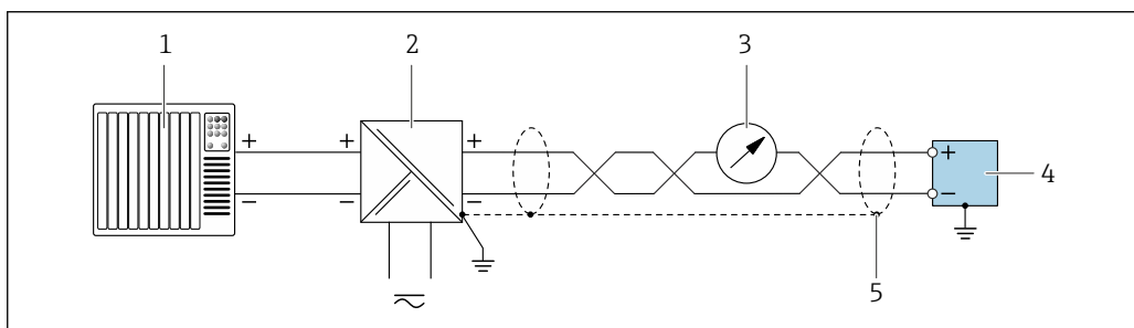
図 27 4～20 mA 電流出力（パッシブ）、HART 搭載の接続例
