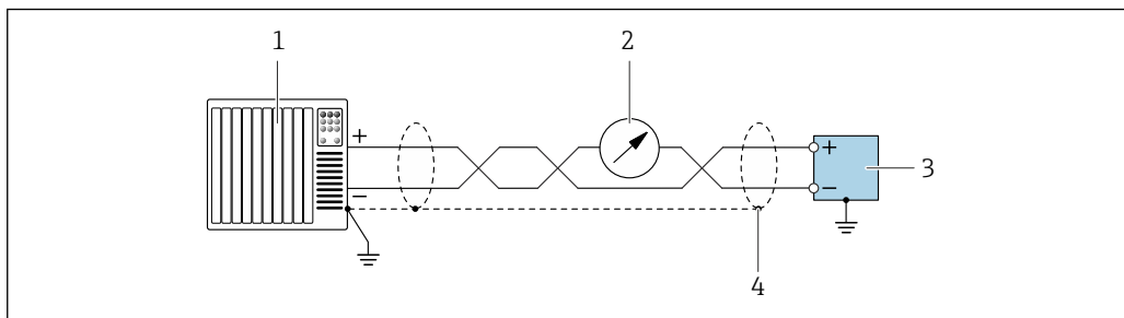
図 26 4～20 mA 電流出力（アクティブ）、HART 搭載の接続例
