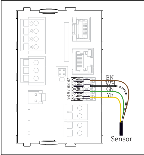
11 추가 공급 전압이 없는 센서
