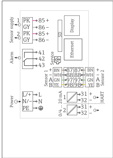
7 BASE2-H 또는 -L의 예를 사용한 전체 배선도
