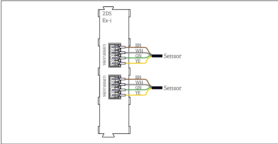
📌 14 센서 통신 모듈 타입 2DS Ex-i에 추가 공급 전압이 없는 센서
