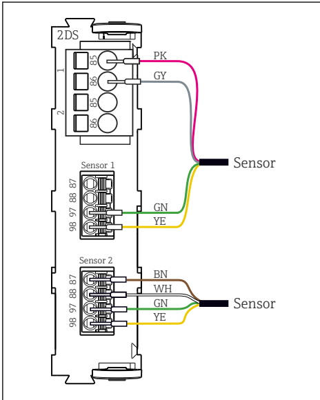
13 센서 모듈 2DS에서 추가 공급 전압이 있거나 없는 센서
