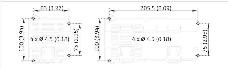
☐ 2 벽 설치 시 드릴링 패턴 mm (in)
