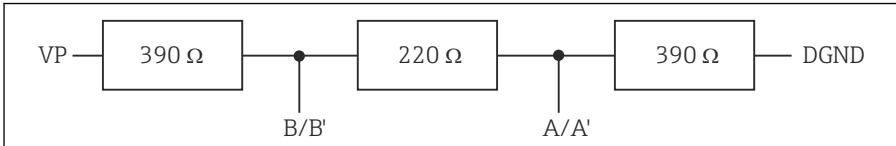
☞ 32 내부 종단의 구조
