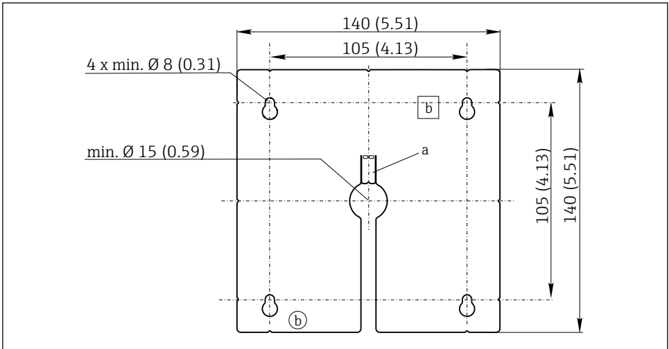
3 외부 디스플레이 설치 플레이트, 치수 mm (in)
