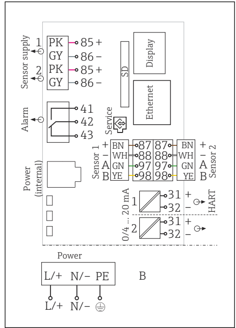
9 BASE2-E 및 외부 전원 공급 장치(B)의 예를 사용한 전체 배선도
