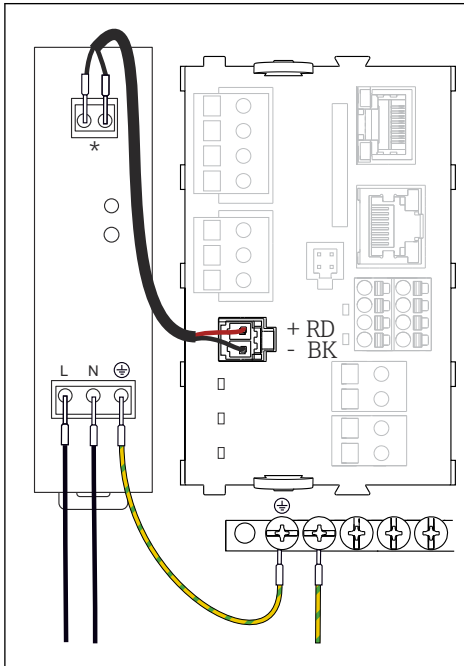
8 BASE2-E의 예를 사용한 전원 공급 장치 연결
