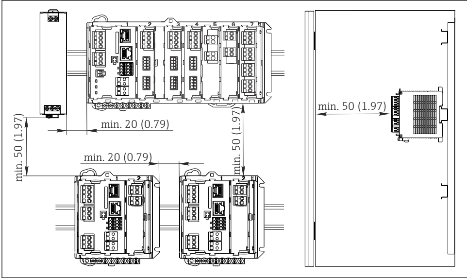
☐ 1 최소 간격 mm (in)
