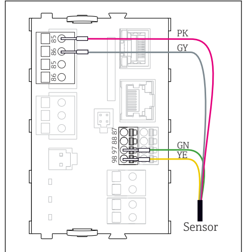
12 추가 공급 전압이 있는 센서
