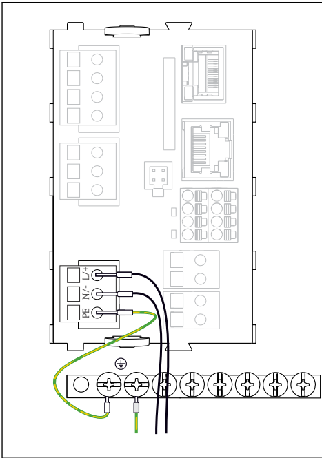
6 BASE2-H 또는 -L의 예를 사용한 전원 공급 장치 연결
