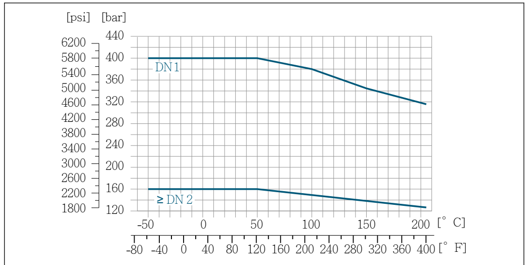
19 Attacco 4-VCO-4: 1.4539 (904L); attacco 8-VCO-4: 1.4539 (904L); adattatore filettato NPTF: 1.4539 (904L)
