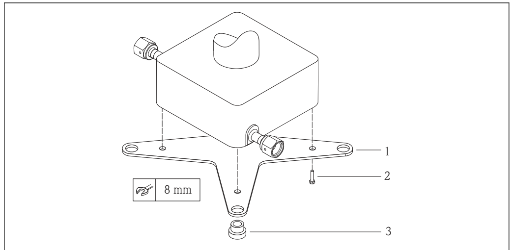
13 Kit di montaggio per piastra di montaggio per Cubemass
