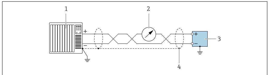
10 Esempio di collegamento all'uscita in corrente a 4 ... 20 mA con HART (attiva)
