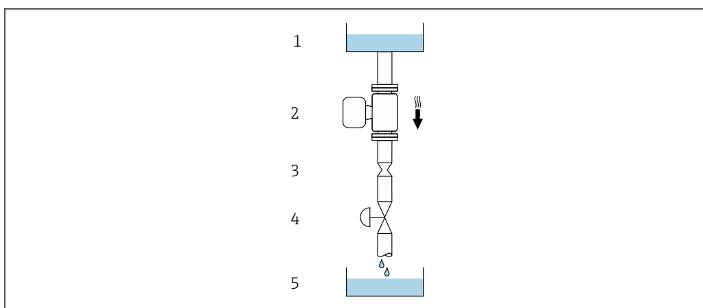
12 Installazione in un tubo a scarico libero (ad es. per applicazioni di dosaggio)
