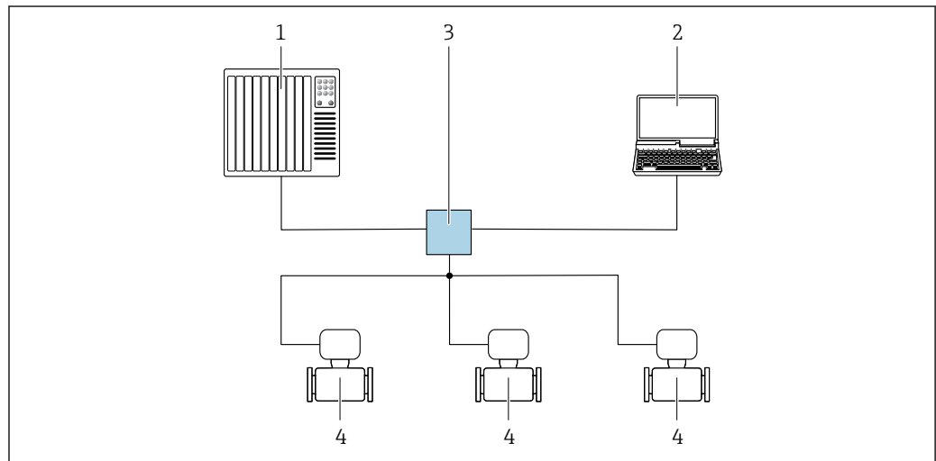
31 Opzioni per il funzionamento a distanza mediante rete PROFINET: topologia a stella
