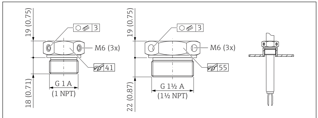
40 Casquillos deslizantes para la operación sin presión p_e = 0 bar (0 psi). Unidad de medida mm (in)
