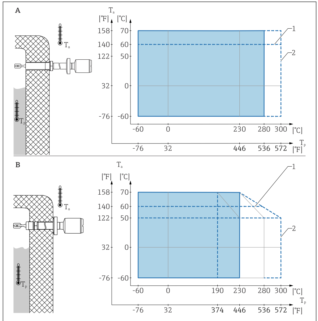
23 Temperatura ambiente admisible T_a en la caja en función de la temperatura de proceso T_p en el depósito; temperatura máxima del proceso 230 °C (446 °F) o 280 °C (536 °F)
