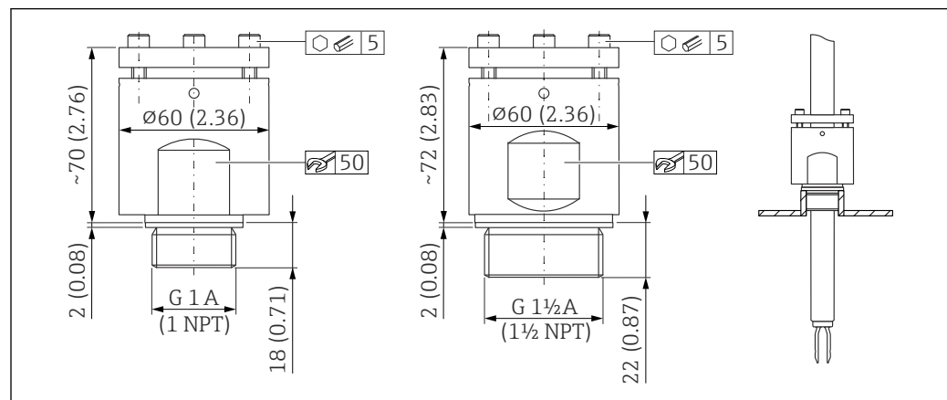
▣ 41 Casquillos deslizantes para alta presión. Unidad de medida mm (in)
