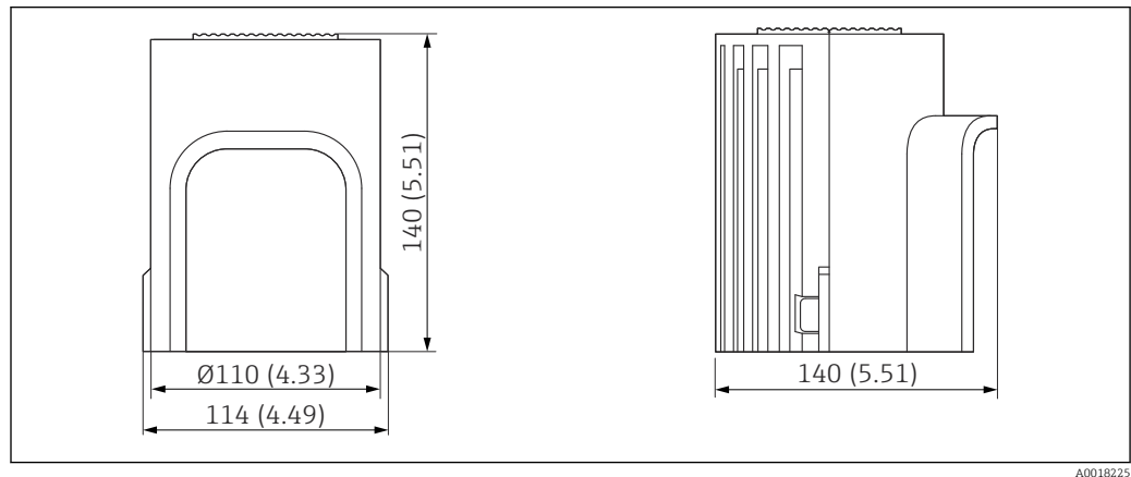
38 Medidas de la tapa de protección ambiental de PBT. Unidad de medida mm (in)
