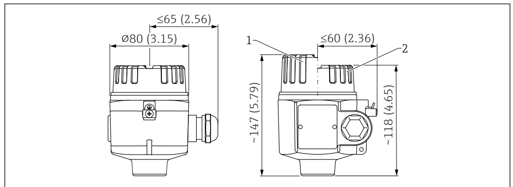
31 Medidas de la caja de 316L, con adaptador roscado en el sensor. Unidad de medida mm (in)
