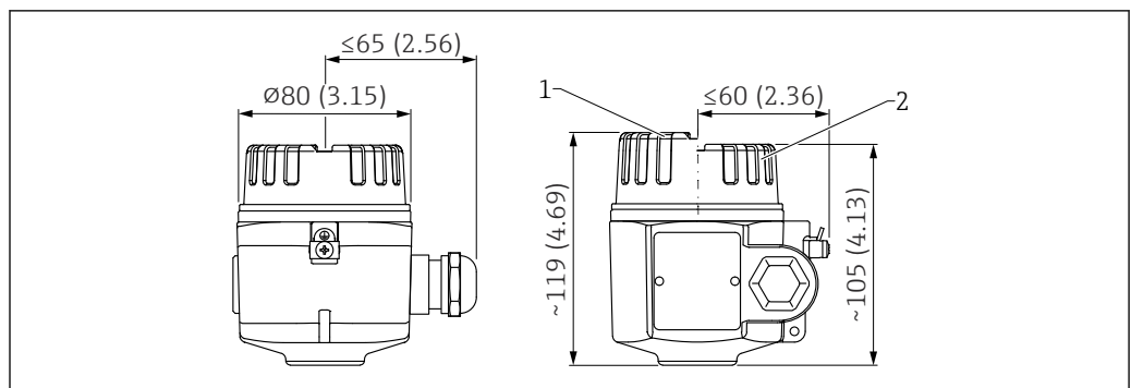
▣ 29 Medidas de la caja de aluminio. Unidad de medida mm (in)
