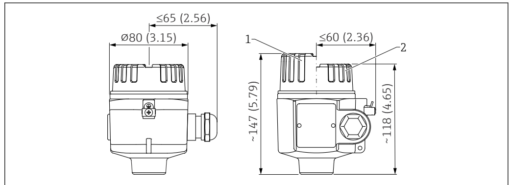
30 Medidas de la caja de aluminio, con adaptador roscado en el sensor. Unidad de medida mm (in)
