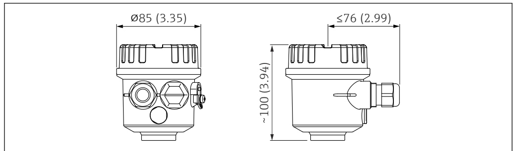
▣ 27 Medidas de la caja de plástico. Unidad de medida mm (in)
