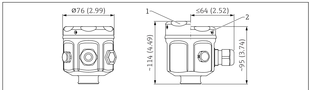
▣ 28 Medidas de la caja de 316L, higiénica. Unidad de medida mm (in)
