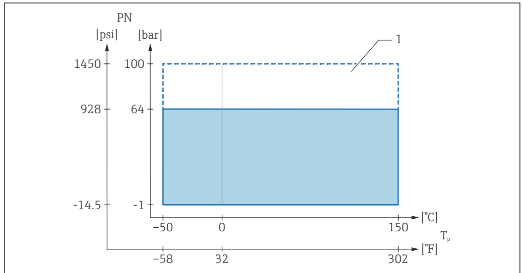
24 Rango de presión de proceso a la temperatura de proceso T_p hasta 150 °C (300 °F)
