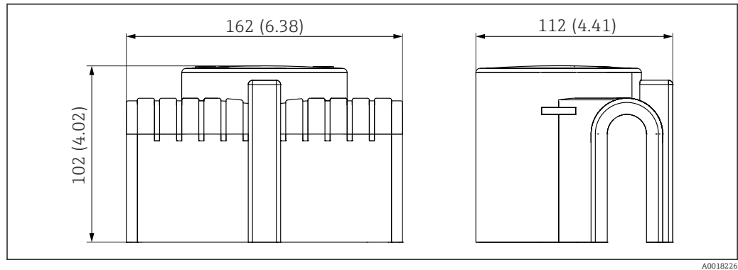
37 Medidas de la tapa de protección ambiental de PA6. Unidad de medida mm (in)
