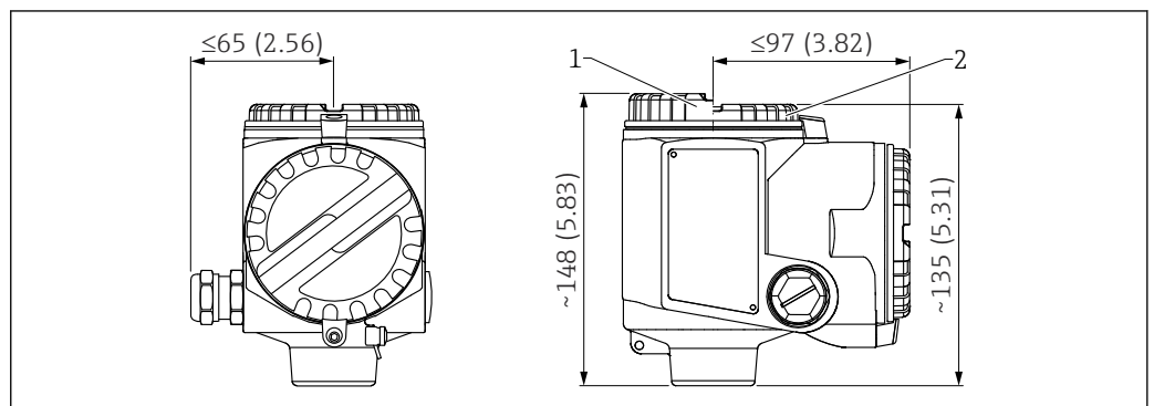
32 Medidas de la caja de aluminio con compartimento de terminales separado. Unidad de medida mm (in)
