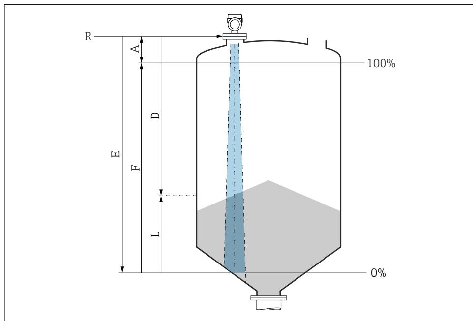
15 Konfigurationsparameter för nivåmätning i bulkmaterial
