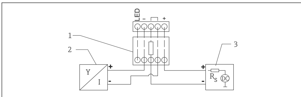
9 Funktionsdiagram över HART-enhet, RIA15 utan ljus, HART-kommunikationsresistormodul
