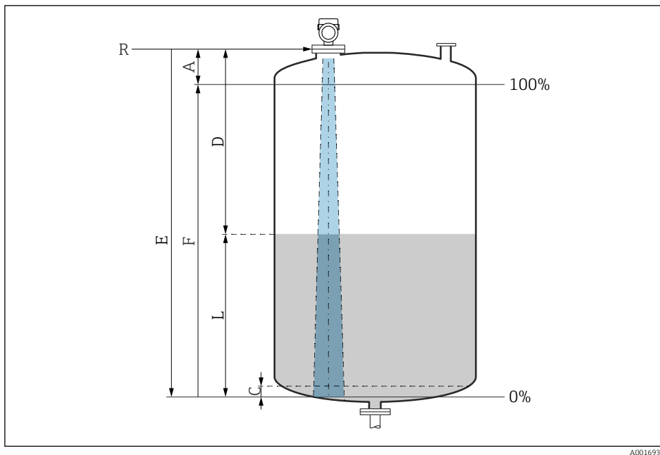
14 Konfigurationsparameter för nivåmätning hos vätskor
