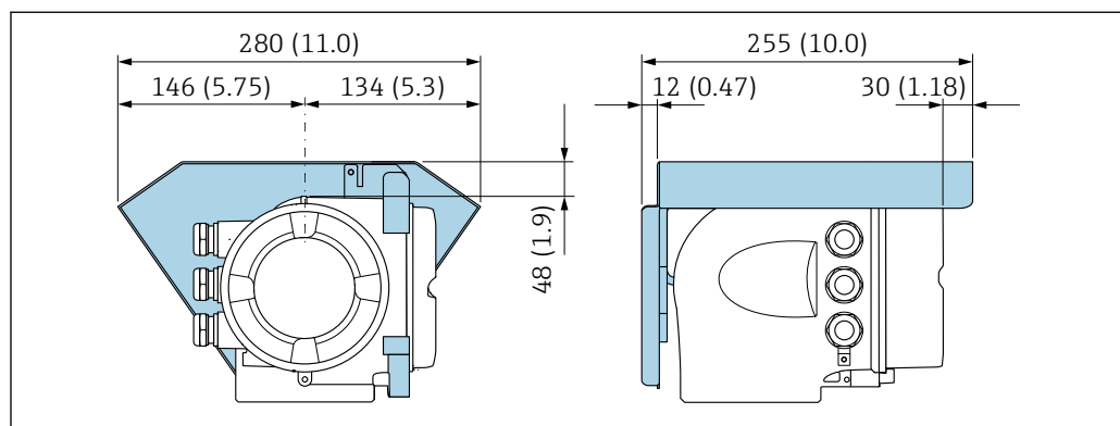
10 Tampa de proteção contra tempo para Proline 500 - unidade mm (pol.)
