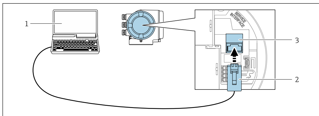
35 Conexão através de Interface de operação (CDI-RJ45)
