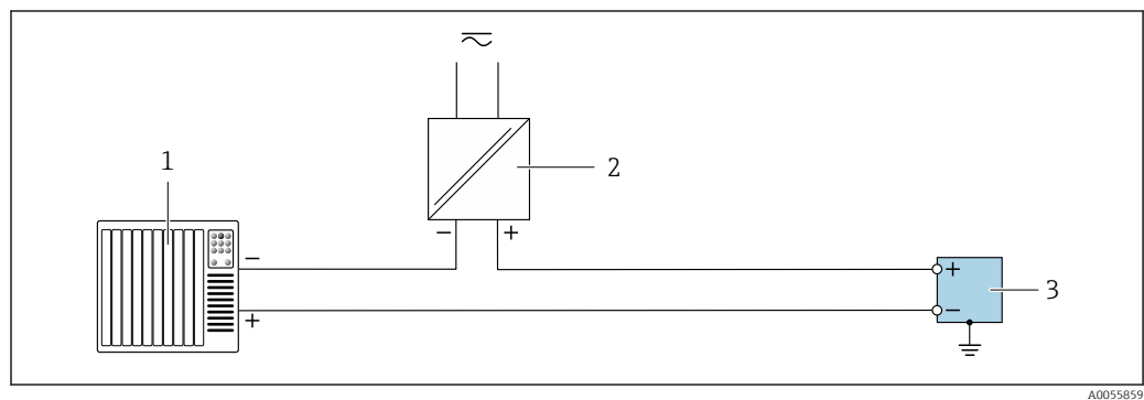
23 Exemplo de conexão para saída a relé
