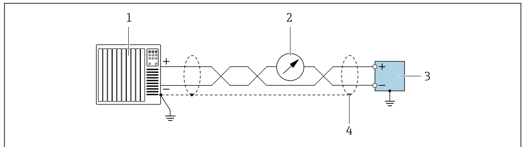
25 Exemplo de conexão para saída em corrente 4 para 20 mA com HART (ativa)
