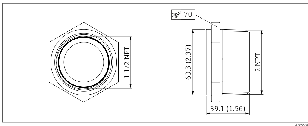
31 Размеры адаптера UNI
