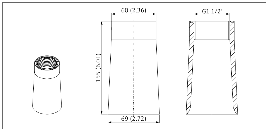
32 Размеры трубки для защиты от перелива среды 40 мм (1,5 дюйм). Единица измерения мм (дюйм)
