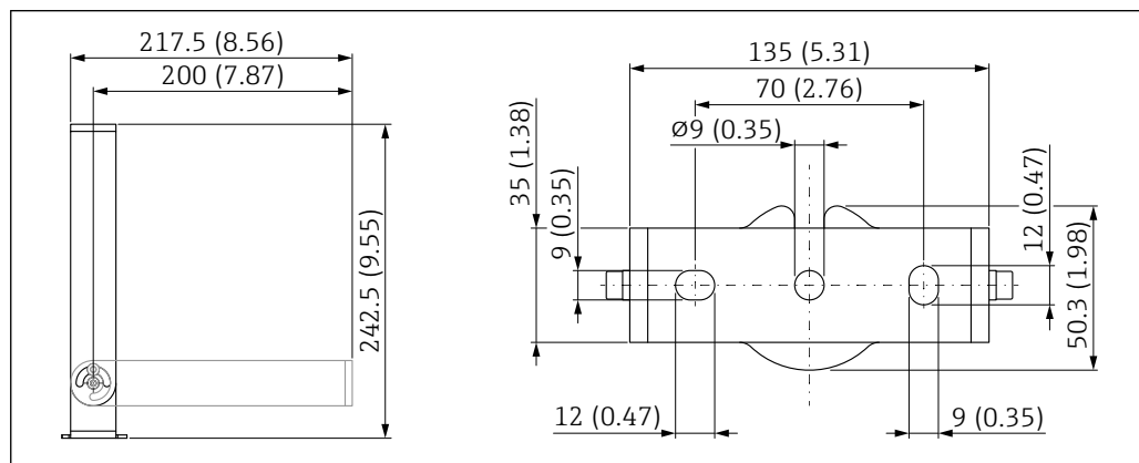
36 Размеры монтажного кронштейна. Единица измерения мм (дюйм)
