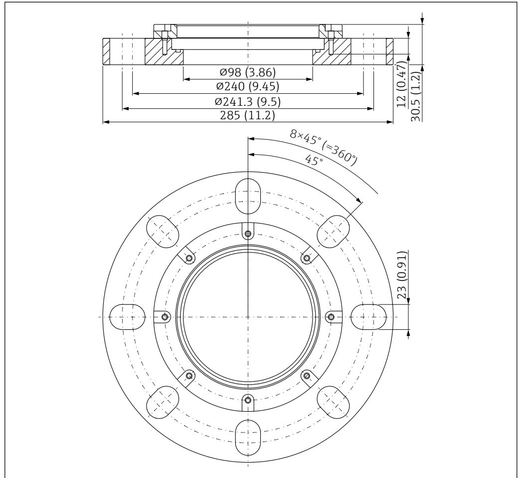
52 Размеры накладного фланца UNI 6"/DN150/150. Единица измерения мм (дюйм)
