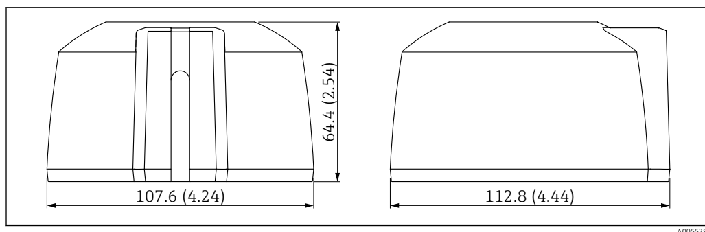
27 Размеры прибора с защитным козырьком, кабельный ввод сбоку. Единица измерения мм (дюйм)
