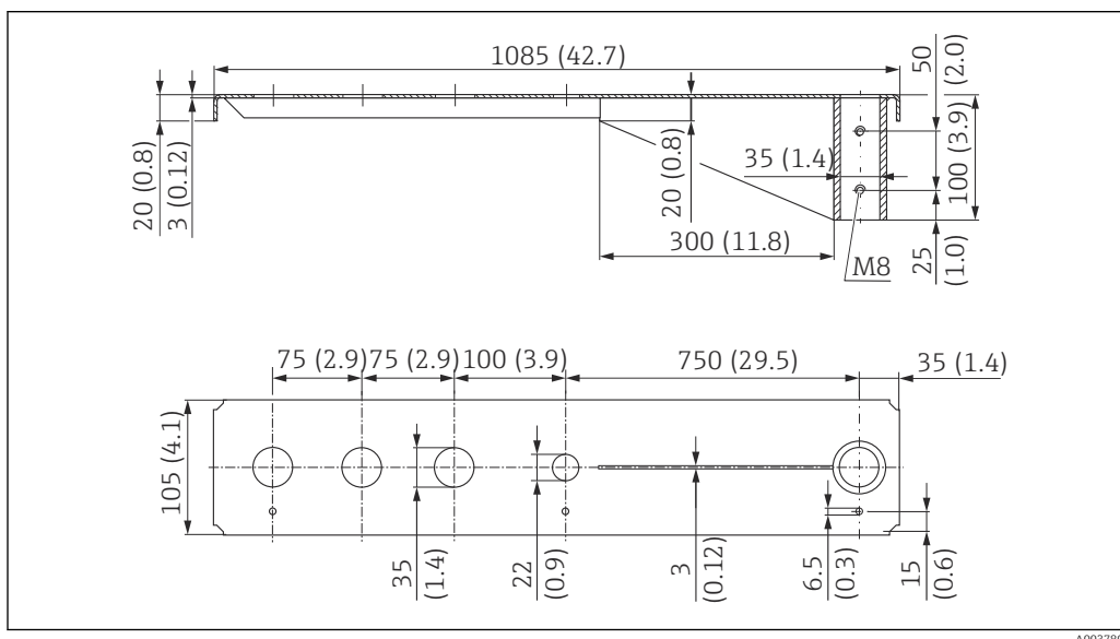
41 Размер консоли 1 000 мм с шарниром, технологическое соединение на кабельном вводе датчика. Единица измерения мм (дюйм)
