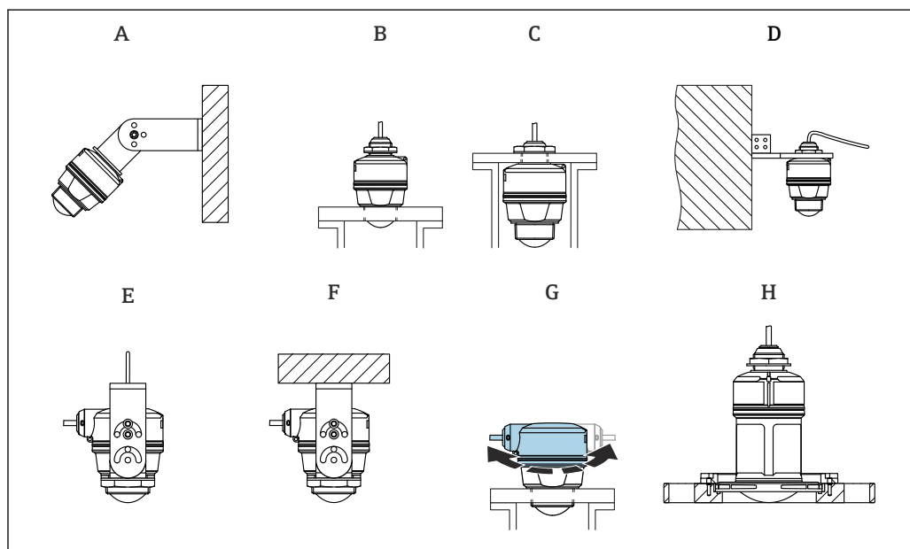
2 Монтаж на стене или потолке
