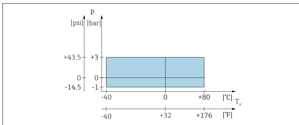
59 Допустимый диапазон рабочей температуры и рабочего давления
