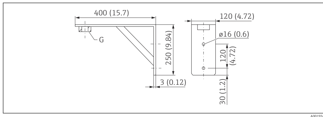
38 Размеры монтажного кронштейна. Единица измерения мм (дюйм)
