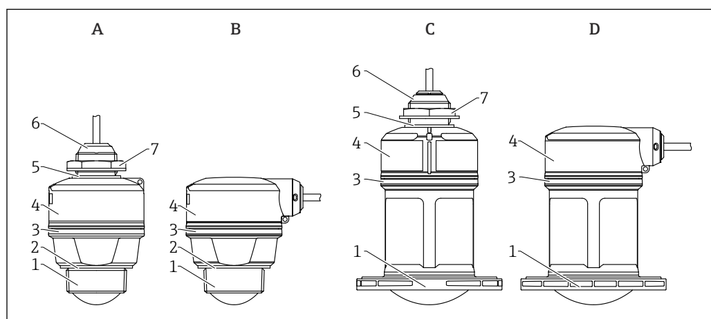
1 Конструкция прибора
