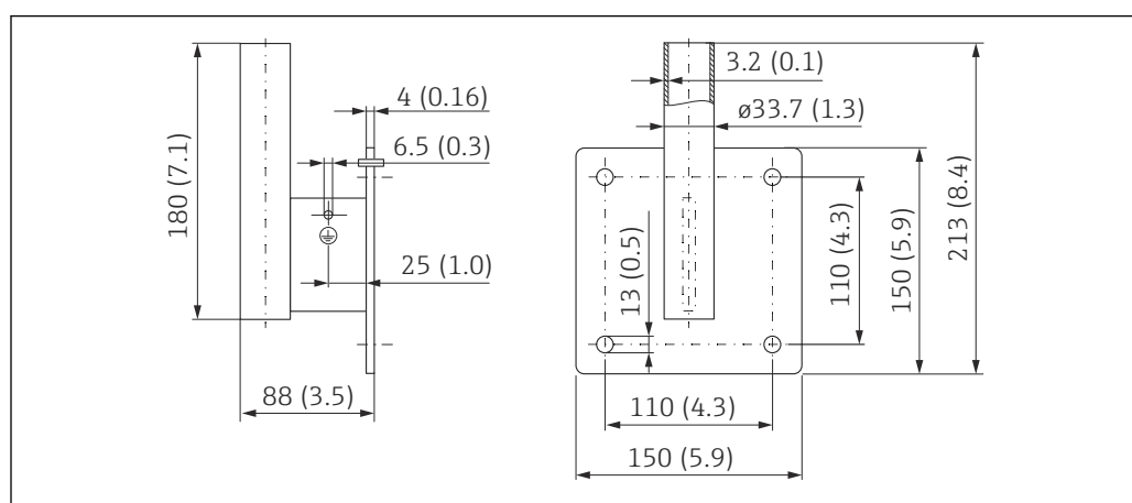
47 Размеры настенного кронштейна. Единица измерения мм (дюйм)
