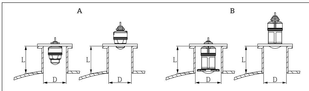
3 Монтаж в патрубке
