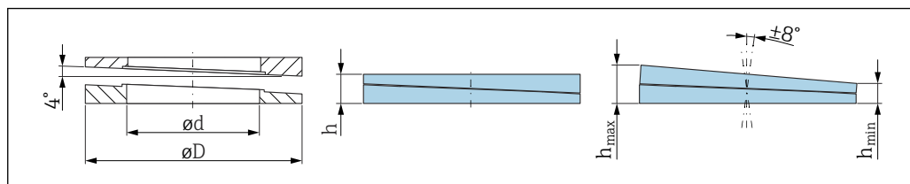
56 Размеры
