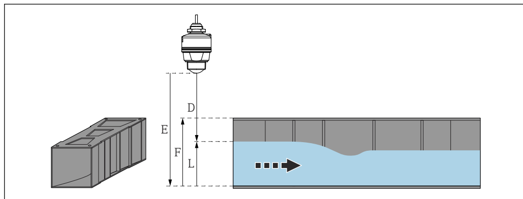
23 Пример: измерительный лоток Хафаги-Вентури
