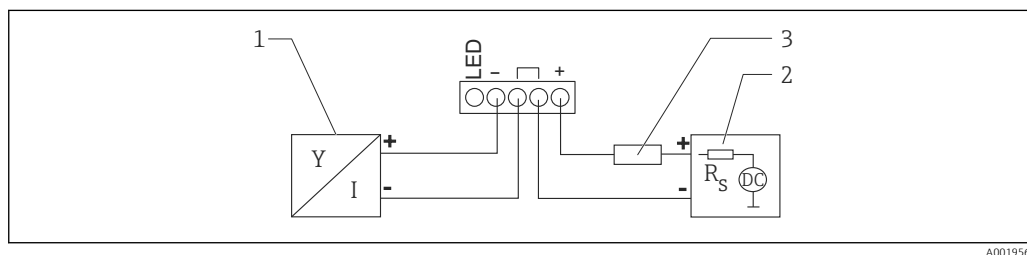
12 Функциональная схема прибора с интерфейсом HART и индикатором сигналов RIA15 без подсветки
