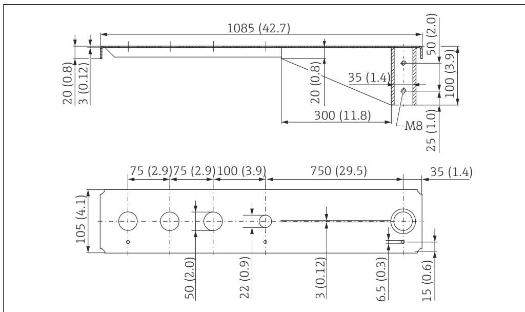
44 Размеры консоли 1 000 мм с шарниром, технологическое соединение на стороне антенны датчика G 1½". Единица измерения мм (дюйм)
