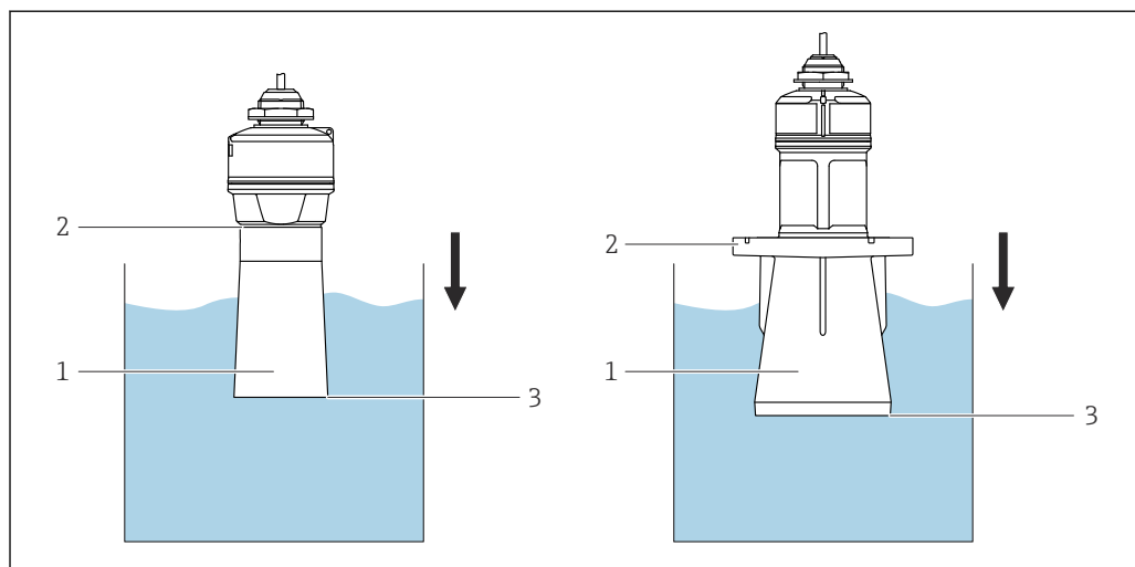
5 Функция трубки для защиты от заполнения водой
