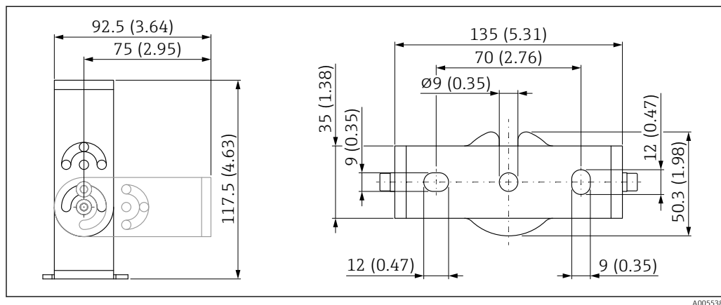
34 Размеры монтажного кронштейна. Единица измерения мм (дюйм)
