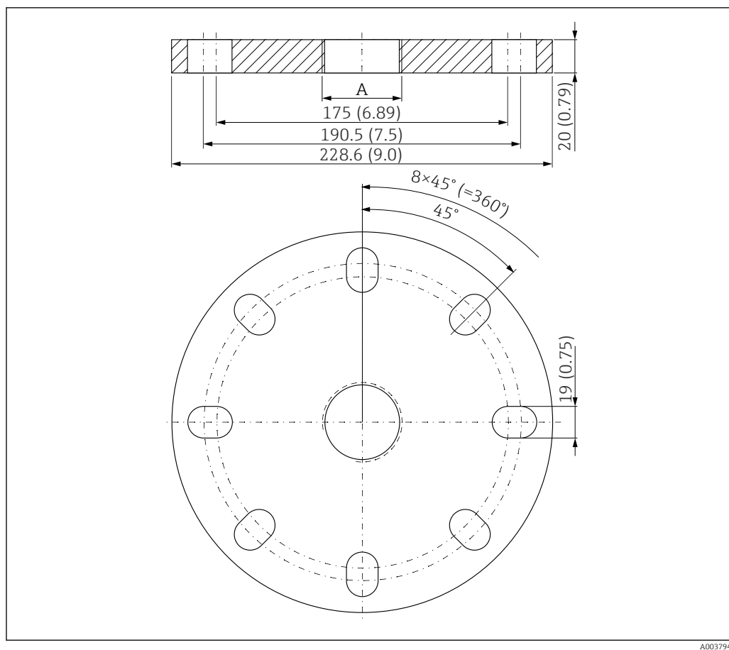
55 Размеры фланца UNI 4 дюйма/DN100/100. Единица измерения мм (дюйм)
