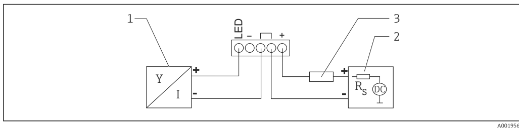
13 Функциональная схема прибора с интерфейсом HART и индикатором сигналов RIA15 с подсветкой
