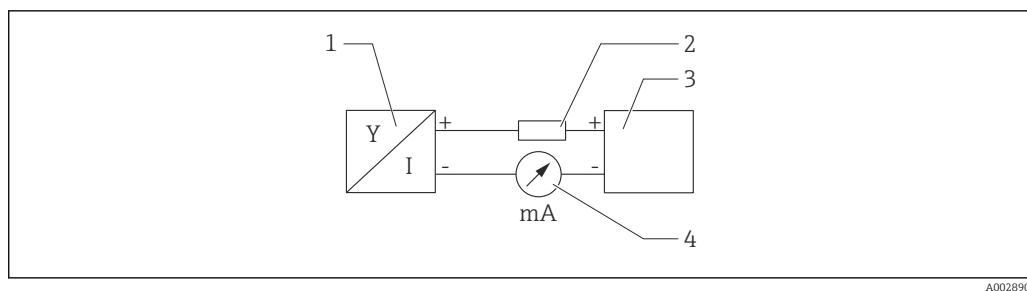
11 Функциональная схема подключения HART
