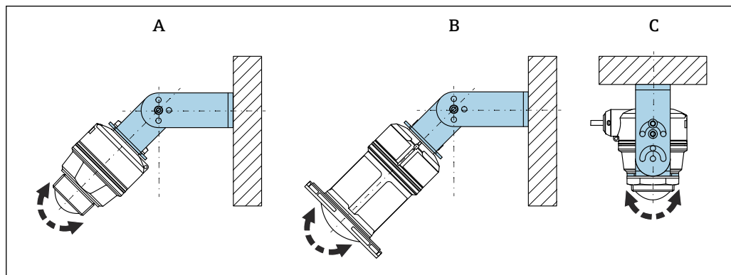
6 Установка с монтажным кронштейном, регулируемая
