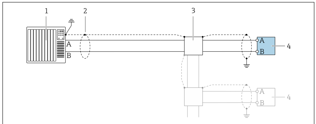
22 Exemple de raccordement pour Modbus RS485, zone non explosible et zone 2/Div. 2
