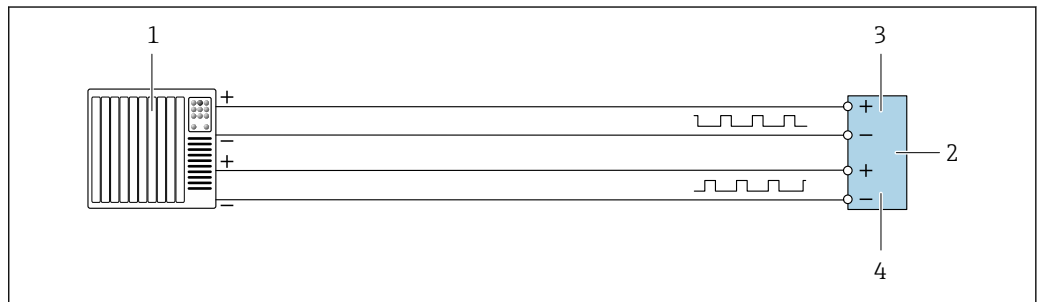
27 Exemple de raccordement pour la sortie impulsion double (active)
