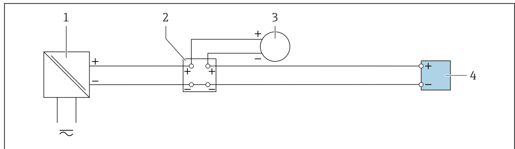
30 Exemple de raccordement pour entrée courant 4 à 20 mA
