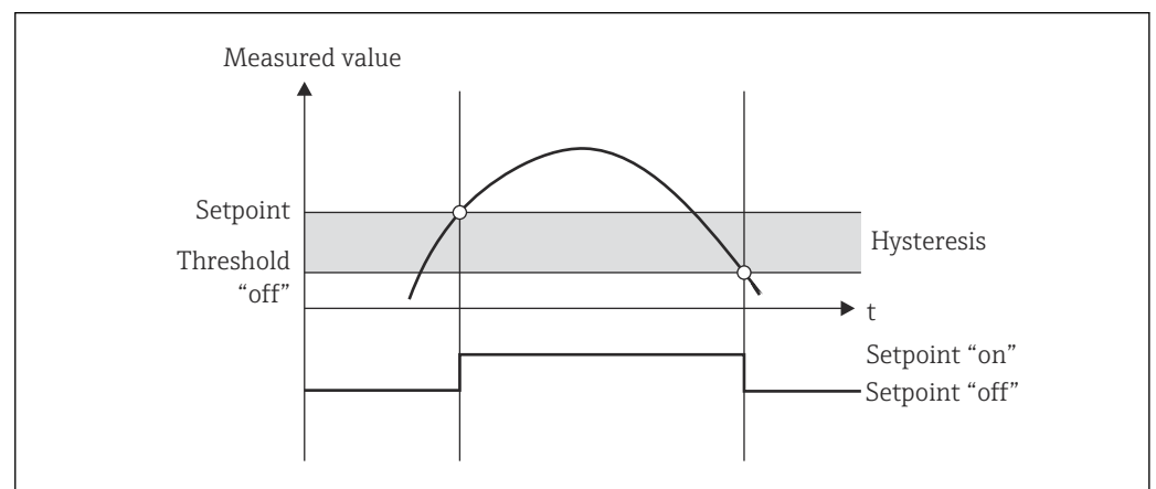
28 Betriebsart "GW oben"
