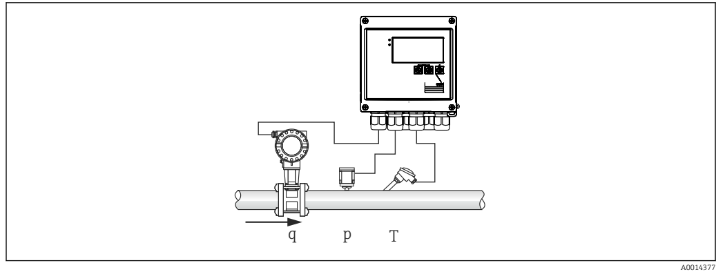
■ 26 Anwendung Tarifzähler für Dampfmasse und Energiefluss (Option)
