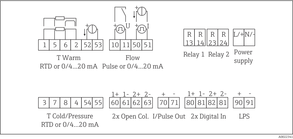
15 Anschlussbild des Geräts
