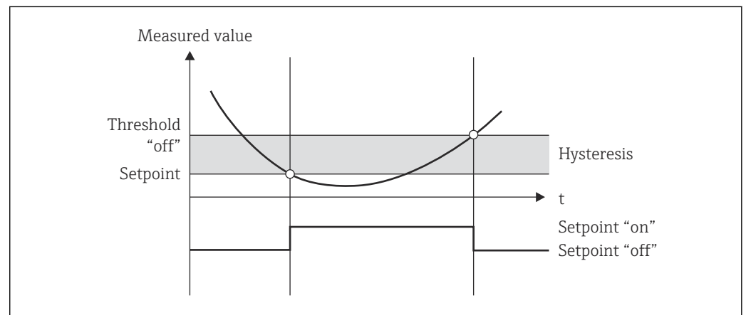
27 Betriebsart "GW unten"
