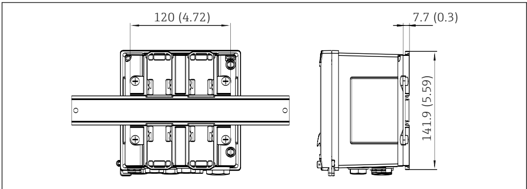
41 Abmessungen Hutschienenadapter in mm (in)
