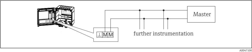
21 Anschluss M-Bus
