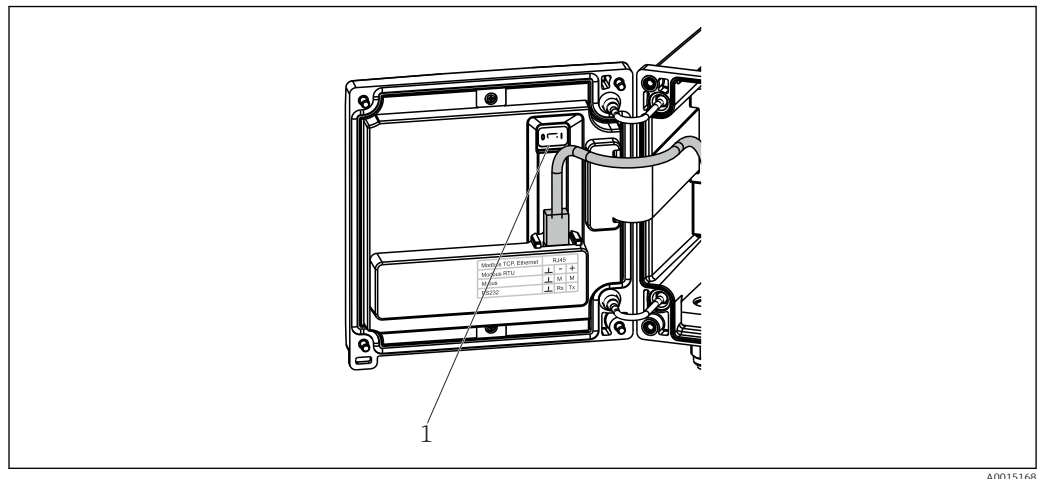
23 Verriegelungsschalter
