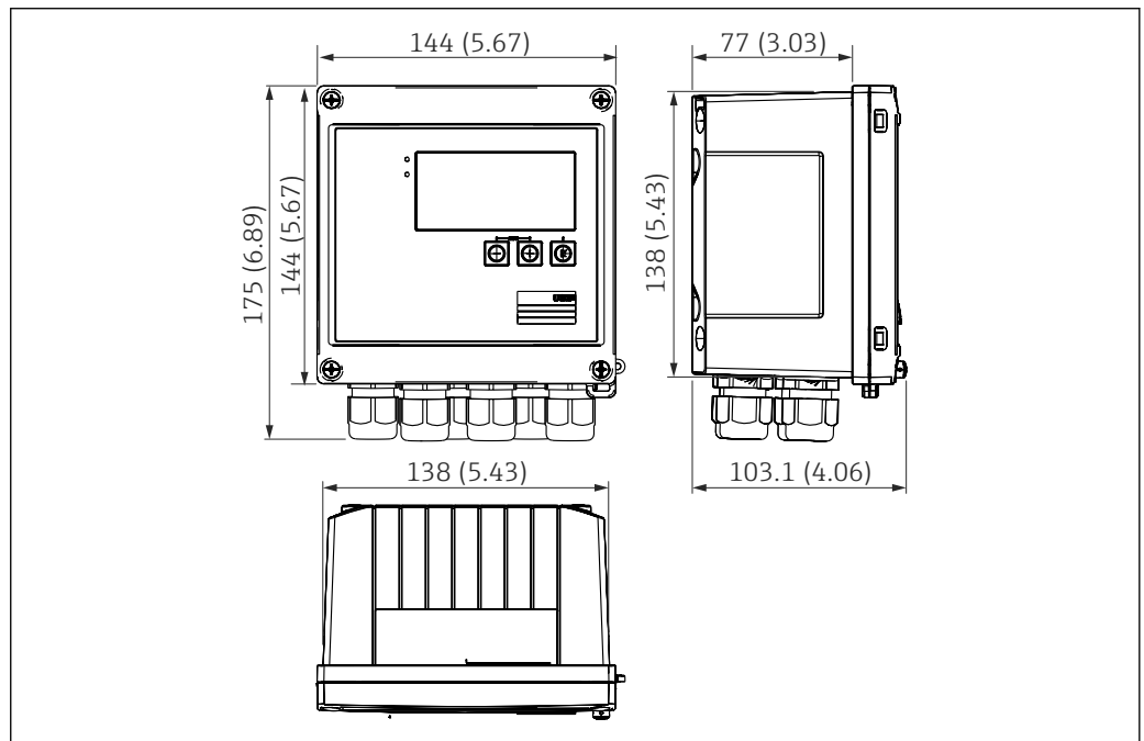
38 Gehäuse des EngyCal; Abmessungen in mm (in)
