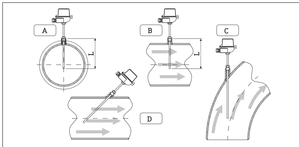
13 Einbauarten Temperatursensoren
