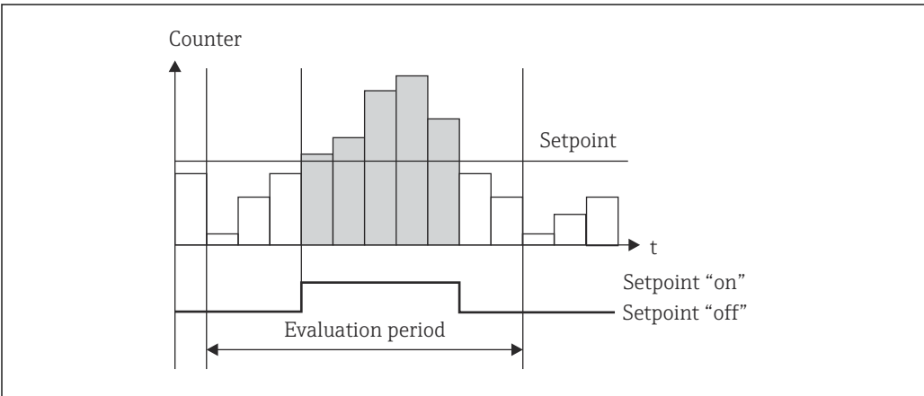
30 Grenzwert für Zähler
