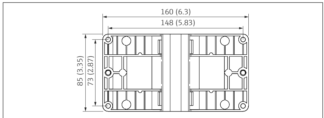
39 Montageplatte für Wand-, Rohr- und Schalttafeleinbau; Abmessungen in mm (in)
