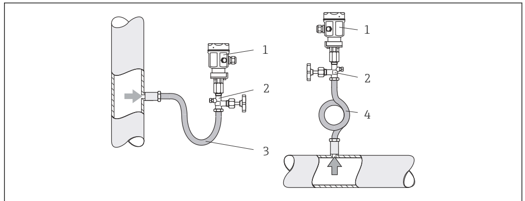
■ 14 Messanordnung Druckmessung in Dämpfen
