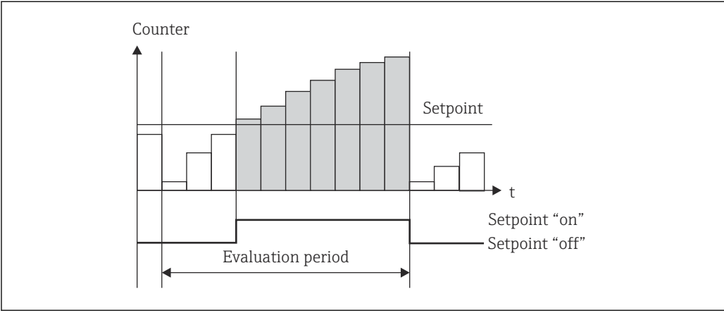
29 Grenzwert für Zähler
