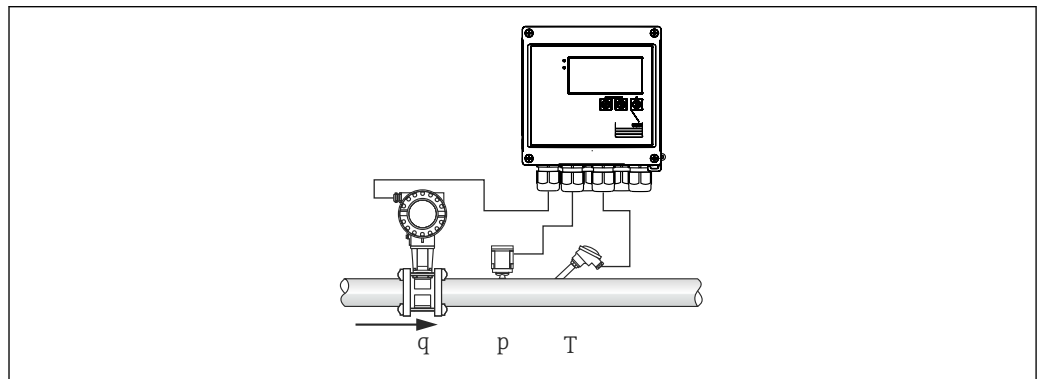
25 Anwendung Dampfmasse und Energie
