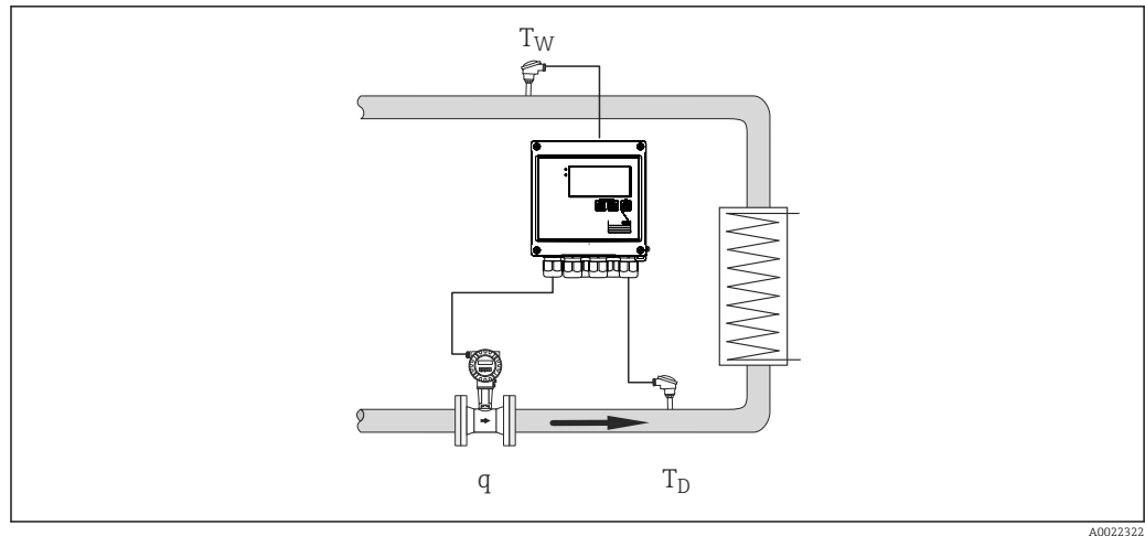
35 Wärmedifferenz/T
