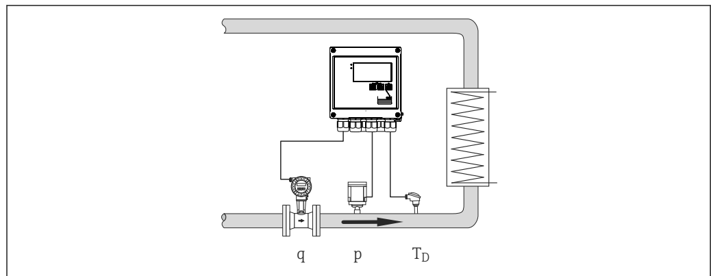
36 Wärmemenge oder Wärmedifferenz/p+T
