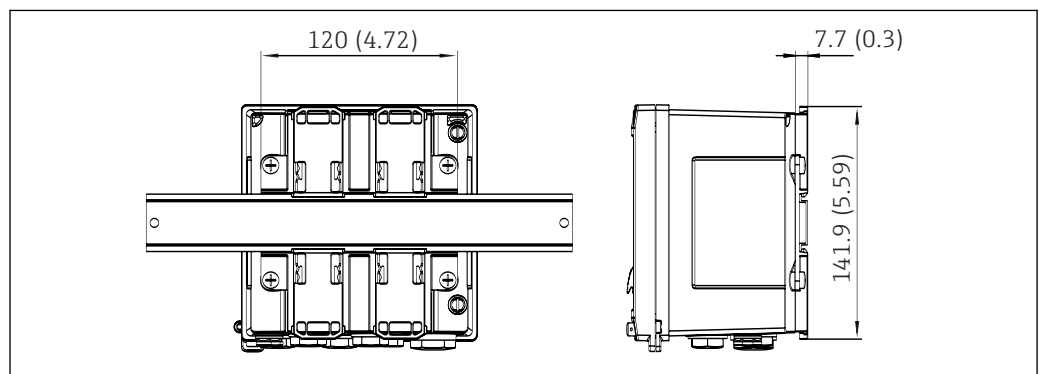
4 Abmessungen Hutschienenadapter in mm (in)
