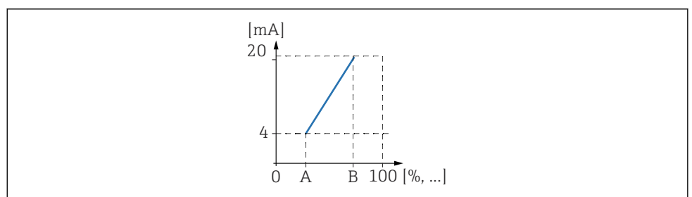
62 Principio de funcionamiento de la rangeabilidad de la corriente
