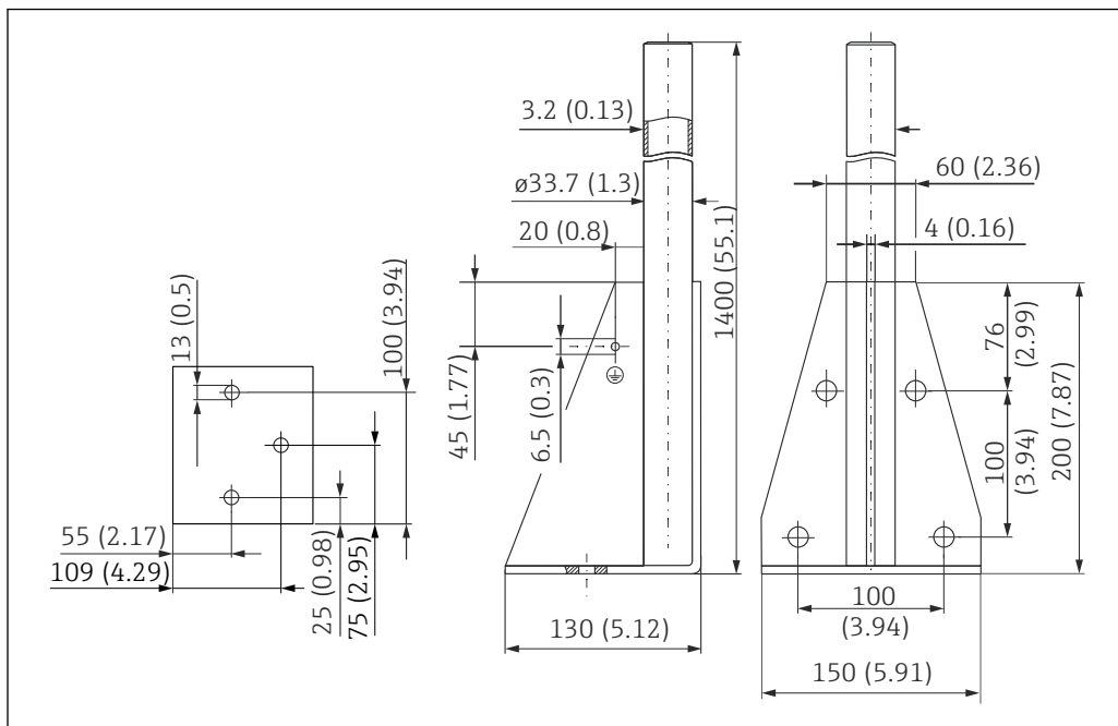
68 Medidas. Unidad de medida mm (in)
