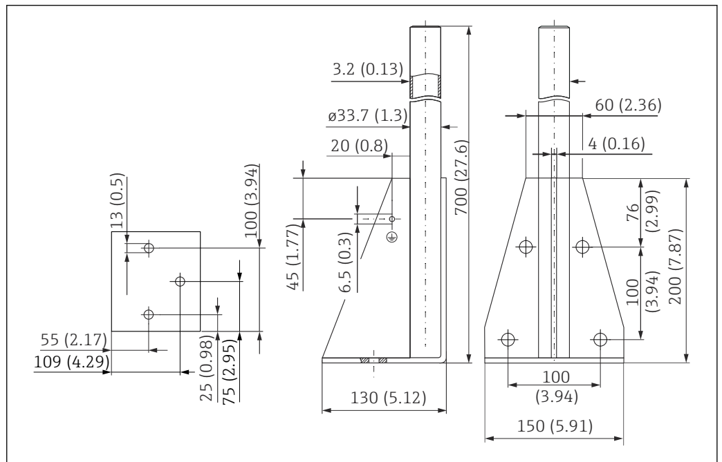
67 Medidas. Unidad de medida mm (in)
