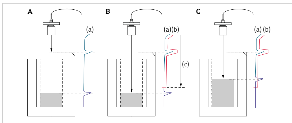
50 Principio de funcionamiento de la función de mapeado (supresión de falsos ecos)
