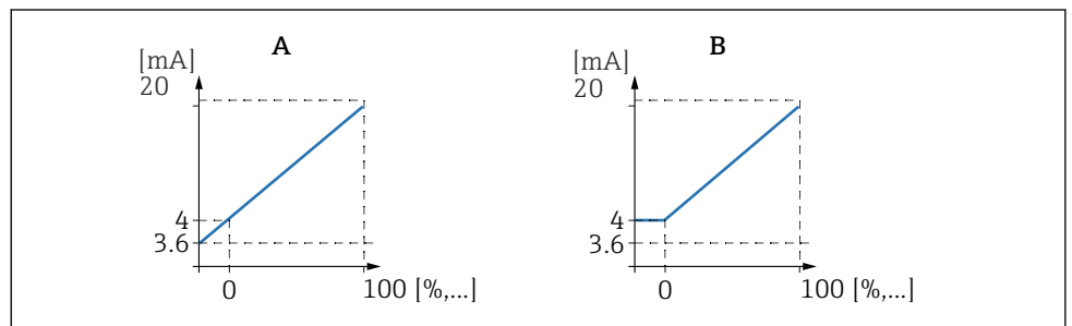
61 Umbral de 4 mA (solo para span de corriente = 4 ... 20 mA)
