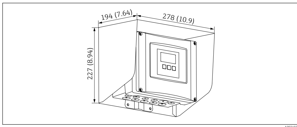
65 Tapa de protección ambiental para caja de policarbonato para montaje en campo. Unidad de medida mm (in)
