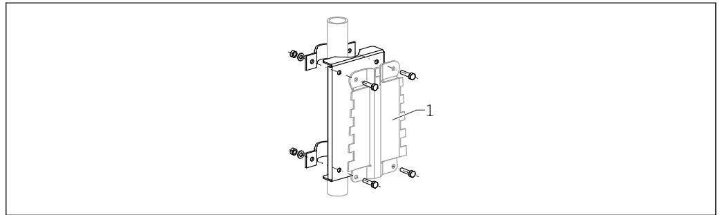
66 Placa de montaje para caja para montaje en campo de policarbonato
