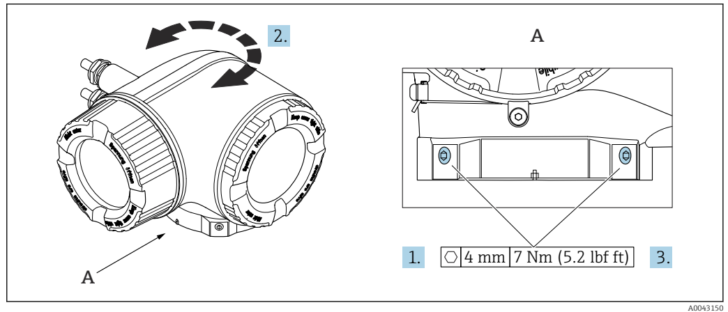
11 Ex-Gehäuse
