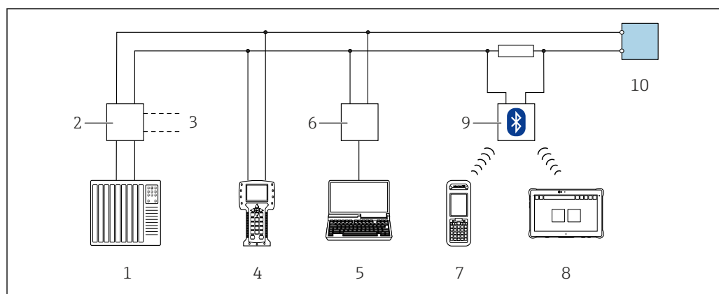
13 Варианты дистанционного управления по протоколу HART (пассивный режим)
