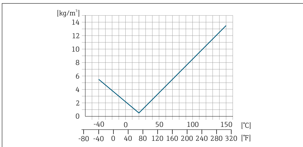
23 Калибровка по плотности на месте эксплуатации, в примере при +20 °C (+68 °F)
