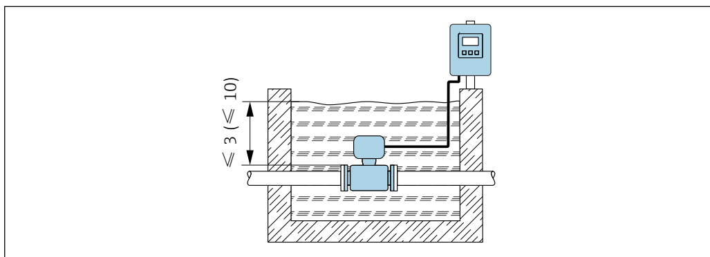
図 5 水中に常時浸漬する場合の設置
