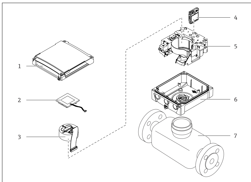
図 2 一体型の主要コンポーネント
