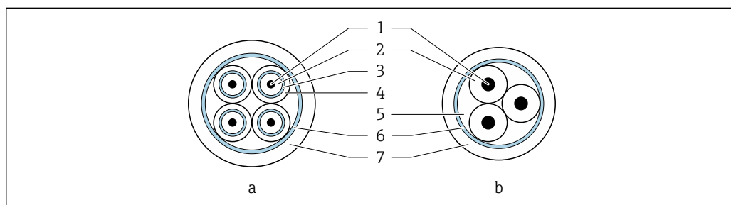
図 8 ケーブル断面
