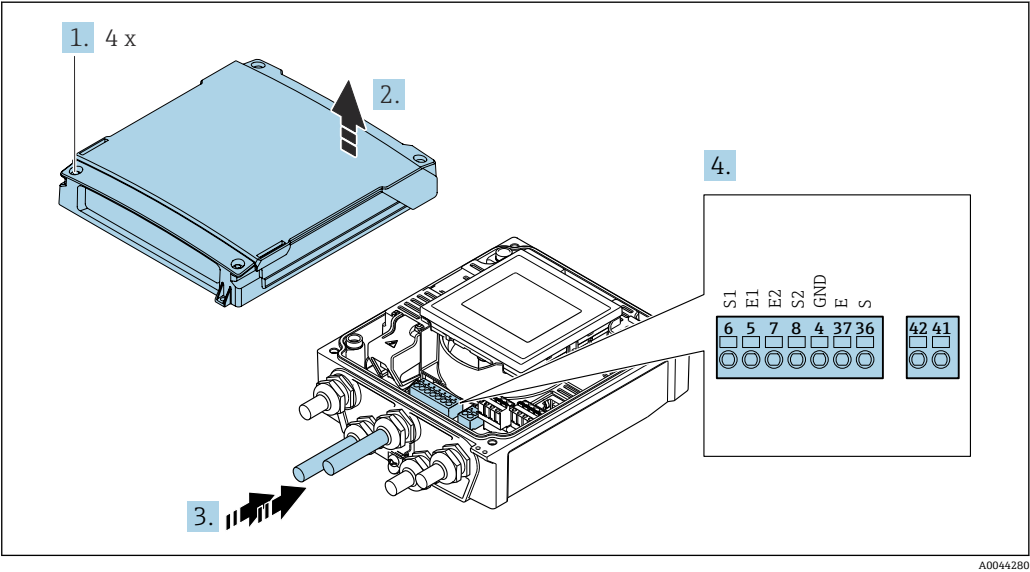
図 13 変換器：端子付きメイン電子モジュール
