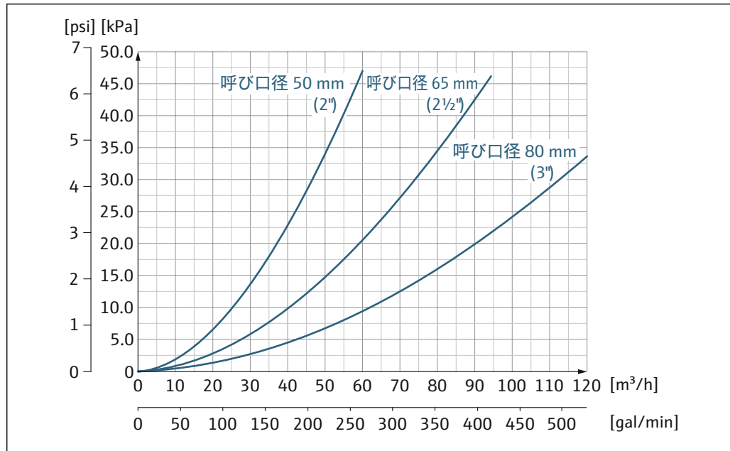
図 18 呼び口径 50~80 mm (2~3") の圧力損失：「設計」のオーダーコード、オプション C「固定フランジ、縮小計測チューブ、0 x 呼び口径 上流側/下流側直管長」の場合
