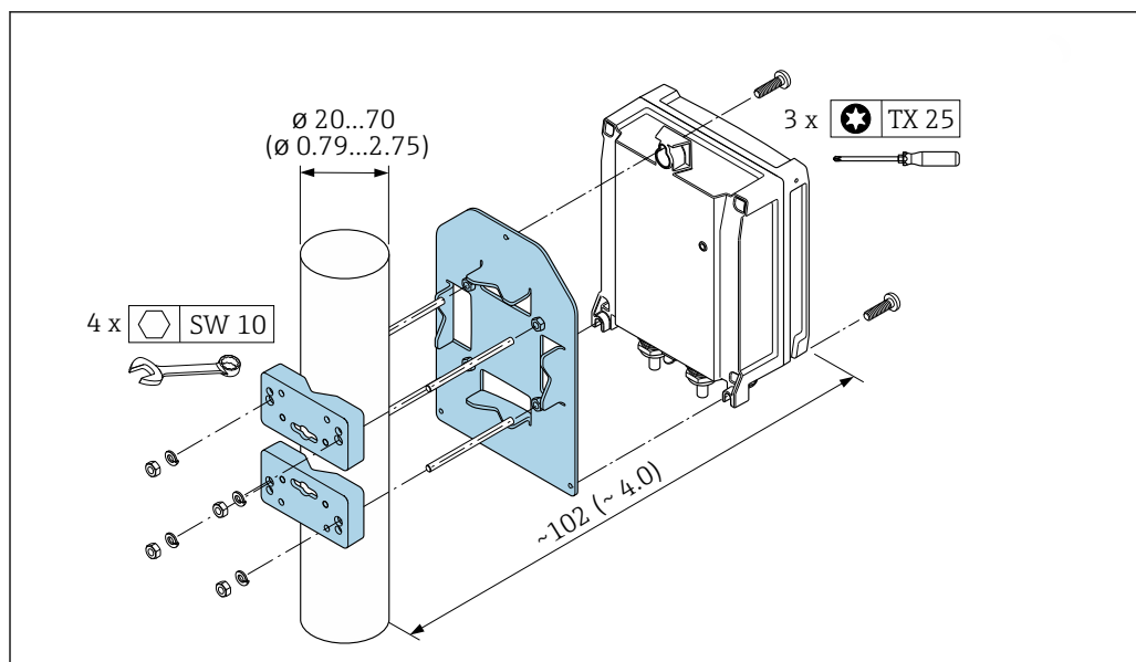
図 7 単位 mm (in)
