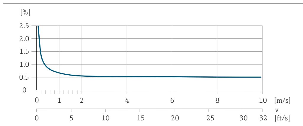
図 17 最大測定誤差 (%) o.r.
