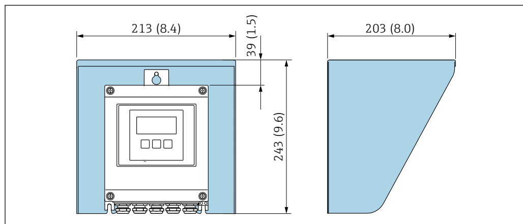
図 4 日除けカバー、寸法：mm (in)
