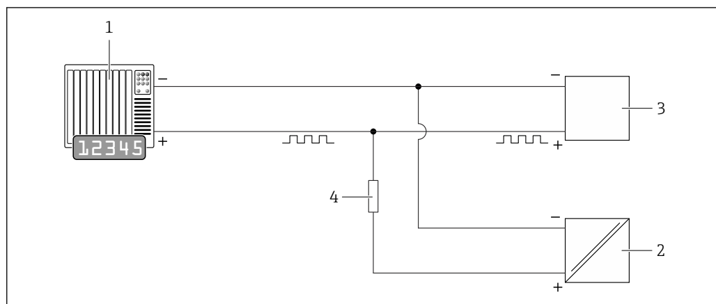
図 15 パルス出力（パッシブ）の接続例
