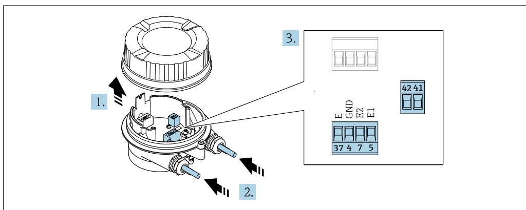
図 12 センサ：接続モジュール
