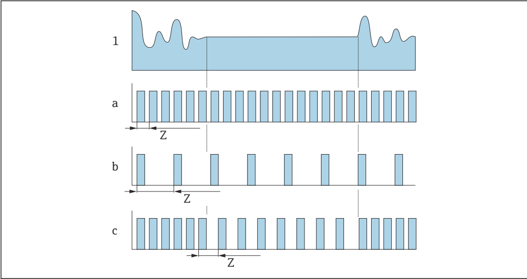
図 16 各種のデータのログ方法の動作原理
