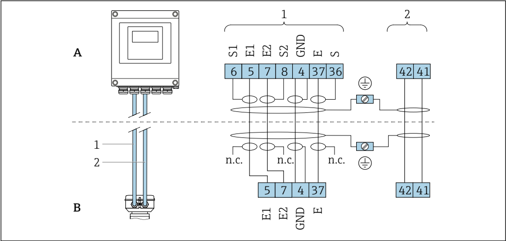
図 9 分離型の端子の割当て
