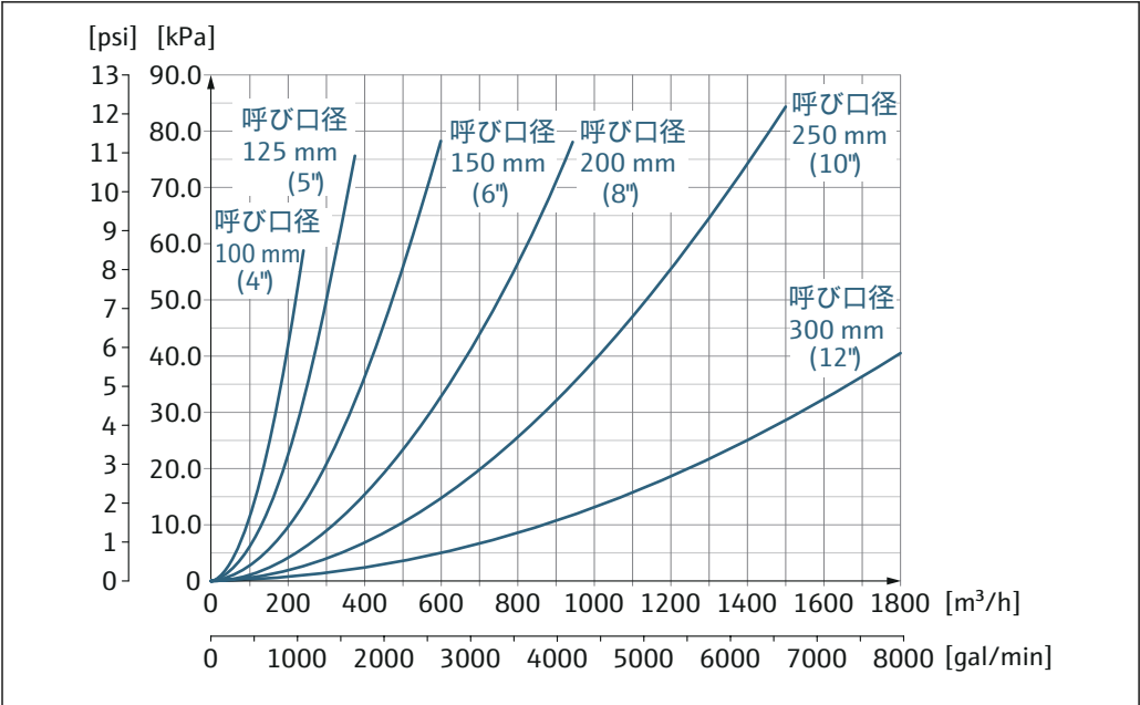
図 19 呼び口径 100～300 mm (4～12") の圧力損失：「設計」のオーダーコード、オプション C「固定フランジ、縮小計測チューブ、0 x 呼び口径 上流側/下流側直管長」の場合
