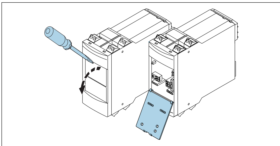
10 Otwieranie panelu przedniego
