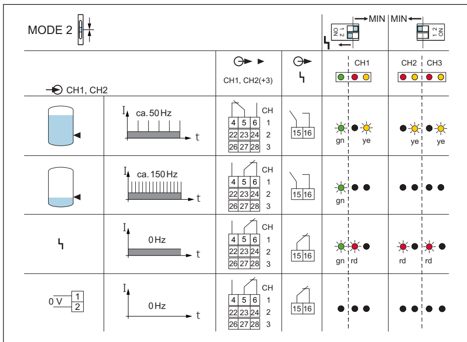
17 Tryb przełączania i sygnalizacja usterki
