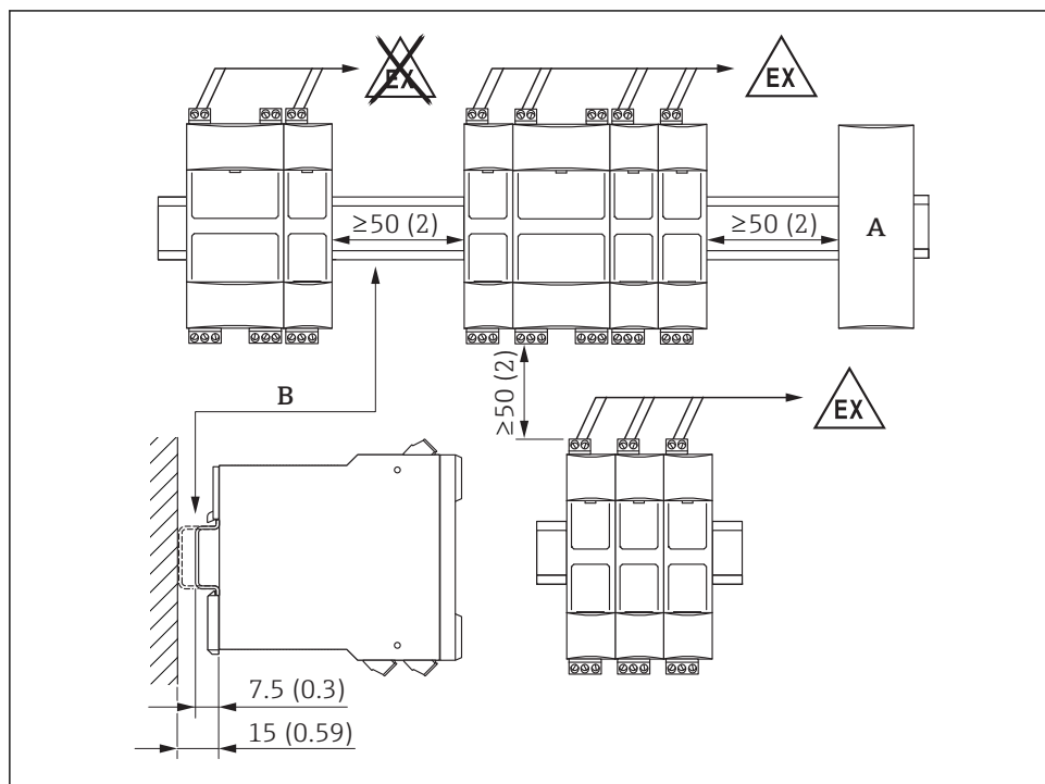
2 Minimalne odstęp, pozycja pozioma. Jednostka miary mm (in)
