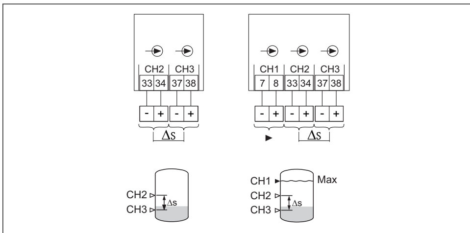
8 Podłączanie czujników w układzie regulacji dwupołożeniowej \Delta s
