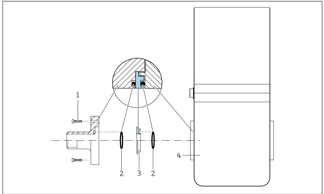
图 5 安装接地环
