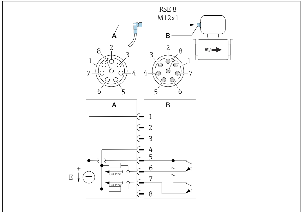
图 6 连接仪表
