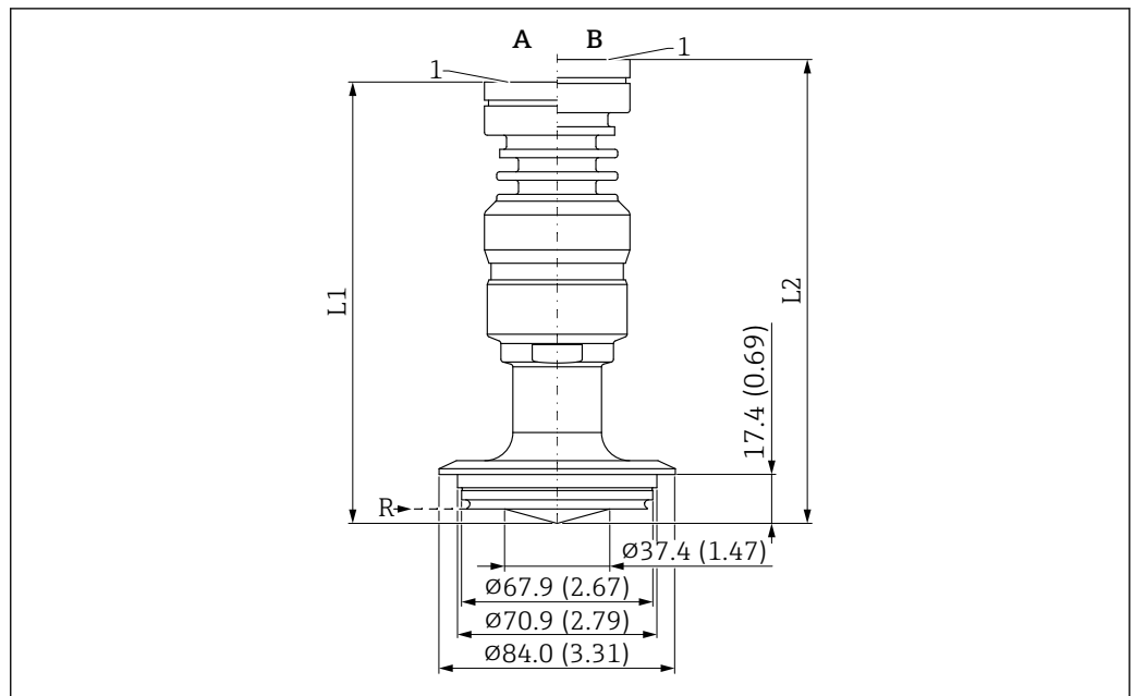
■ 52 PEEK 外装付フラッシュマウントアンテナ、40 mm (1.5 in)、バリベント N チューブ DN65-162 の寸法。測定単位 mm (in)
