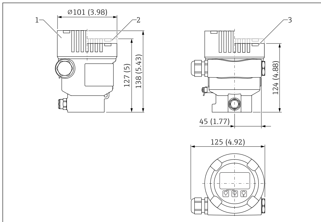
41 寸法；シングルコンパートメントハウジング（アルミニウム、コーティング）；M20 カップリングおよびプラグ（プラスチック）付き。測定単位 mm (in)
