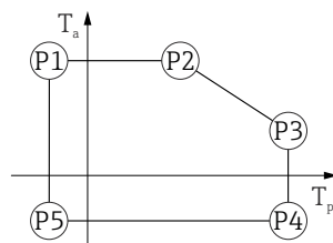
図 23 アルミニウムハウジング、コーティング ; プロセス温度 -10～+200 °C (+14～+392 °F)
