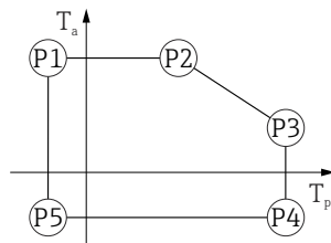
■ 31 SUS 316L 相当製ハウジング ; プロセス温度 -20~+200 °C (-4~+392 °F)
