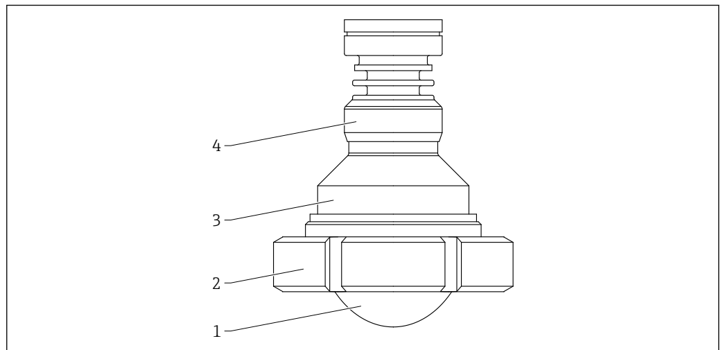
■ 57 材質 ; 外装付フラッシュマウントアンテナ、80 mm (3 in)、ナット DIN11851。測定単位 mm (in)
