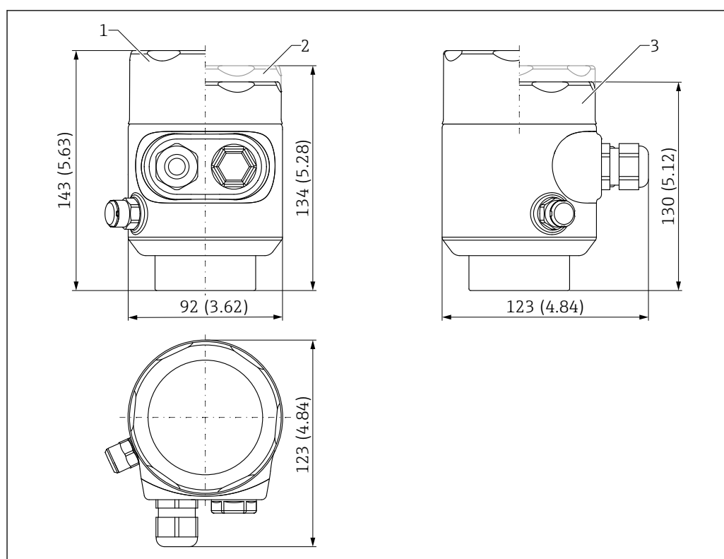
図 42 寸法；シングルコンパートメントハウジング（SUS 316L 相当、サニタリ仕様）；M20 カップリングおよびプラグ（プラスチック）付き。測定単位 mm (in)
