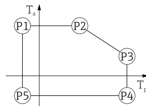
図 29 SUS 316L 相当製ハウジング ; プロセス温度 -10 \sim +200\text{ }^{\circ}\text{C} ( +14 \sim +392\text{ }^{\circ}\text{F} )
