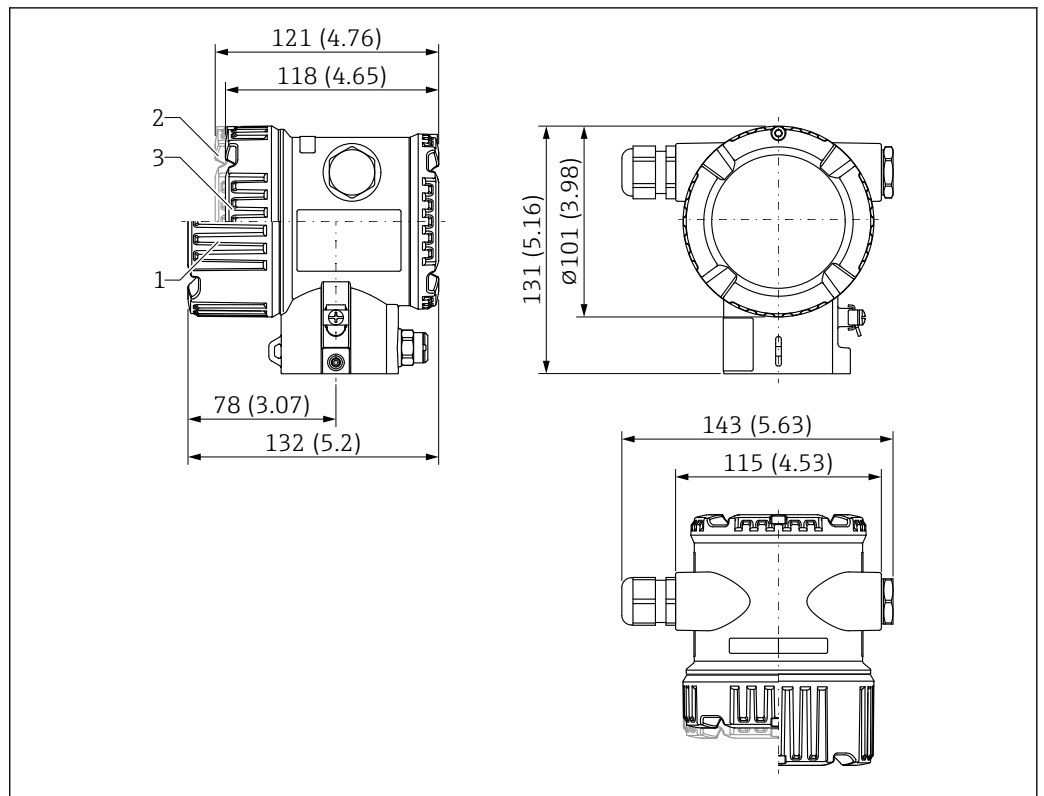
■ 43 寸法；デュアルコンパートメントハウジング（アルミニウム、コーティング）；M20 カップリングおよびプラグ（プラスチック）付き。測定単位 mm (in)
