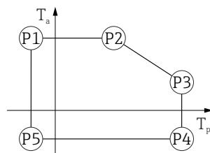
図 10 プラスチックハウジング；プロセス温度 -10\sim+150^{\circ}\text{C} ( +14\sim+302^{\circ}\text{F} )
