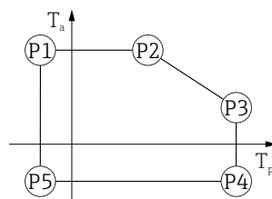
図 35 SUS 316L 相当製ハウジング、サニタリ仕様 ; プロセス温度 -10~+200 °C (+14~+392 °F)
