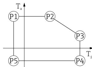
図 34 SUS 316L 相当製ハウジング、サニタリ仕様 ; プロセス温度 -10~+150 °C (+14~+302 °F)
