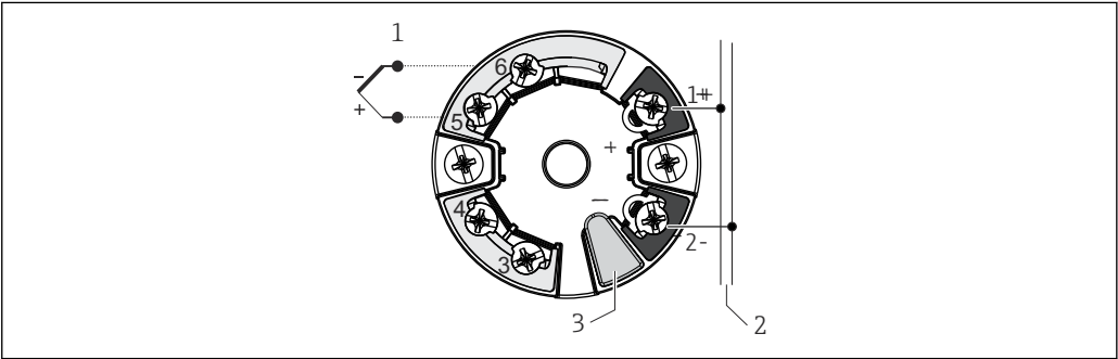
图 9 iTEMP TMT7x 或 iTEMPT MT31 模块化温度变送器（单路传感器输入）
