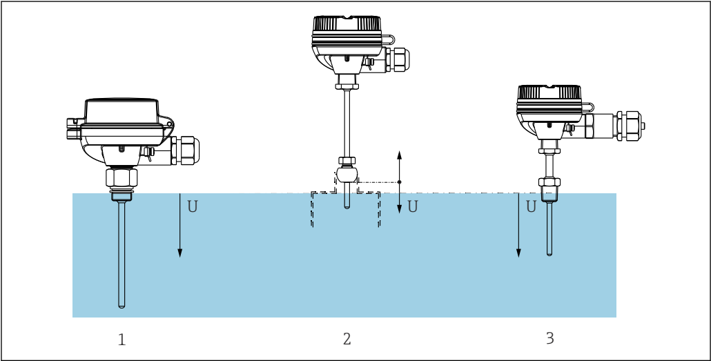
图 2 温度计直接接液测量 1 螺纹过程连接，无延长颈 2 球体或柱体焊接安装 3 带延长颈和螺纹过程连接
