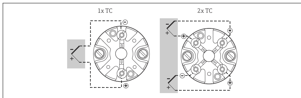
图 7 已安装的热电偶陶瓷端子接线块。
