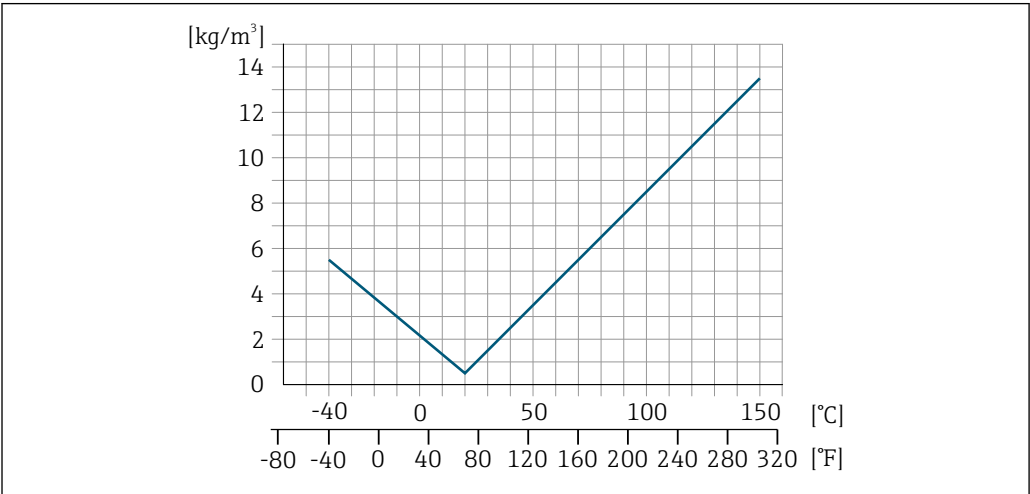
34 Regolazione della densità in campo, ad es. a +20 °C (+68 °F)
