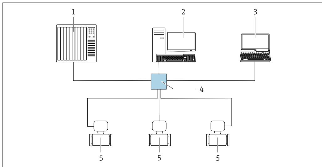
24 Opzioni per il funzionamento a distanza mediante rete EtherNet/IP: topologia a stella
