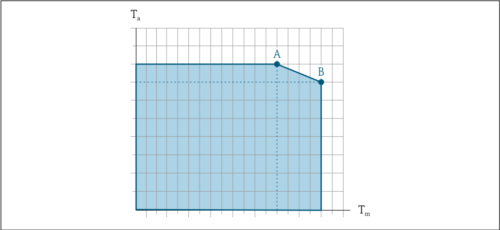
35 Rappresentazione esemplificativa, valori nella tabella sottostante. T_a Temperatura ambiente T_m Temperatura del fluido A Temperatura del fluido massima consentita T_m con T_{a\ max} = 60\ ^\circ\text{C} (140 °F); temperature del fluido superiori T_m richiedono una temperatura ambiente ridotta T_a B Temperatura ambiente massima consentita T_a per la temperatura del fluido massima specificata T_m del sensore
