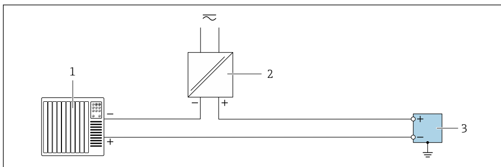
図 25 パルス出力/周波数出力/スイッチ出力（パッシブ）の接続例
