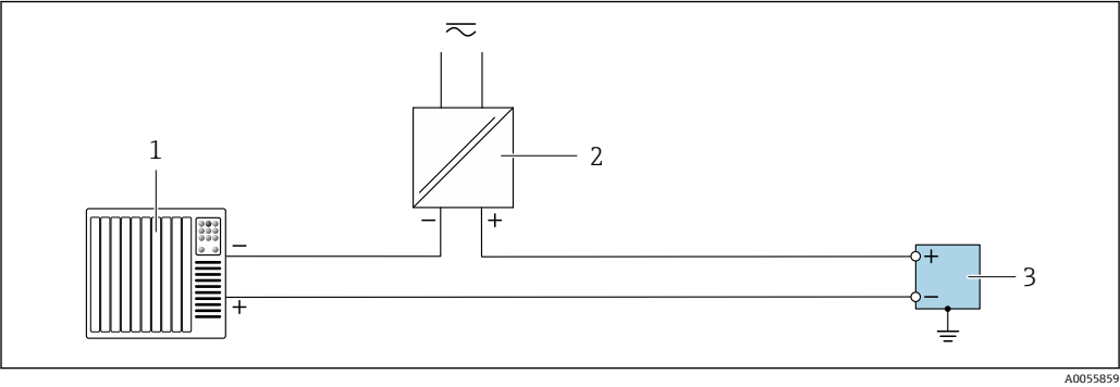
図 26 リレー出力の接続例 1 オートメーションシステム、スイッチ入力付き (例 : PLC) 2 電源 3 リレー出力付き変換器
