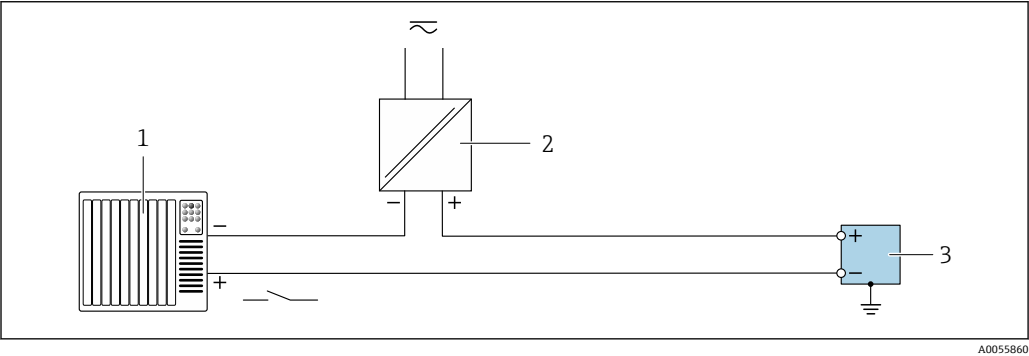
図 27 ステータス入力の接続例 1 オートメーションシステム、スイッチ出力 (パッシブ) 付き (例 : PLC) 2 電源 3 ステータス入力付き変換器
