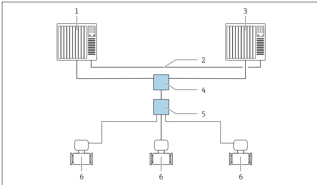
図 36 冗長システム (S2) のレイアウト例：スター型トポロジー
