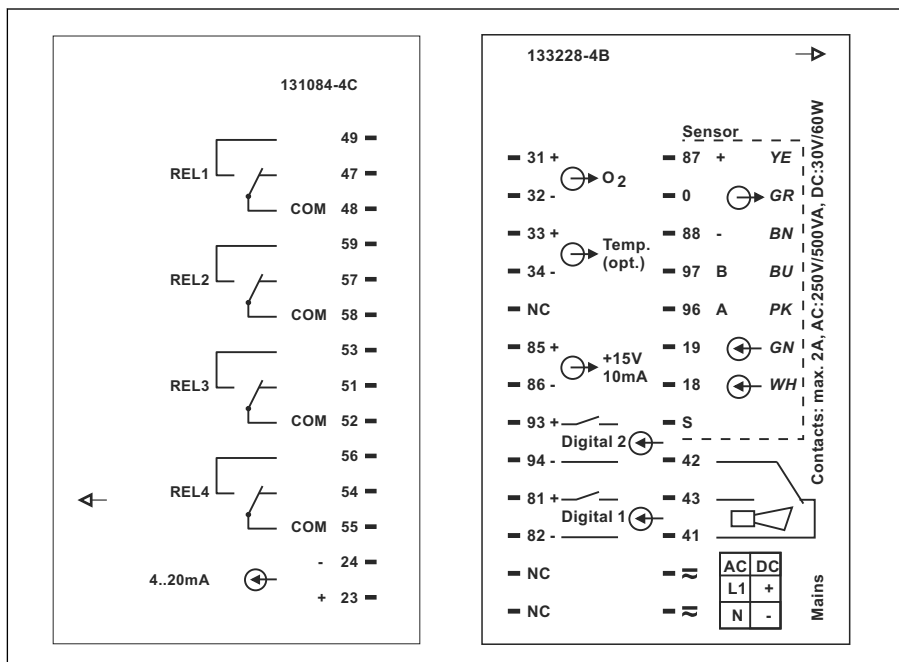
図 7 Liquisys M パネルマウント型機器の端子部ステッカー (WX/WS バージョン)
