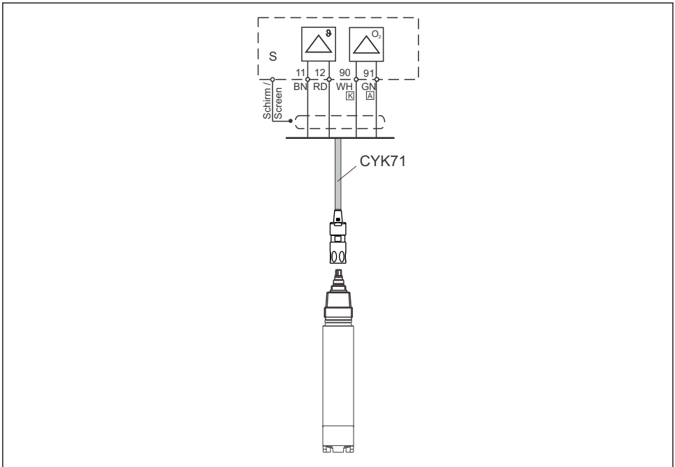
図 5 接続例：COS41 および CYK71 ケーブル
