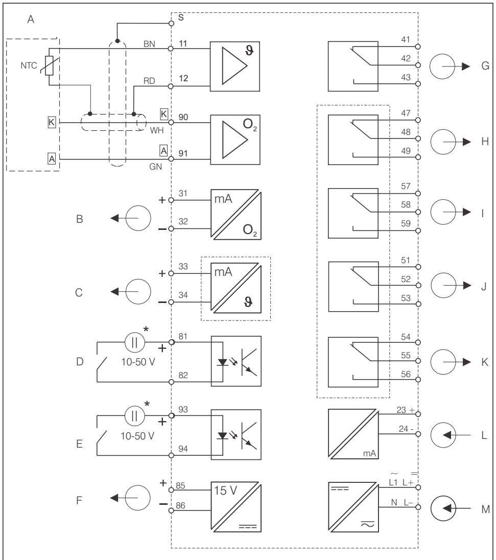
図 3 変換器の電気接続、DX または DS バージョン
