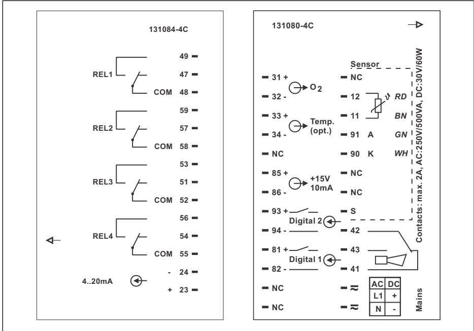
図 4 端子部ステッカー
