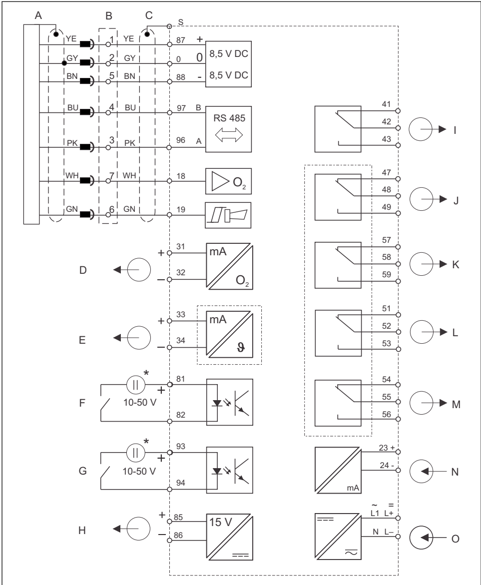
図 6 Liquisys M COM223/253 (WX または WS バージョン) の電気接続
