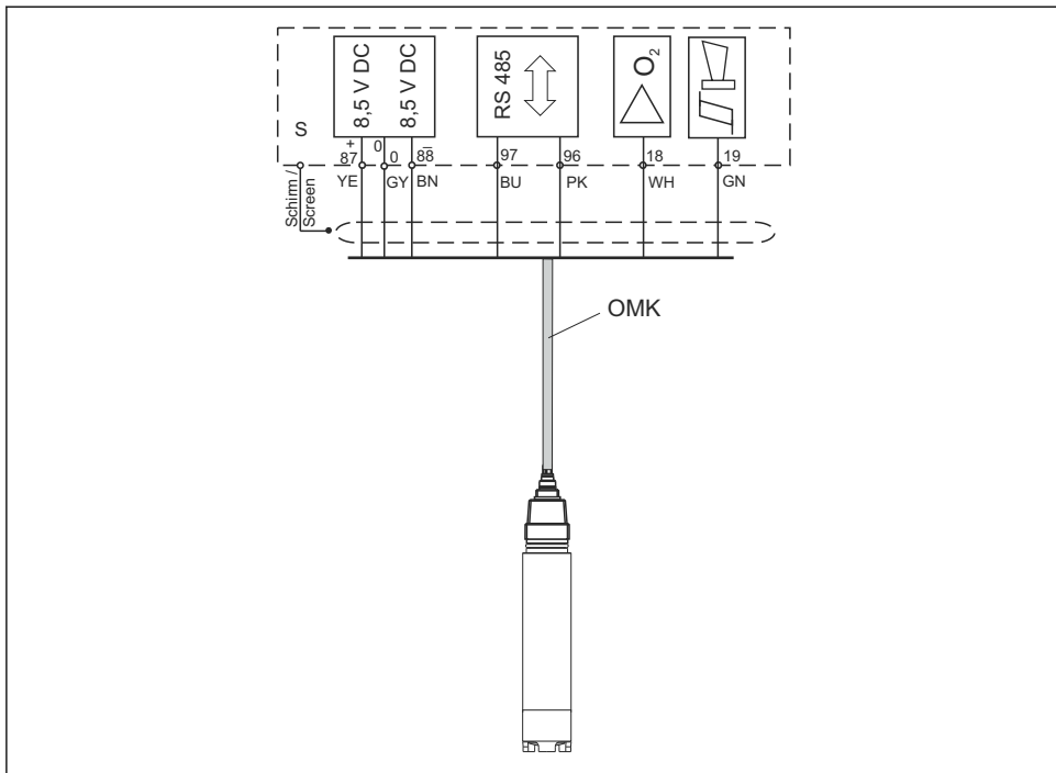
図 9 接続例：COS31/71 および OMK ケーブル
