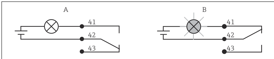
図 10 アラーム接点用の推奨のフェールセーフ切替
