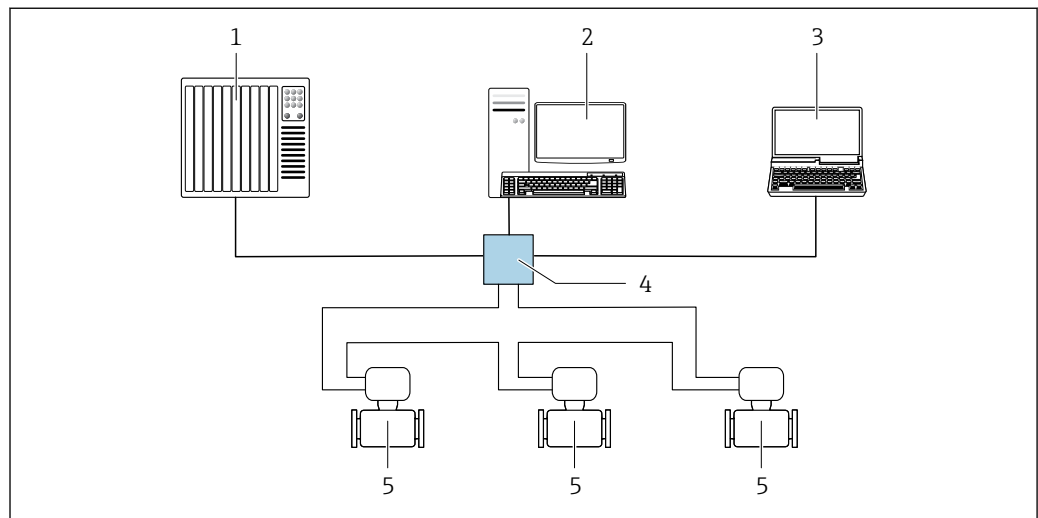
26 Opzioni per funzionamento a distanza mediante rete EtherNet/IP: topologia ad anello
