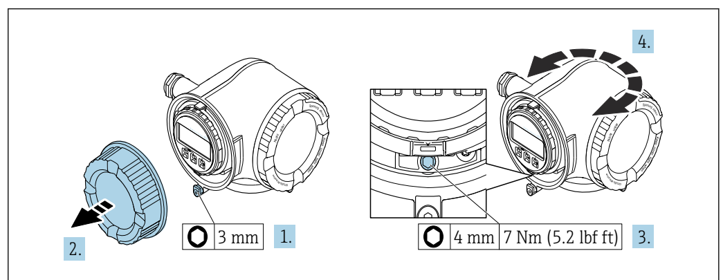
10 Custodia in versione non-Ex
