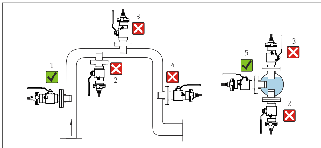
20 Orientations et positions de montage (avec support rétractable CUA451)
