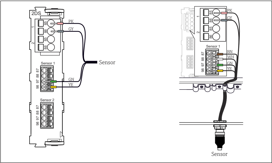
13 Raccordement du capteur à l'entrée capteur (à gauche) ou via connecteur M12 (à droite)
