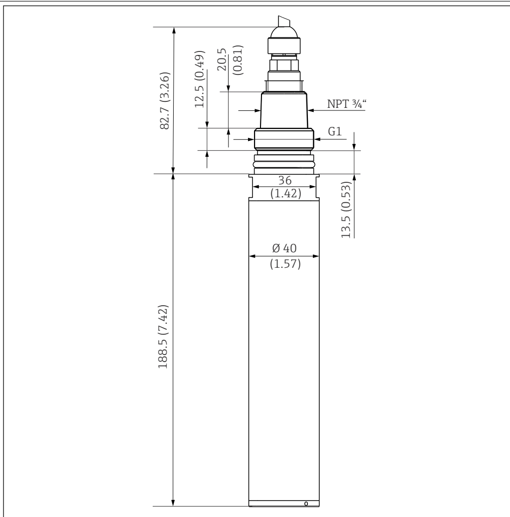
21 Dimensions. Unité de mesure : mm (in)
