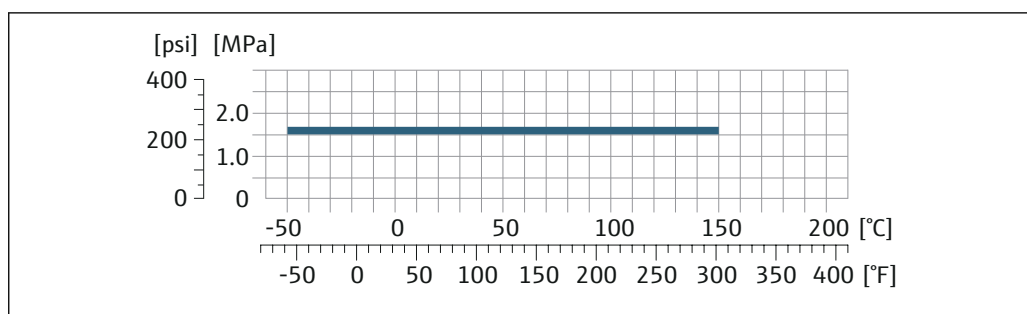
図 27 接続部材質 グレード 2 チタン
