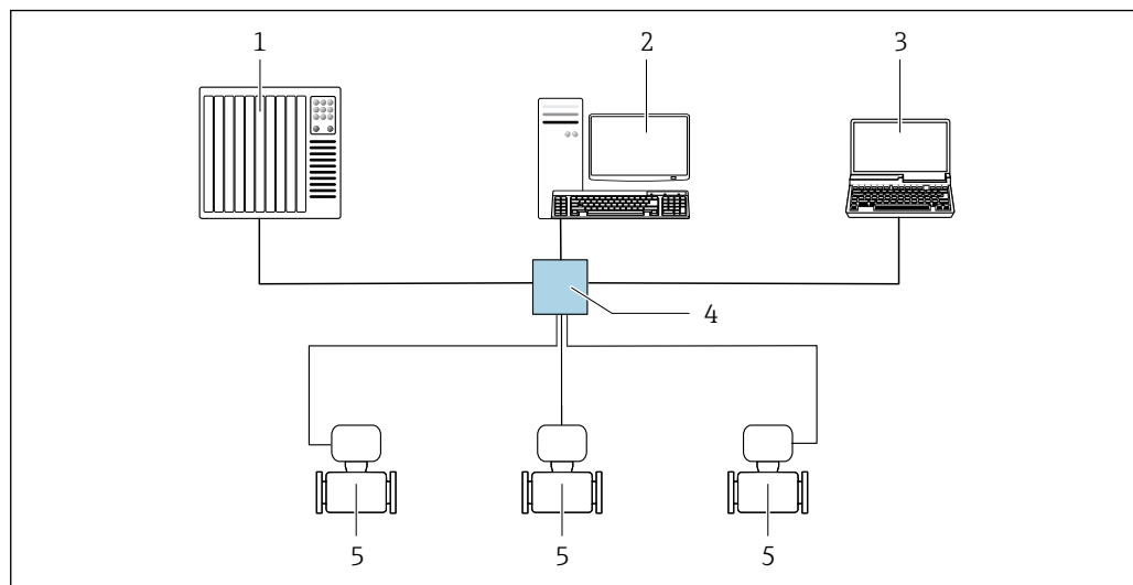
図 56 Modbus TCP over Ethernet - 100 Mbit/s 経由のリモート操作用オプション：スター型トポロジー
