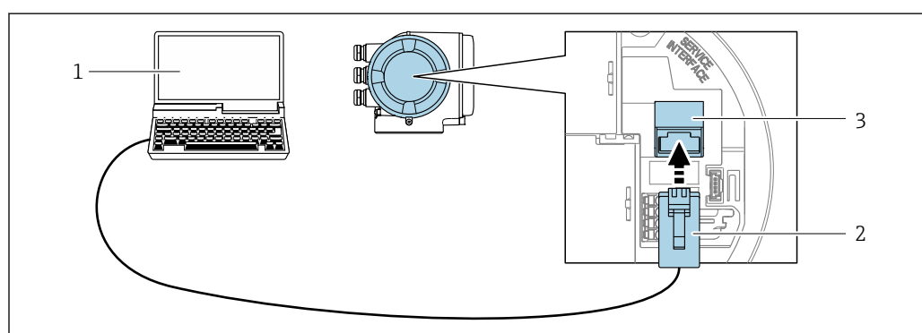
図 58 サービスインタフェース (CDI-RJ45) 経由の接続
