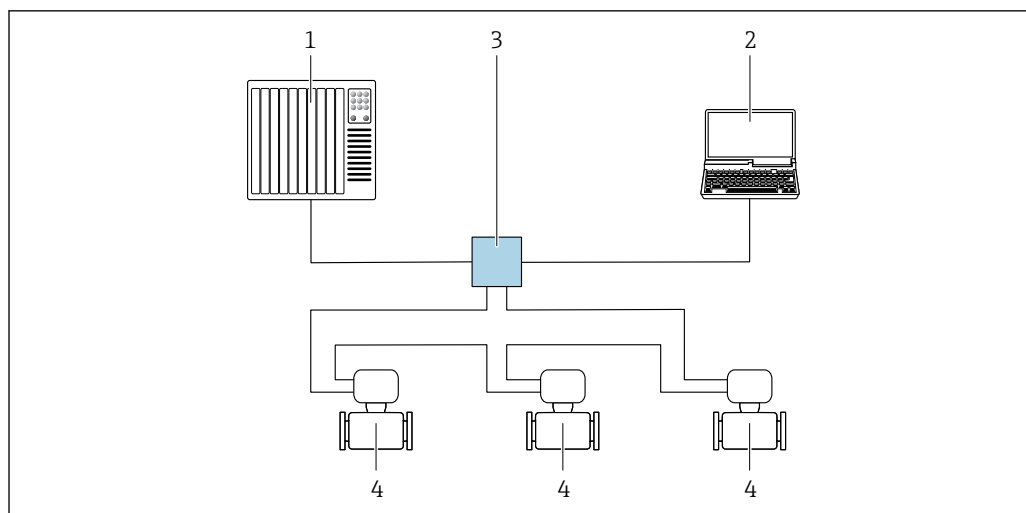
図 54 PROFINET ネットワーク経由のリモート作用オプション：リング型トポロジー
