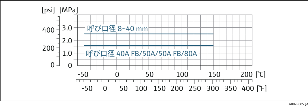
図 24 フランジ材質 グレード 2 チタン
