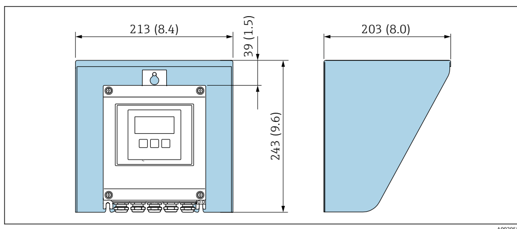
図 37 Proline 500 – デジタル用の日除けカバー、単位 mm (in)
