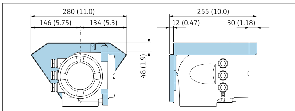
図 38 Proline 500 用の日除けカバー、単位 mm (in)
