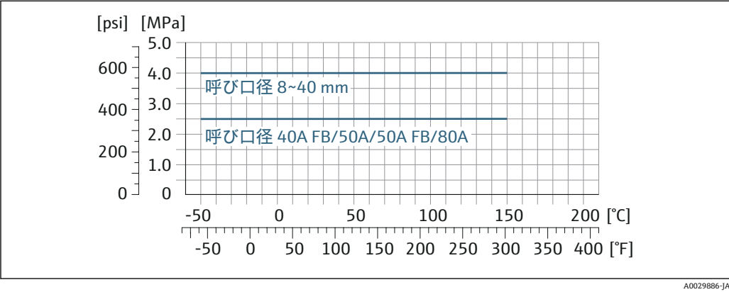
図 25 接続部材質 グレード 2 チタン
