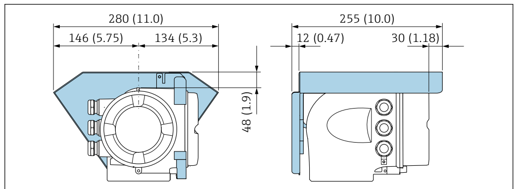
図 19 Proline 500 用の日除けカバー、単位 mm (in)
