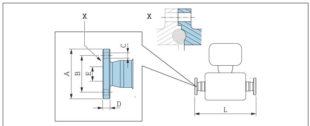
図 30 Xの詳細：非対称型プロセス接続；着色部分が供給されます。
