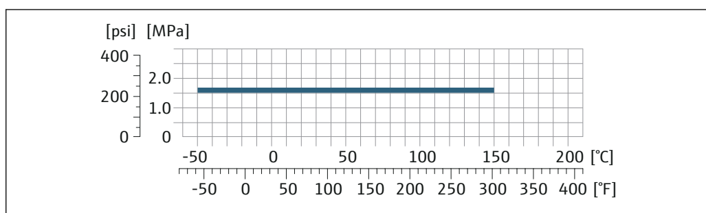
図 28 接続部材質 グレード 2 チタン
