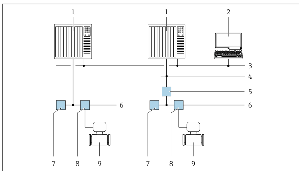
図 47 FOUNDATION Fieldbus ネットワークを介したリモート操作用のオプション
