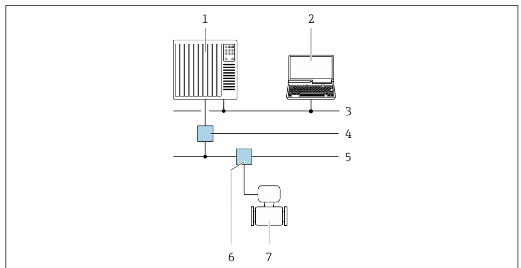
図 49 PROFIBUS PA ネットワークを介したリモート操作のオプション
