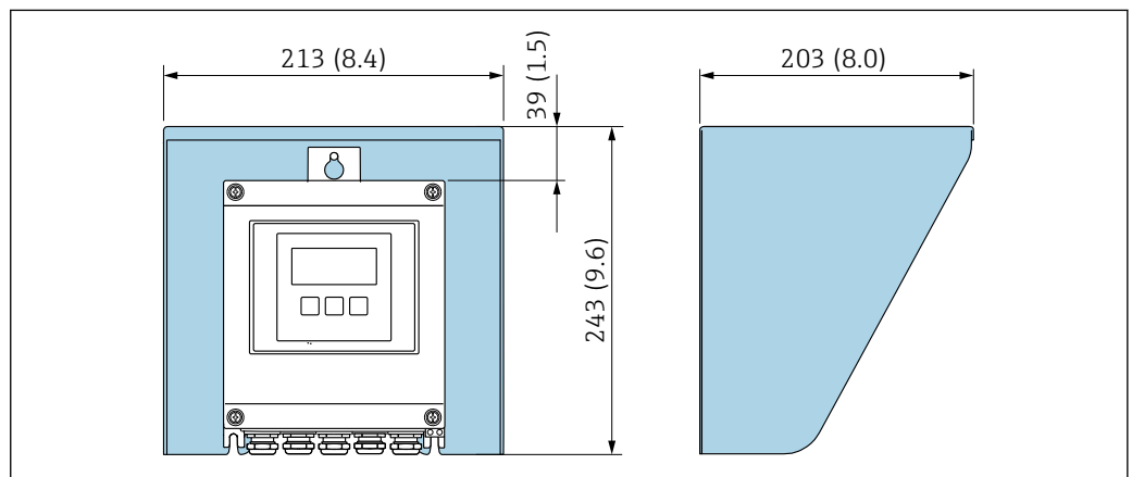
図 18 Proline 500 – デジタル用の日除けカバー、単位 mm (in)
