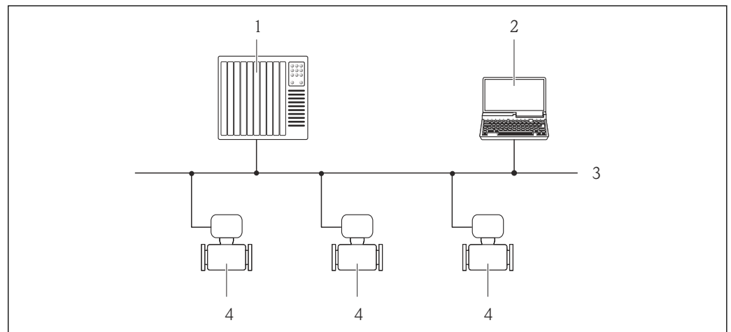
図 48 PROFIBUS DP ネットワークを介したリモート操作のオプション
