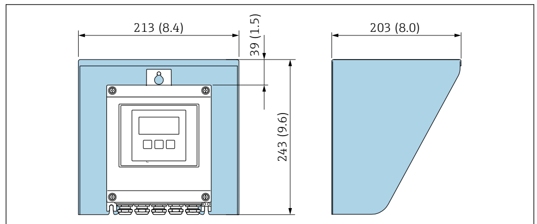
31 Proline 500 – デジタル用の日除けカバー、単位 mm (in)
