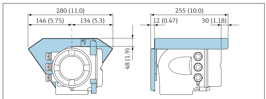
32 Proline 500 用の日除けカバー、単位 mm (in)
