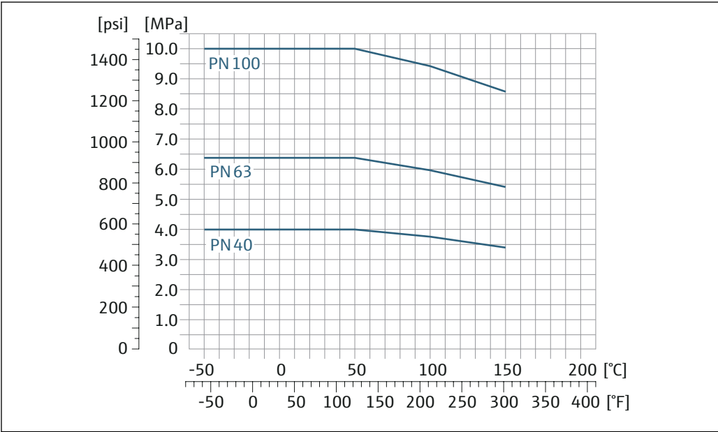
21 フランジ材質 1.4301 (SUS 304 相当) ; 接液部 : チタン
