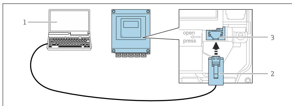
図 57 サービスインタフェース (CDI-RJ45) 経由の接続
