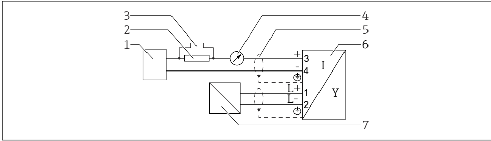
図 15 ブロック図、4 線式：4～20 mA HART（10.4～48 V DC ）
