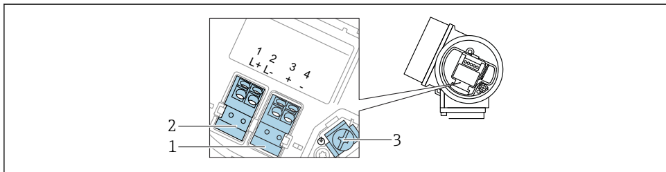
図 14 端子の割当て、4 線式：4～20 mA HART（10.4～48 V DC ）
