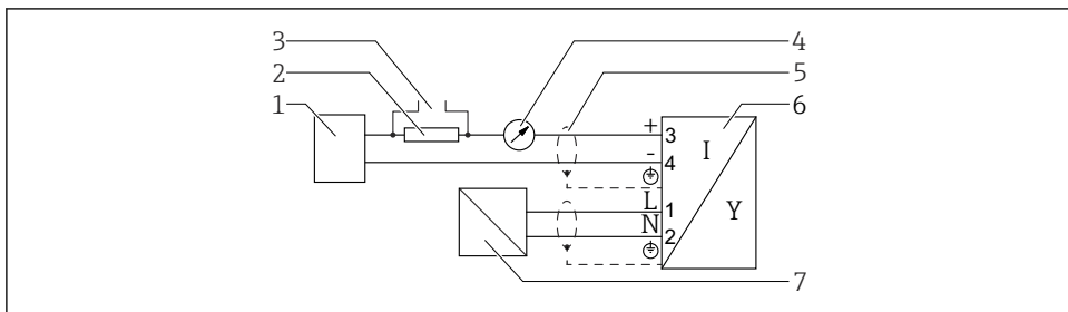
図 17 ブロック図、4 線式：4～20 mA HART (90～253 V AC )
