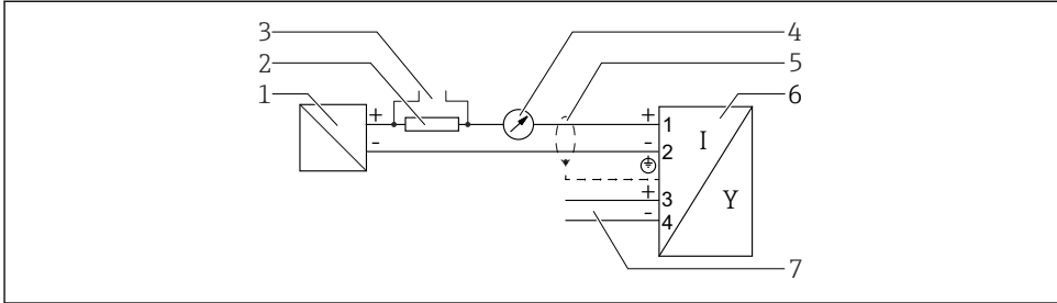
図 11 ブロック図、2 線式：4～20 mA HART、スイッチ出力
