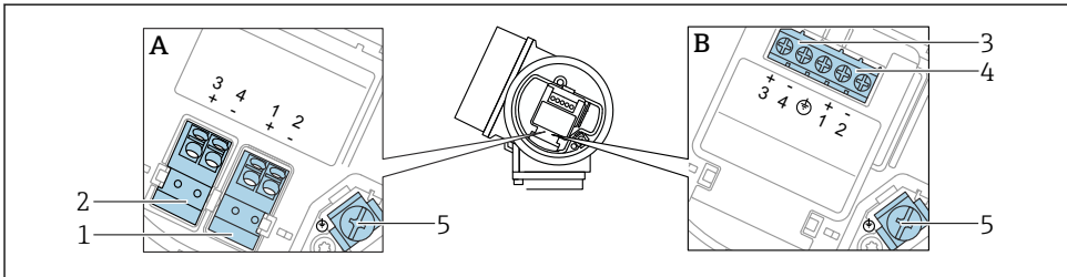
図 12 端子の割当て、2 線式：4～20 mA HART、4～20 mA
