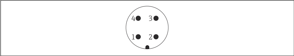
図 18 M12 プラグのピン割当て
