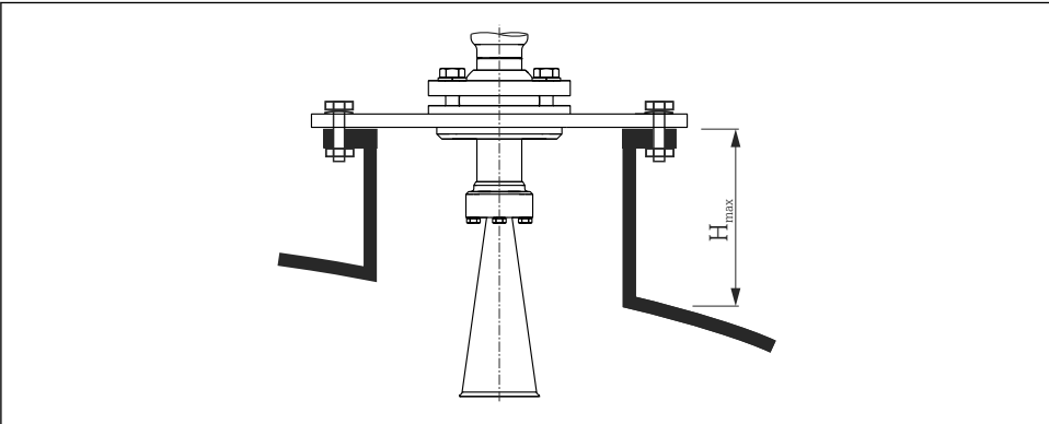
図 4 ホーンアンテナのノズル高 (FMR57)
