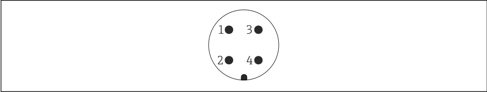
図 19 7/8" プラグのピン割当て
