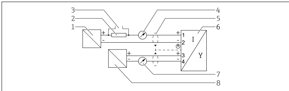
図 13 ブロック図、2 線式：4～20 mA HART、4～20 mA
