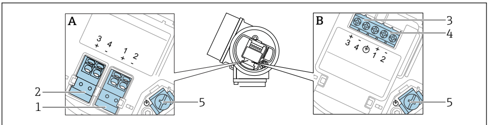
図 10 端子の割当て、2 線式：4～20 mA HART、スイッチ出力
