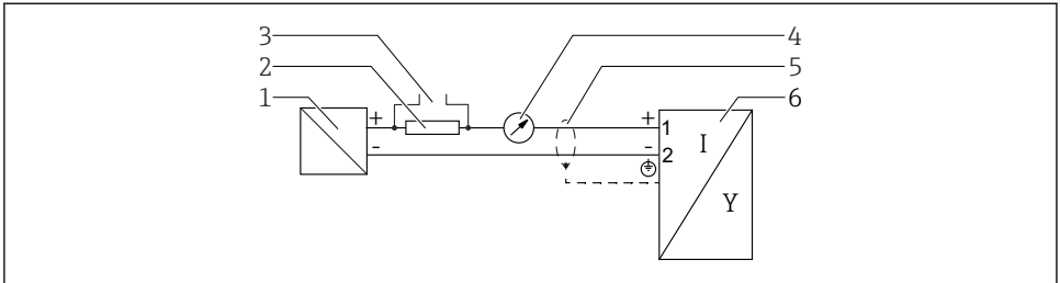
図 9 ブロック図、2 線式：4～20 mA HART
