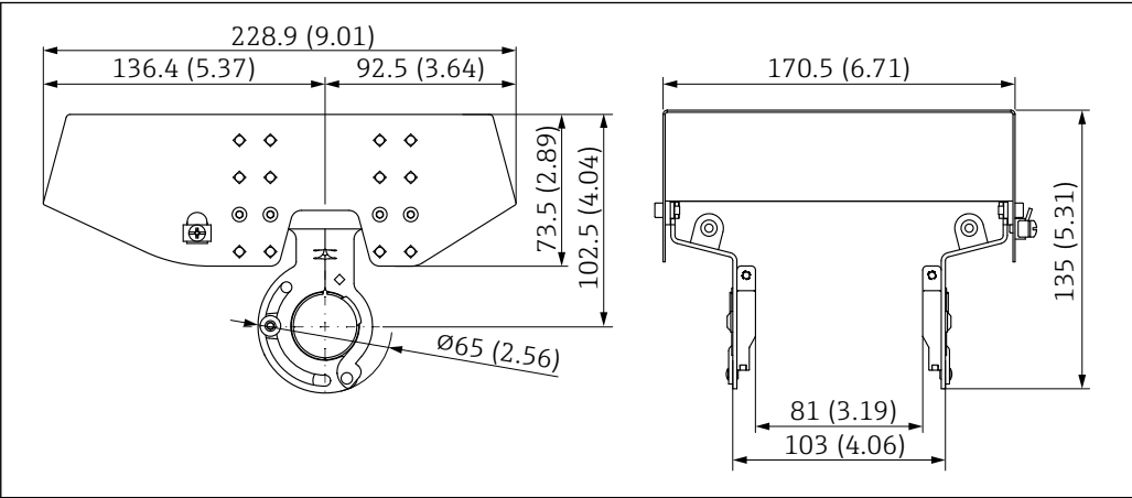
30 防护罩，适用双腔体外壳。测量单位 mm (in)
