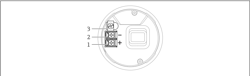
图 18 接线腔内的接线端子和接地端，单腔室外壳
