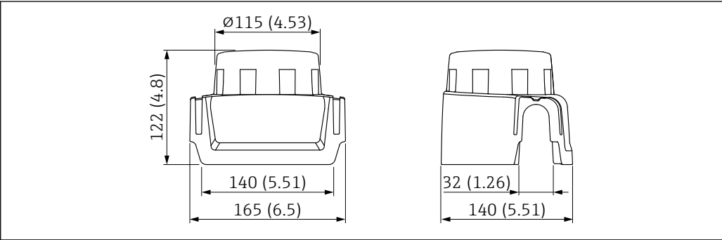
31 防护罩，适用单腔体铝外壳。测量单位 mm (in)
