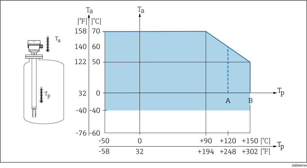
图 33 外壳允许环境温度 T_a 与罐体内部过程温度 T_p 的关系
