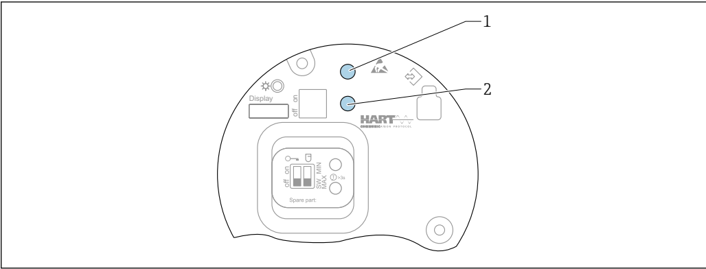
图 29 FEL60H 电子插件上的操作按键
