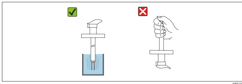
图 25 音叉的功能测试
