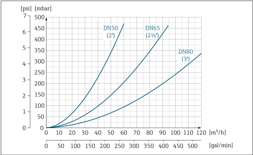
32 Perte de charge DN 50 à 80 (2 to 3") pour caractéristique de commande "Construction", option C "Bride fixe, tube de mesure rétréci", sections d'entrée/de sortie 0 x DN"
