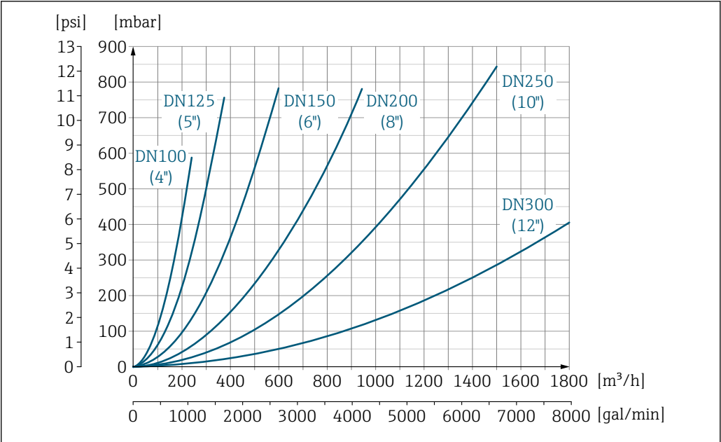
33 Perte de charge DN 100 à 300 (4 to 12") pour caractéristique de commande "Construction", option C "Bride fixe, tube de mesure rétréci", sections d'entrée/de sortie 0 x DN"
