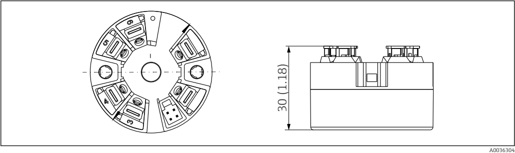
7 Versão com terminais push-in. Dimensões são idênticas à versão com terminais de parafuso, com exceção da altura do invólucro.
