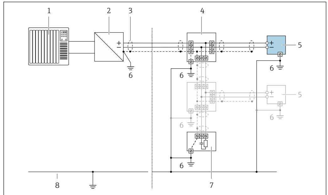
Fig. 17 Ejemplo de conexión para PROFIBUS PA
