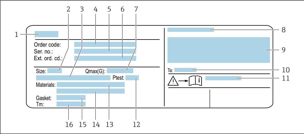
图 4 传感器的铭牌示意图
