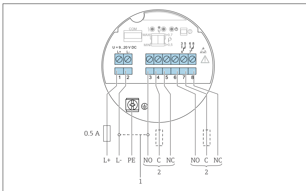
24 Collegamento c.c. con uscita a relè, inserto elettronico FEL64 DC
