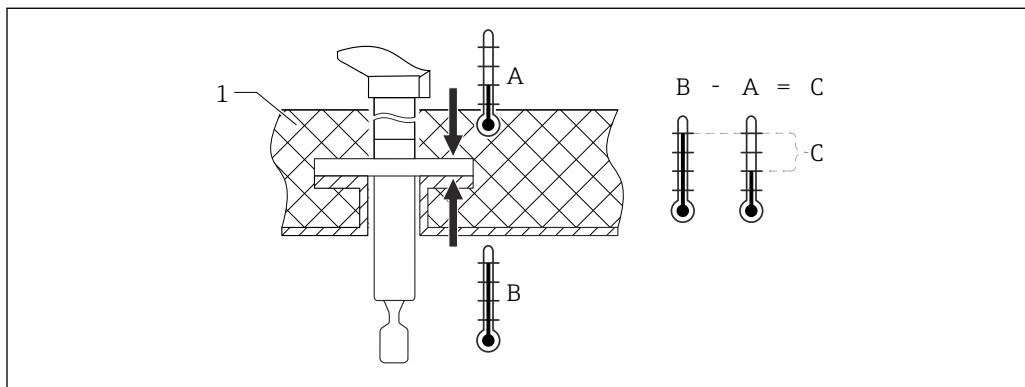
4 Differenza di temperatura tra lato esterno e interno della flangia
