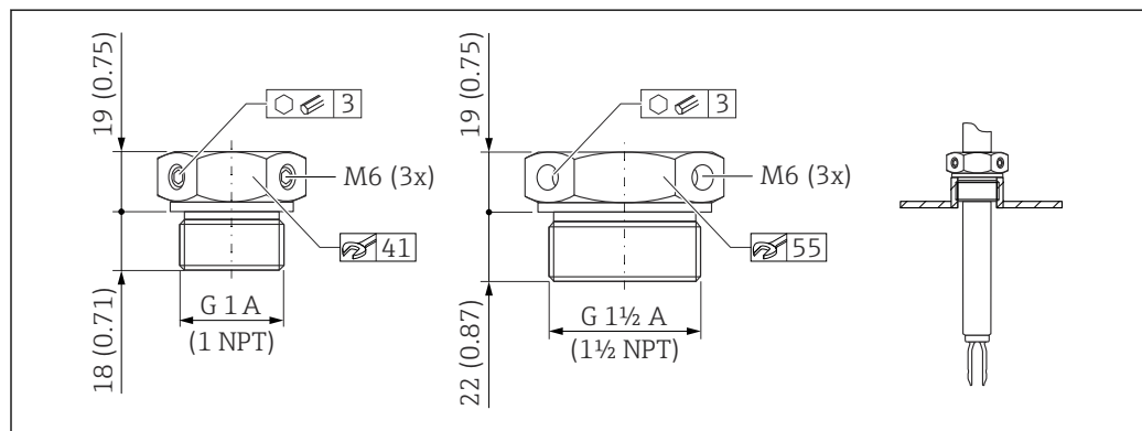
49 Manicotti scorrevoli per il funzionamento non pressurizzato p_e = 0 bar (0 psi). Unità di misura mm (in)
