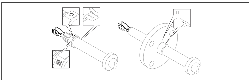
11 Posizione del rebbo vibrante installato orizzontalmente nel silo utilizzando la marcatura
