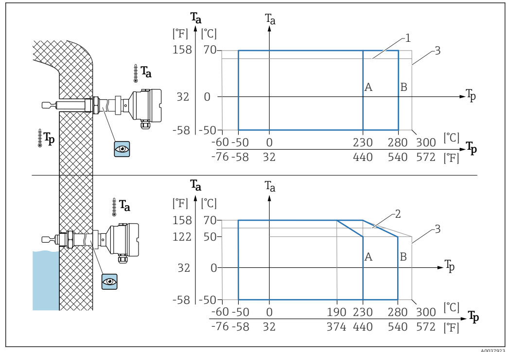
51 Temperatura ambiente T_a consentita sulla custodia in base alla temperatura di processo T_p presente nel recipiente
