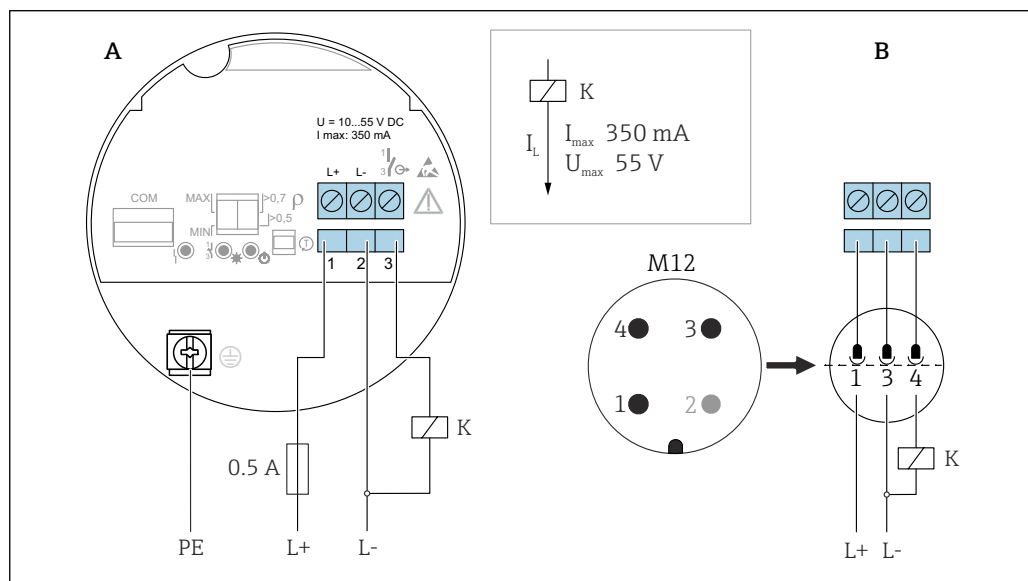
20 PNP c.c. trifilare, inserto elettronico FEL62
