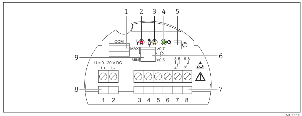
33 Esempio di inserto elettronico FEL64DC
