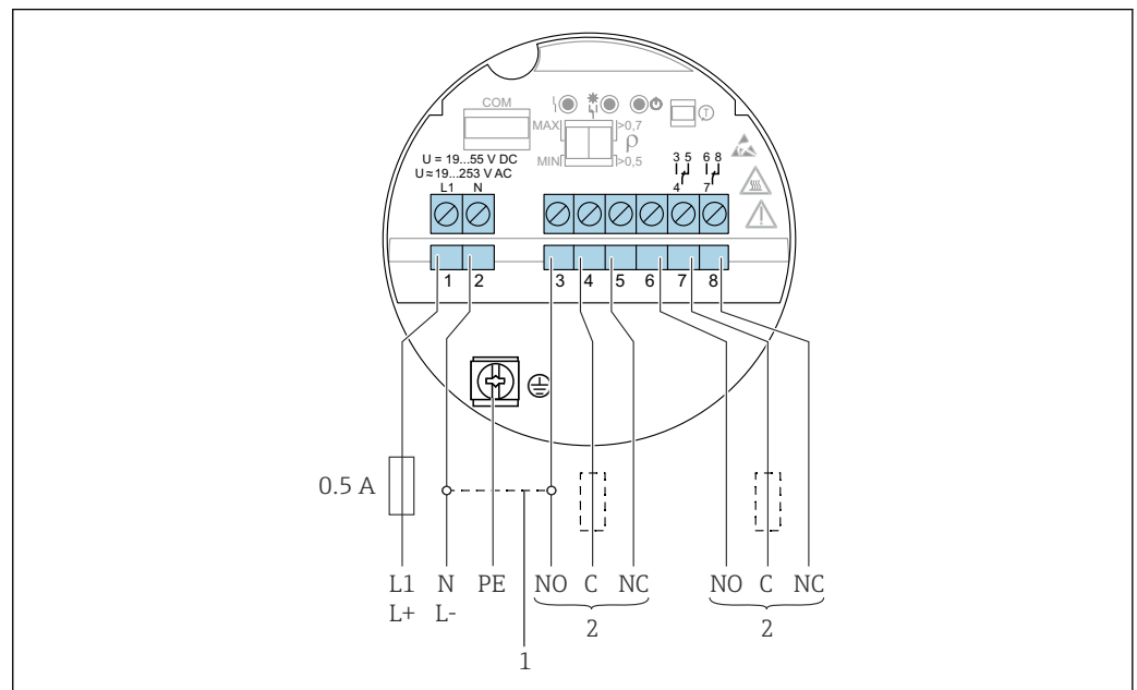
22 Connessione di corrente universale con uscita a relè, inserto elettronico FEL64
