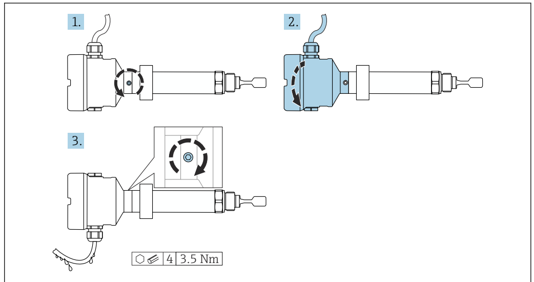
15 Custodia con vite di bloccaggio esterna; formare un anello salvagoccia sul cavo
